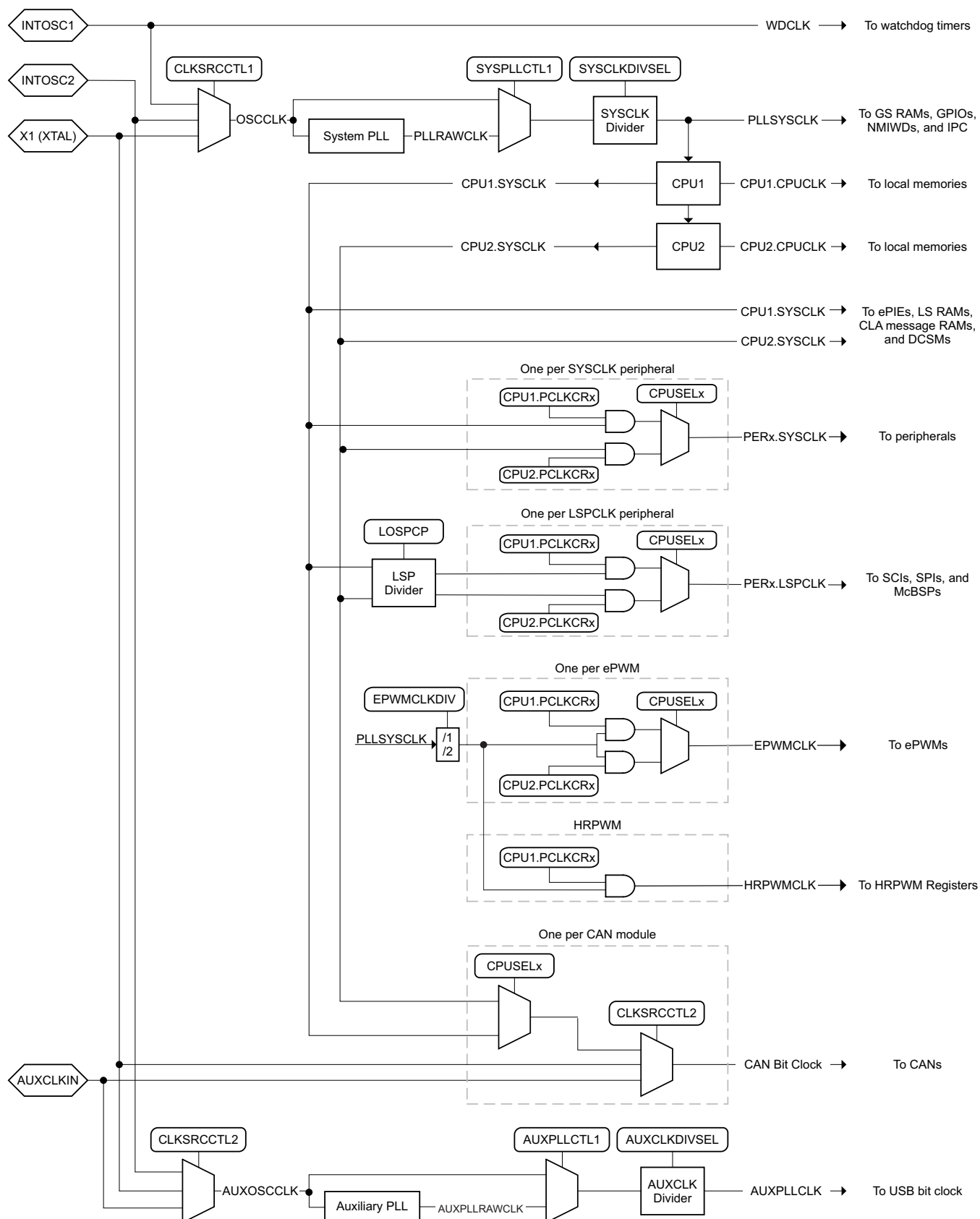
图 4-8. Clocking System
