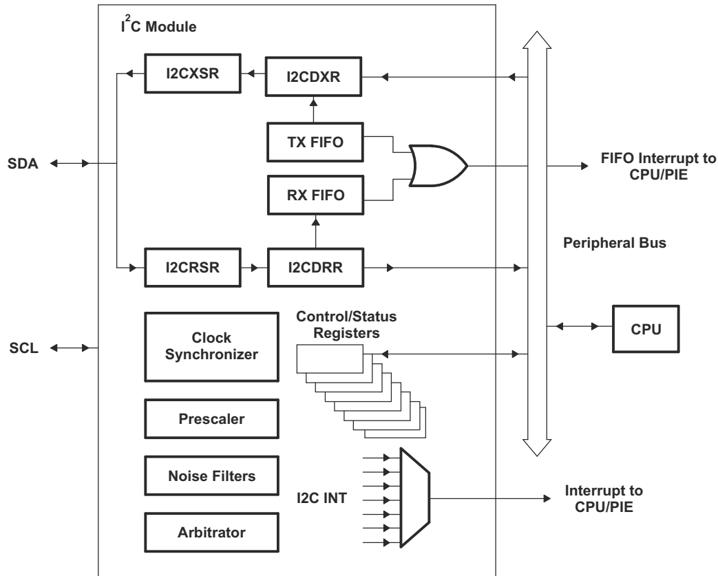
图 6-62. I 2 C 外设模块接口
