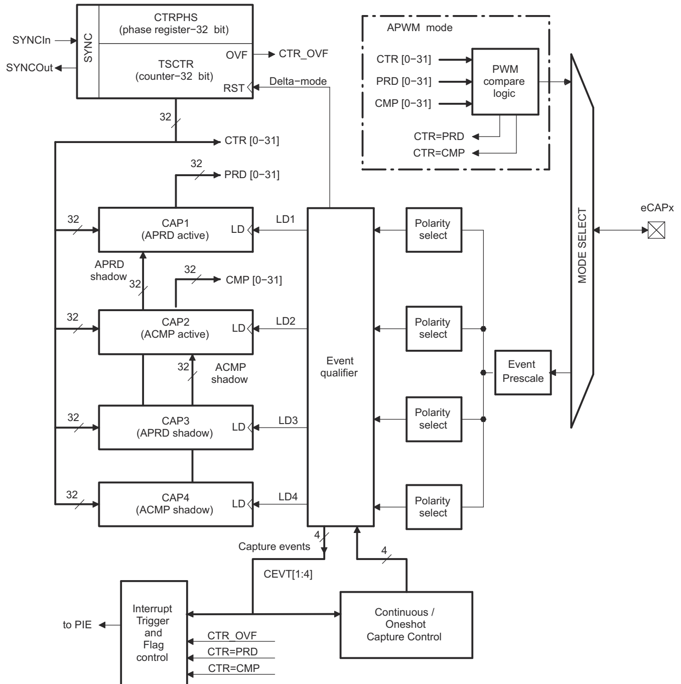
图 6-49. eCAP 方框图
