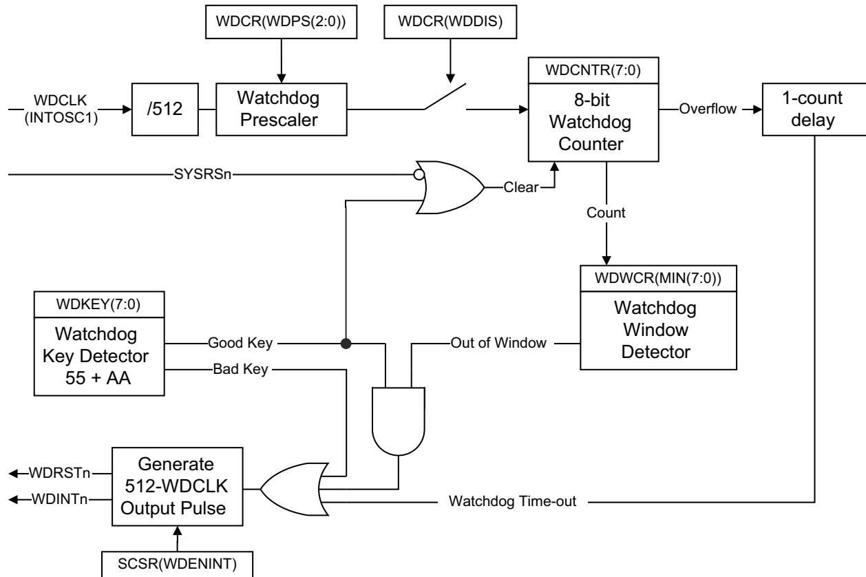
图 7-4. 窗口看门狗
