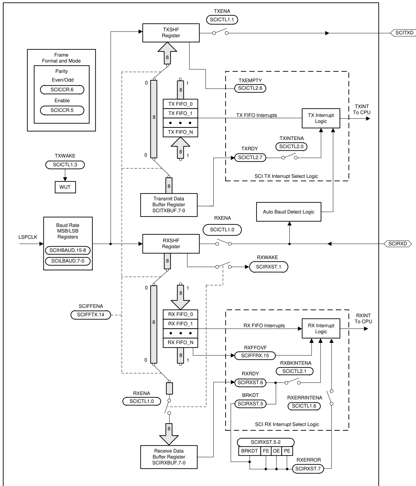
图 6-71. SCI 方框图
