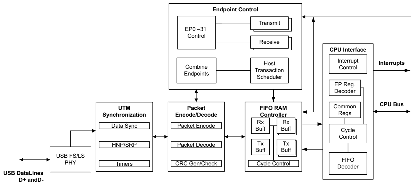
图 6-77. USB 方框图
