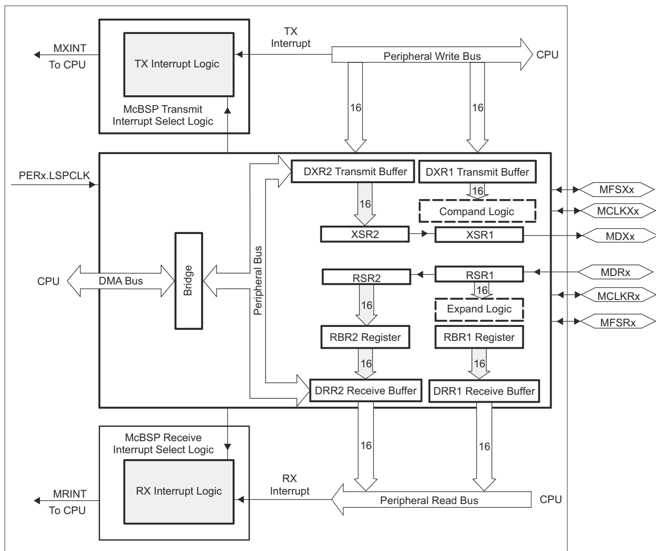
图 6-64. McBSP 方框图
