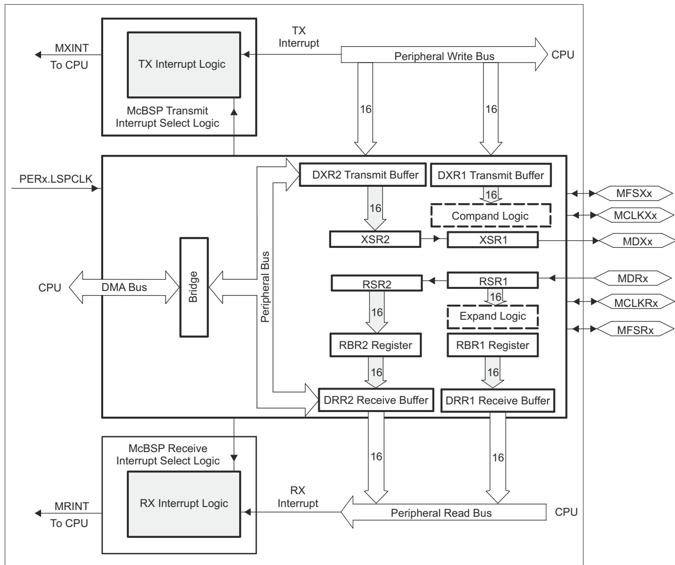
图 6-64. McBSP 方框图
