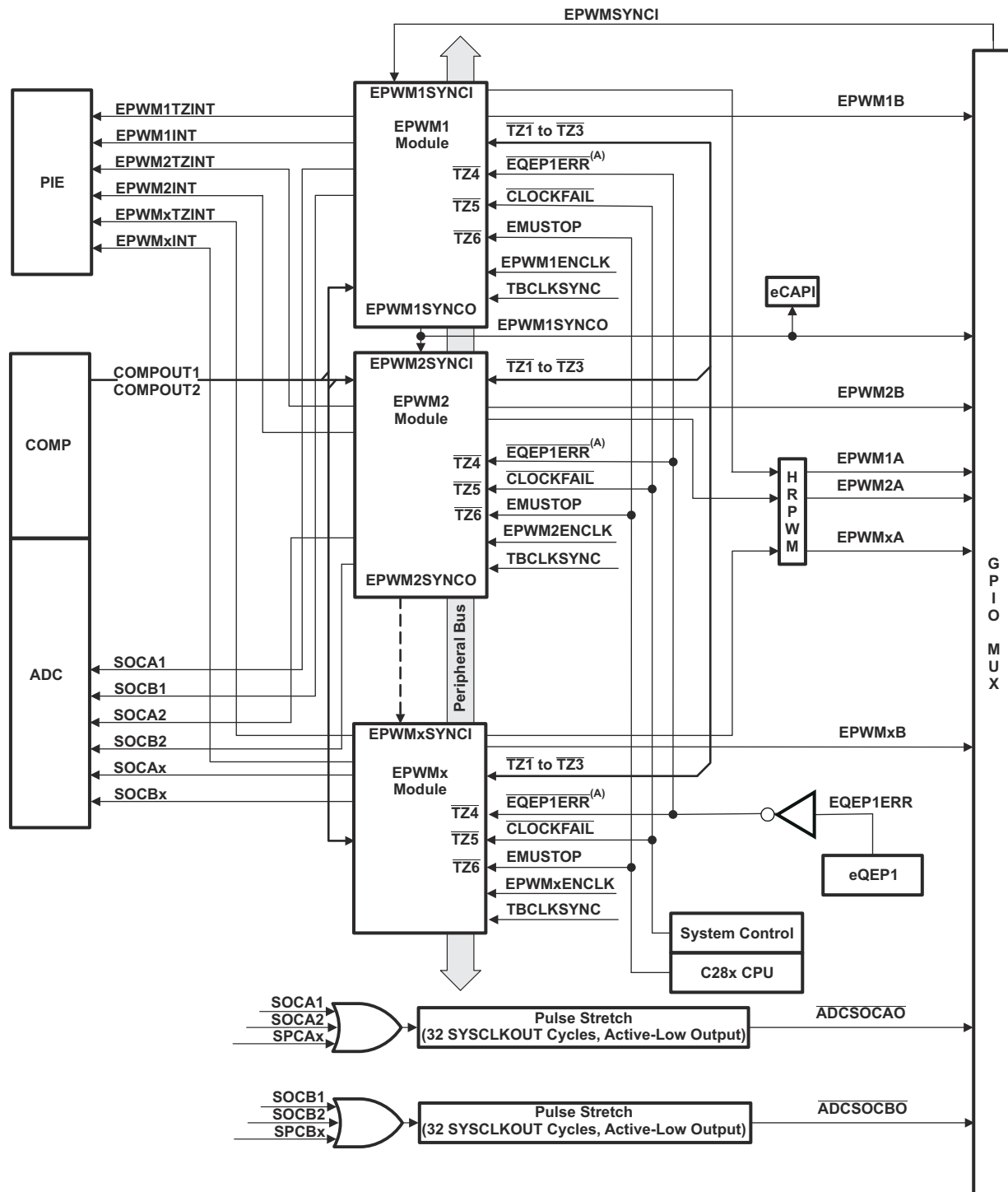
图 8-48. ePWM
