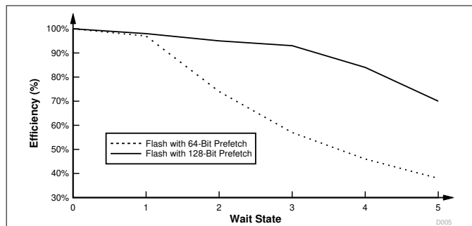
图 6-24. 具有大量 32 位浮点数学指令的应用程序代码
