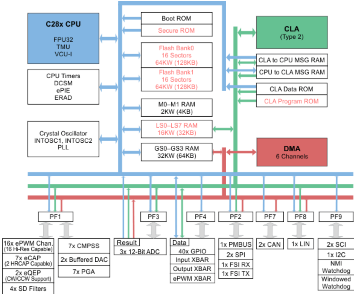
图 7-1. 功能方框图
