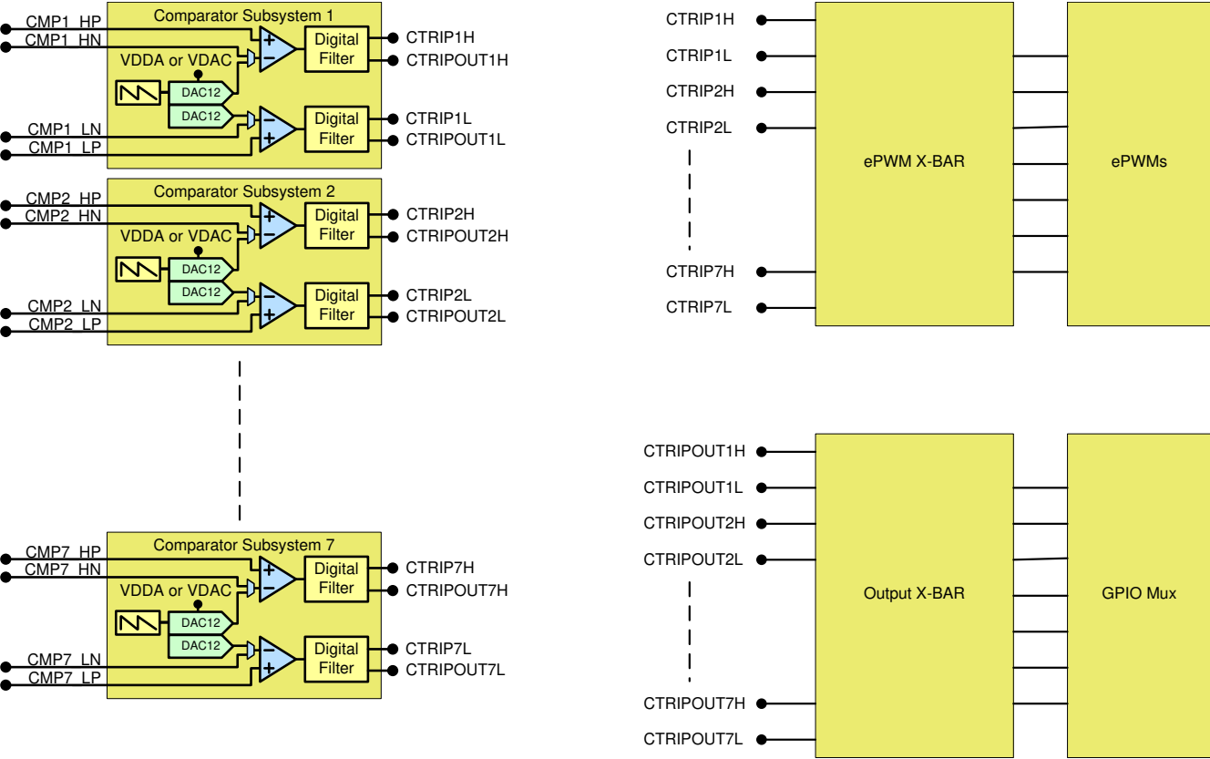
图 6-57. CMPSS 连接
