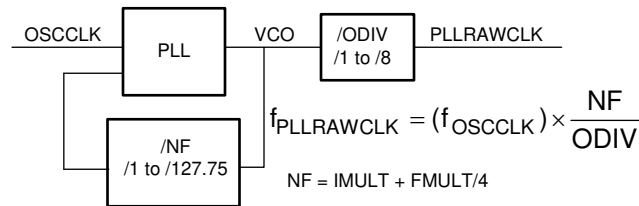
图 6-16. 系统 PLL
