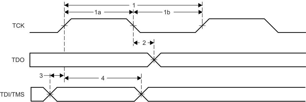
图 6-28. JTAG 时序
