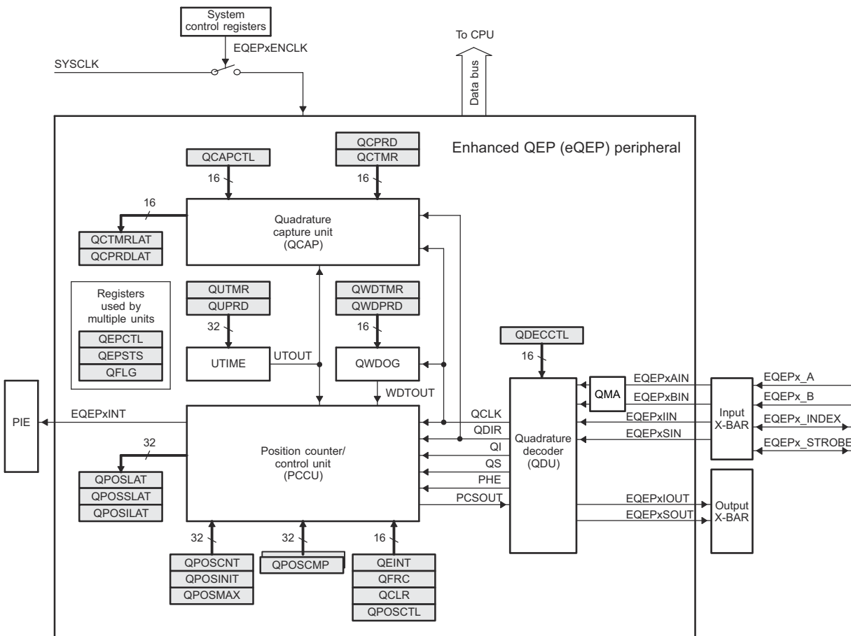
图 6-72. eQEP 方框图
