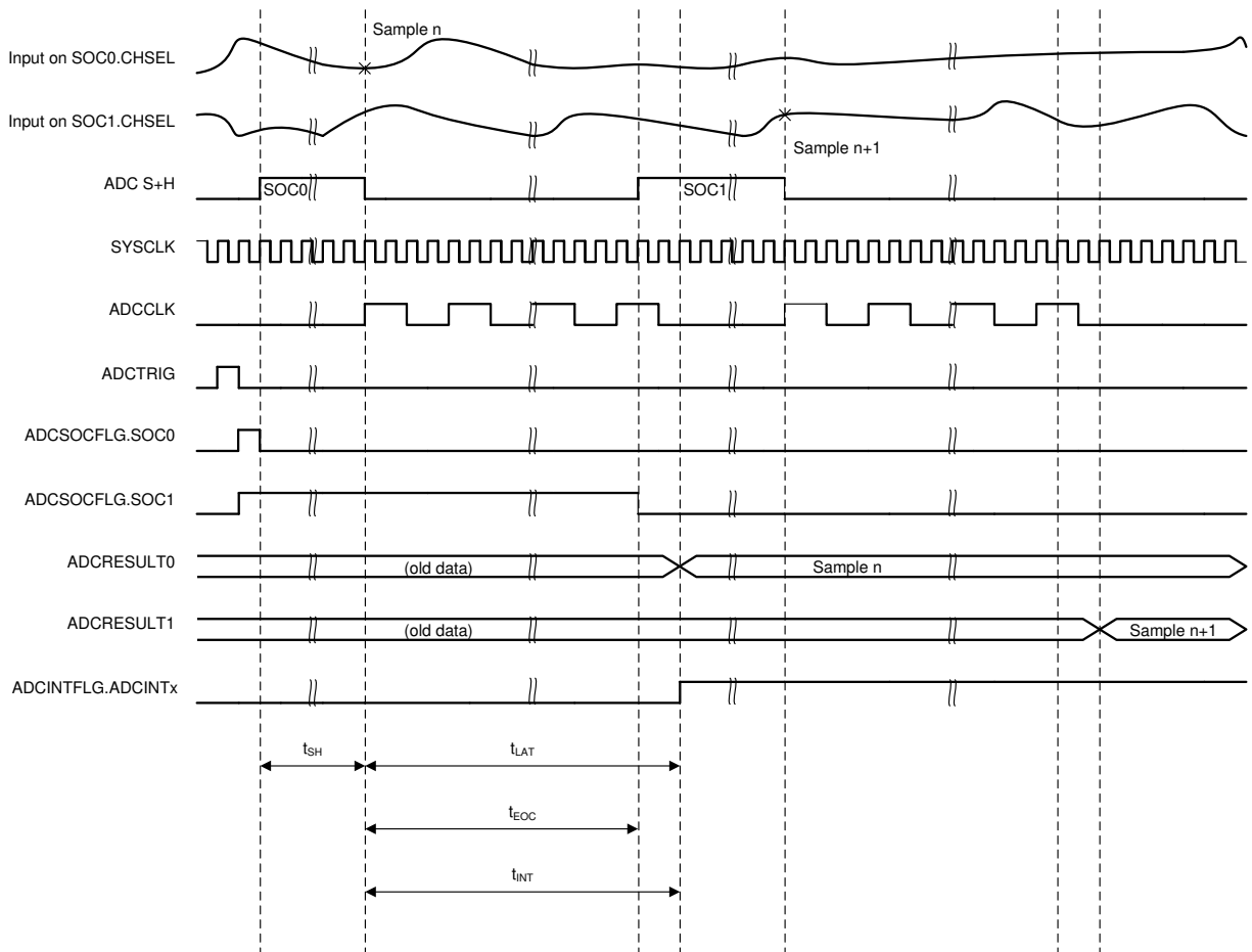
图 6-44. ADC 时序
