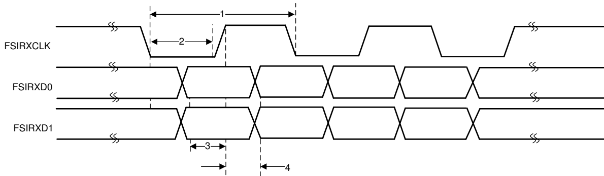
图 6-98. FSIRX 时序
