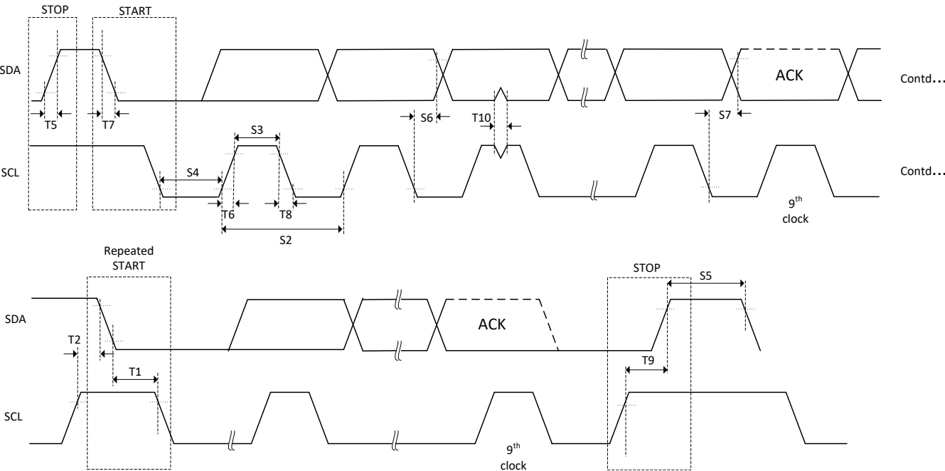
图 6-80. I2C 时序图
