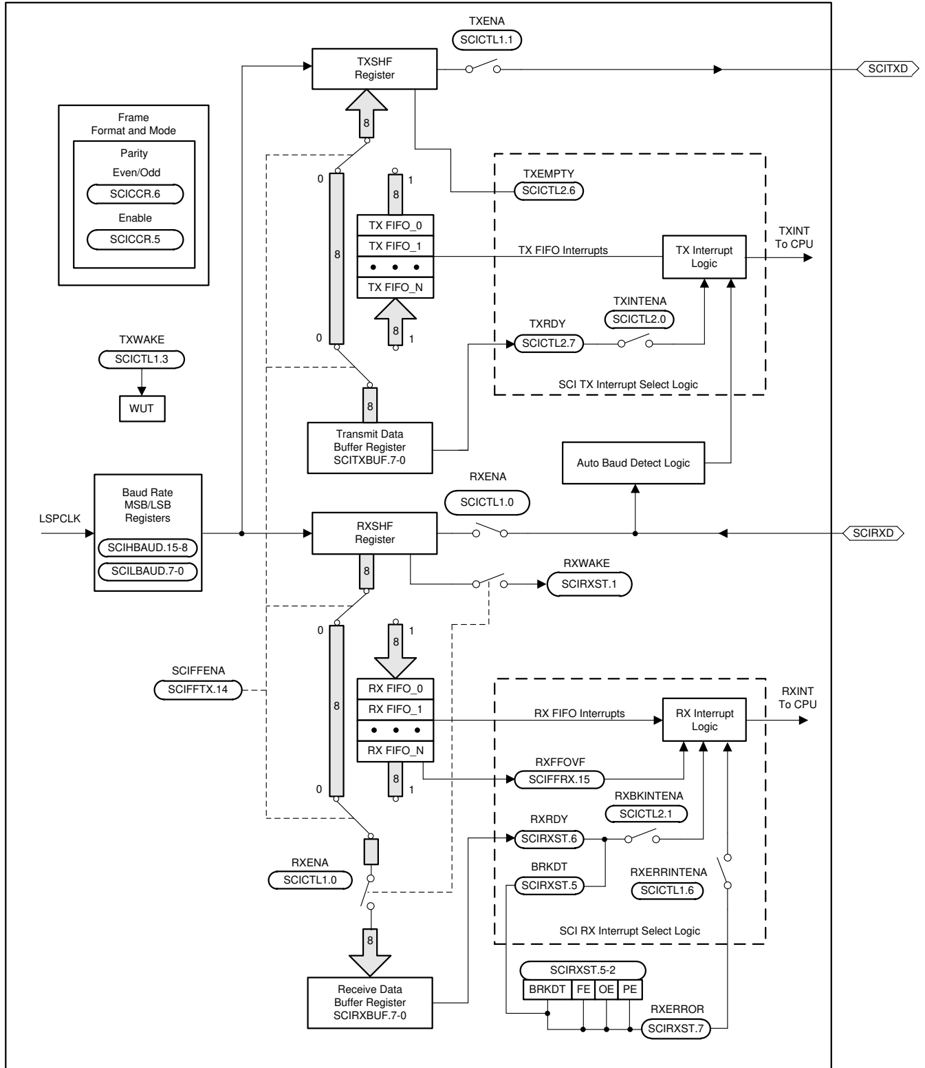
图 6-82. SCI 方框图
