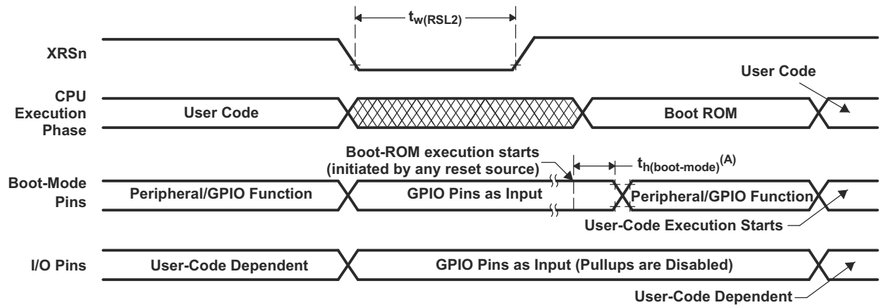
图 6-13. 上电复位
