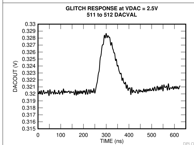
图 6-53. 毛刺脉冲响应 - 511 至 512 DACVAL
