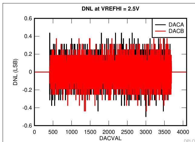
图 6-51. DNL
