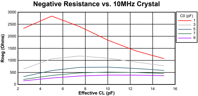
图 6-22. 10MHz 时的负电阻变化
