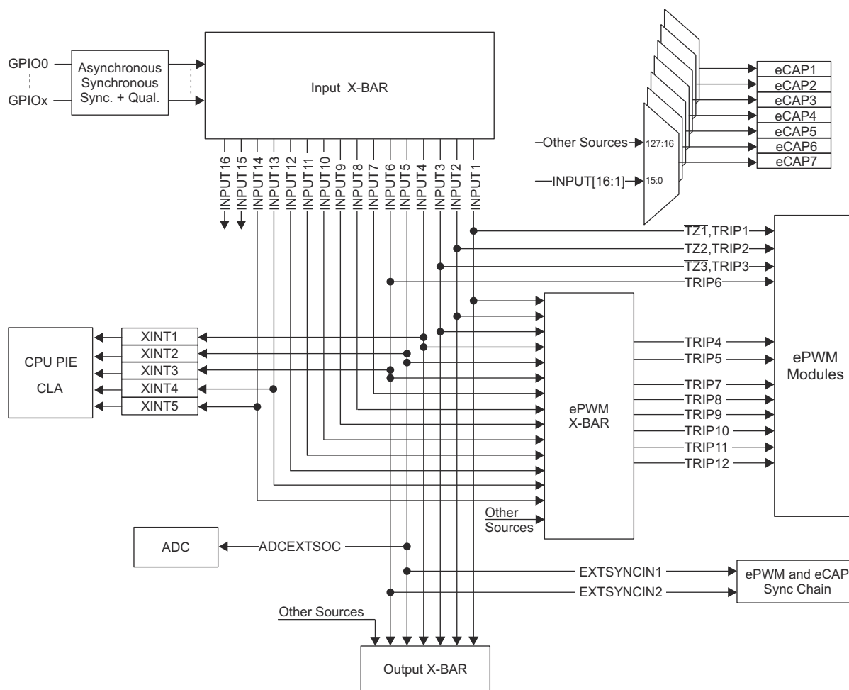
图 5-5. 输入 X-BAR
