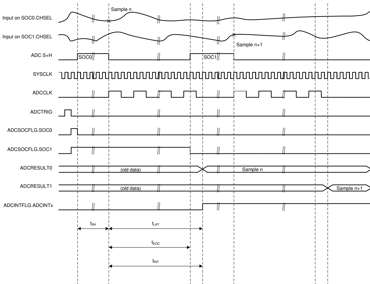
图 6-44. ADC 时序
