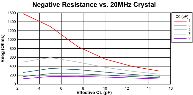
图 6-23. 20MHz 时的负电阻变化
