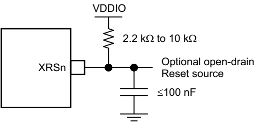
图 6-12. 复位电路
