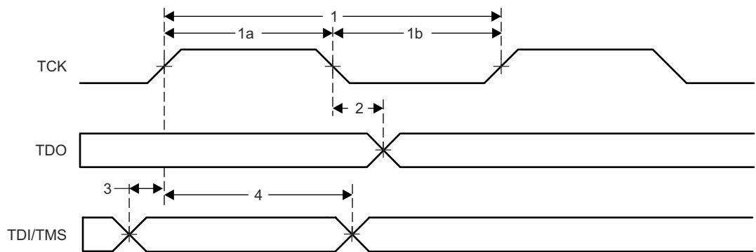
图 6-28. JTAG 时序
