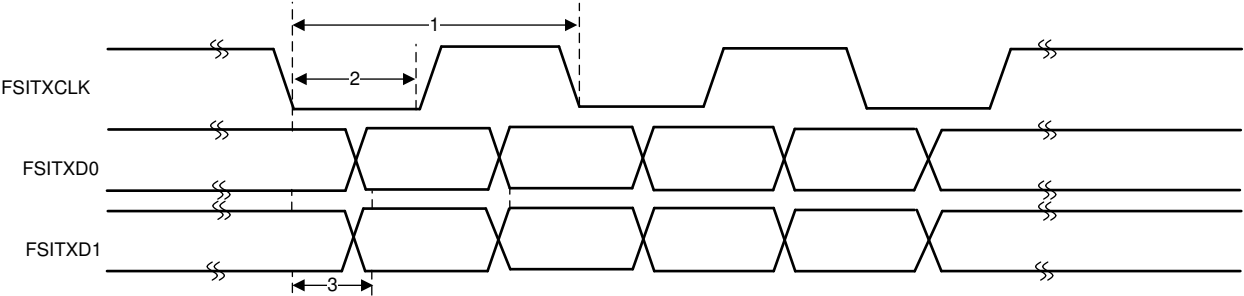
图 6-95. FSITX 时序
