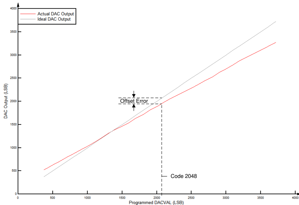
图 6-48. 缓冲 DAC 偏移
