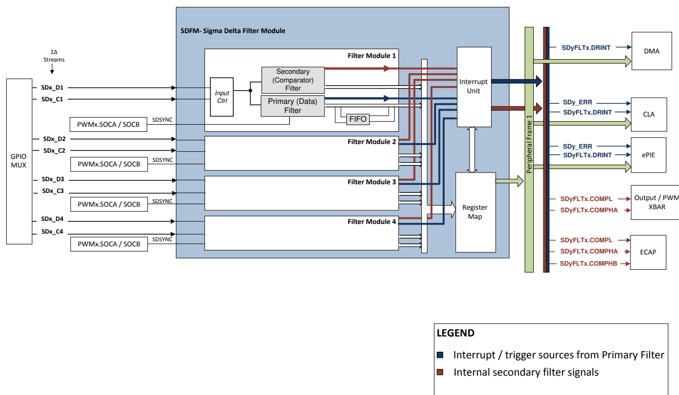
图 6-73. SDFM 方框图
