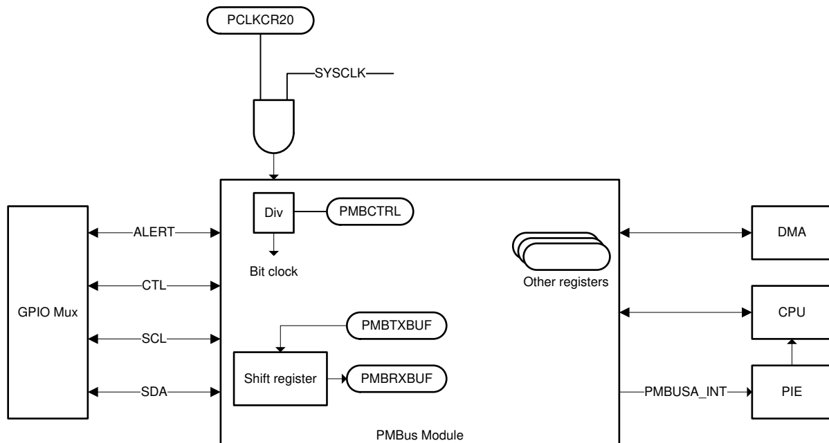
图 6-81. PMBus 方框图
