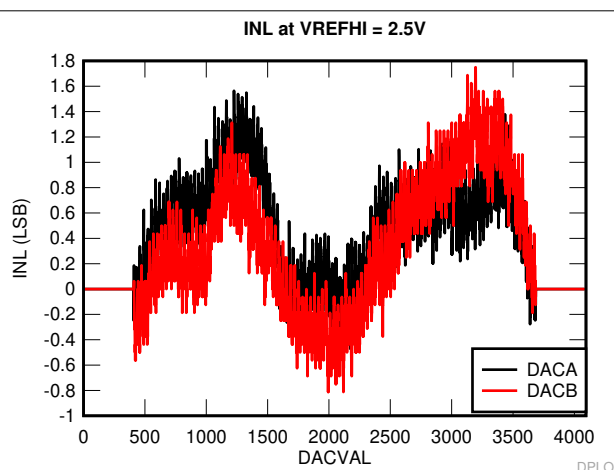
图 6-52. INL
