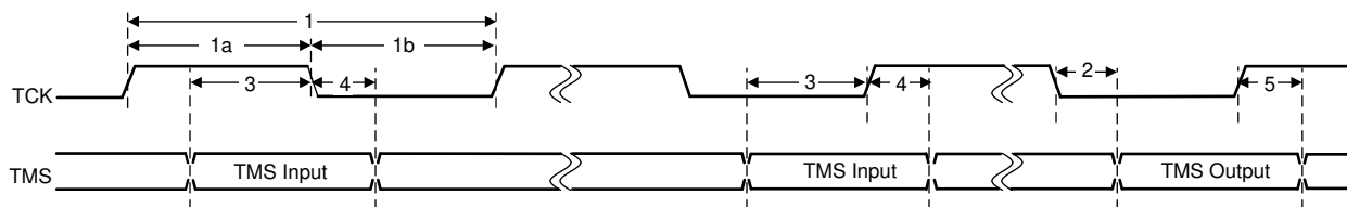
图 6-29. cJTAG 时序
