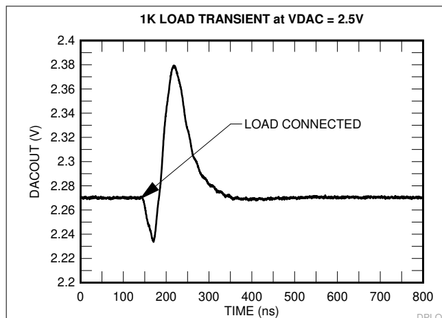
图 6-55. 1k \Omega 负载瞬态
