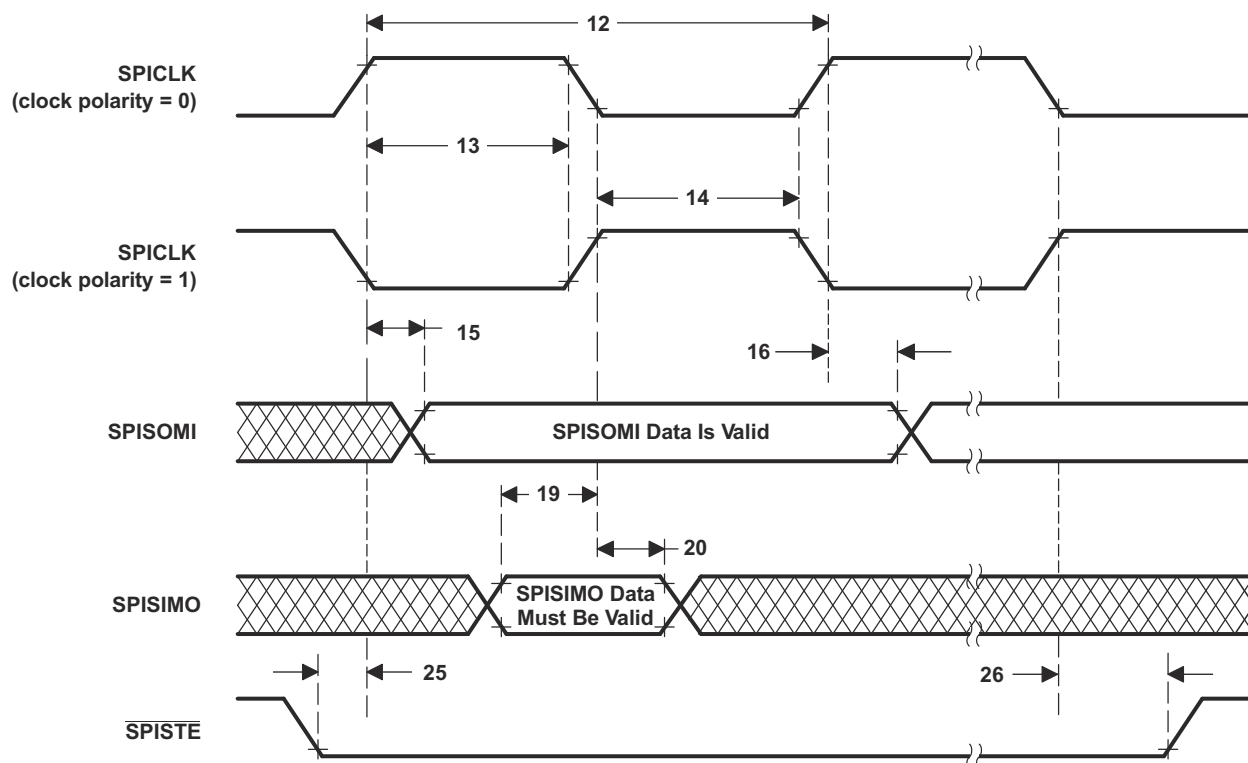
图 6-90. 高速 SPI 从模式外部时序 (时钟相位 = 0)
