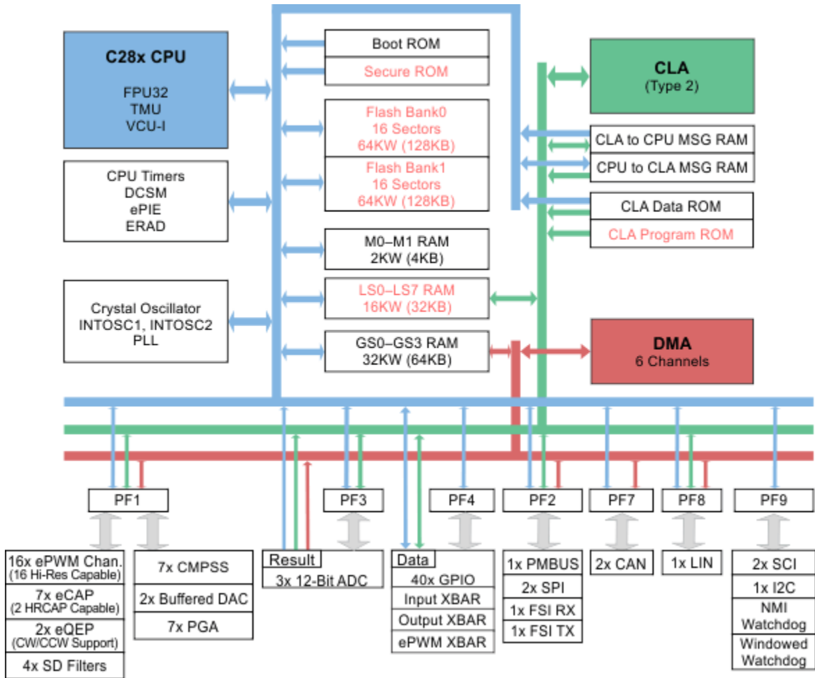
图 7-1. 功能方框图
