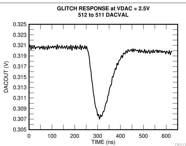
图 6-54. 毛刺脉冲响应 - 512 至 511 DACVAL
