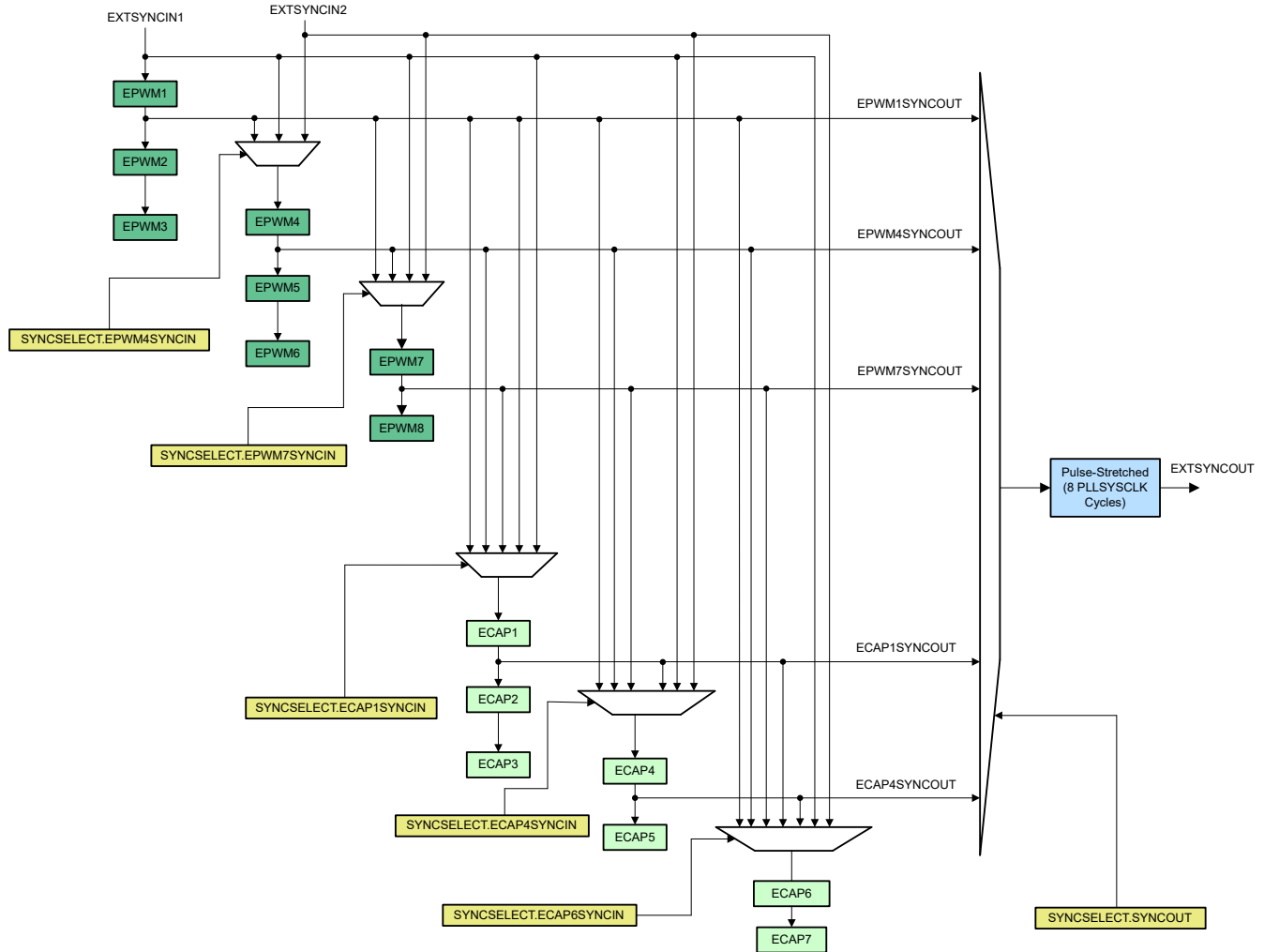
图 6-69. 同步链架构
