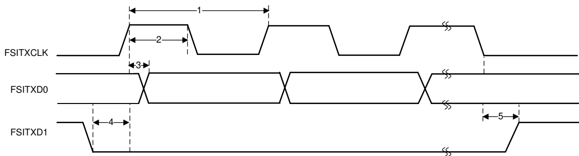
图 6-99. FSITX SPI 信令模式时序
