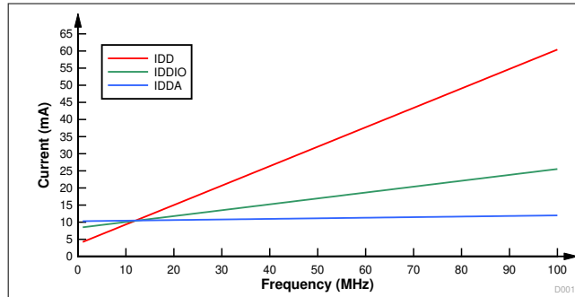
图 6-2. 电流与频率间的关系 - 外部电源
