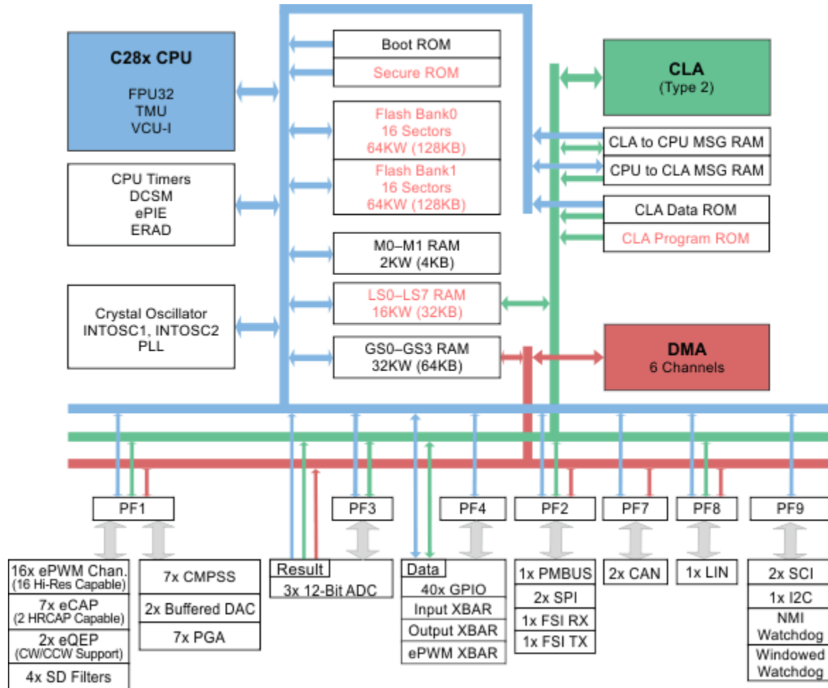
图 3-1. 功能方框图
