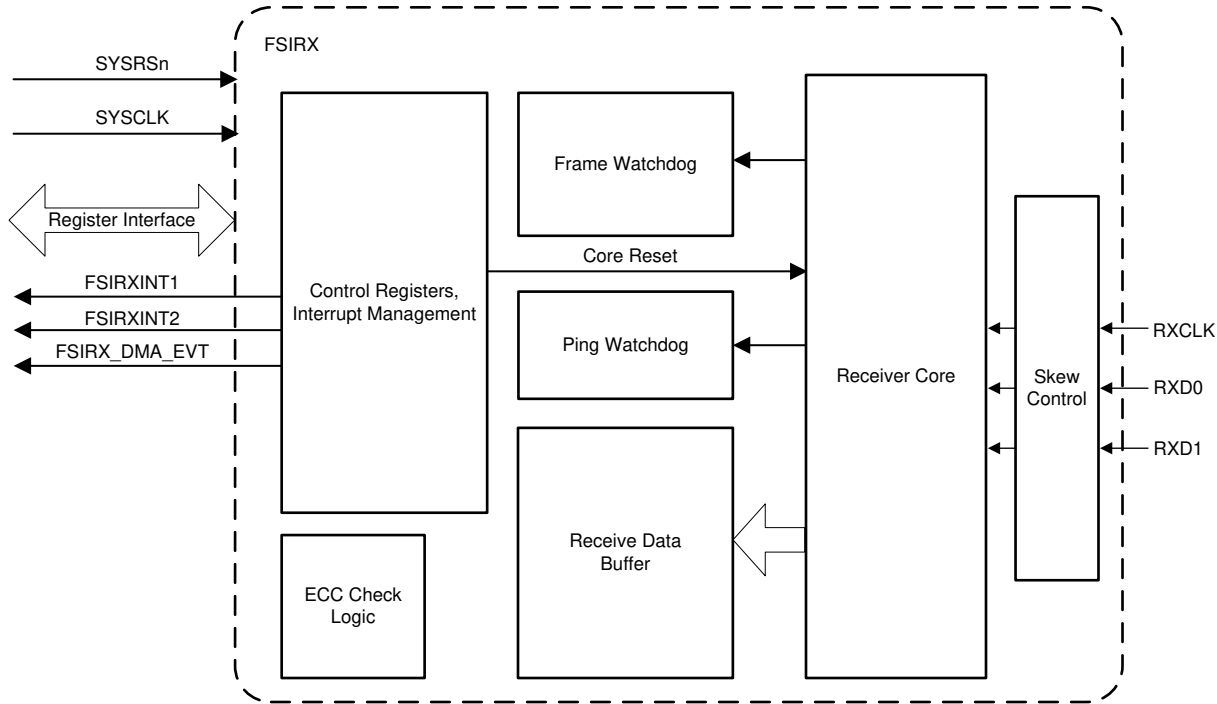
图 6-97. FSIRX 方框图
