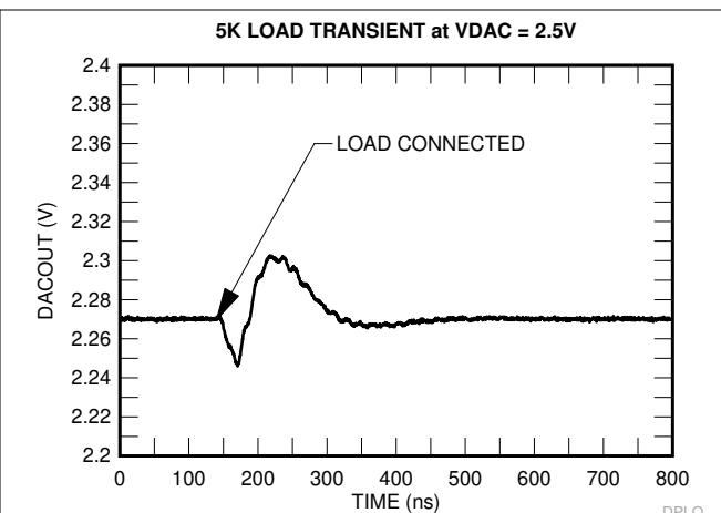
图 6-56. 5k \Omega 负载瞬态
