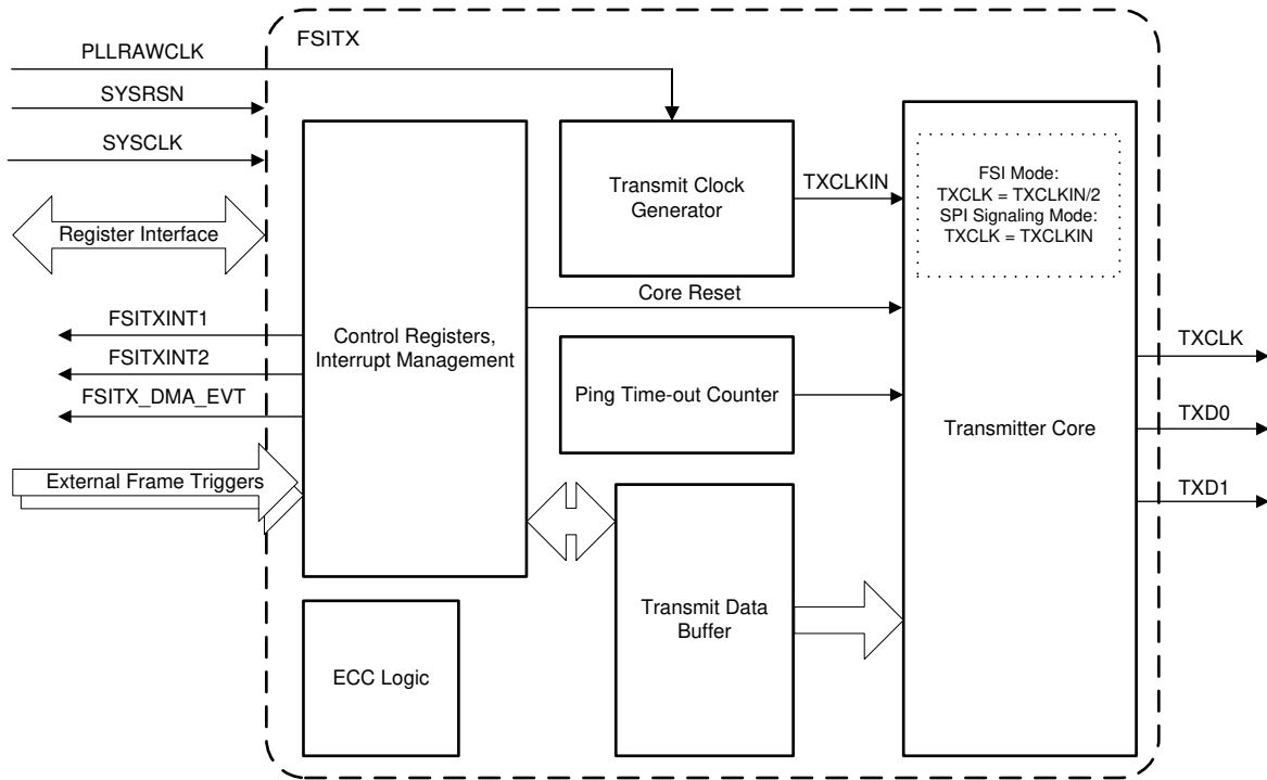
图 6-94. FSITX 方框图
