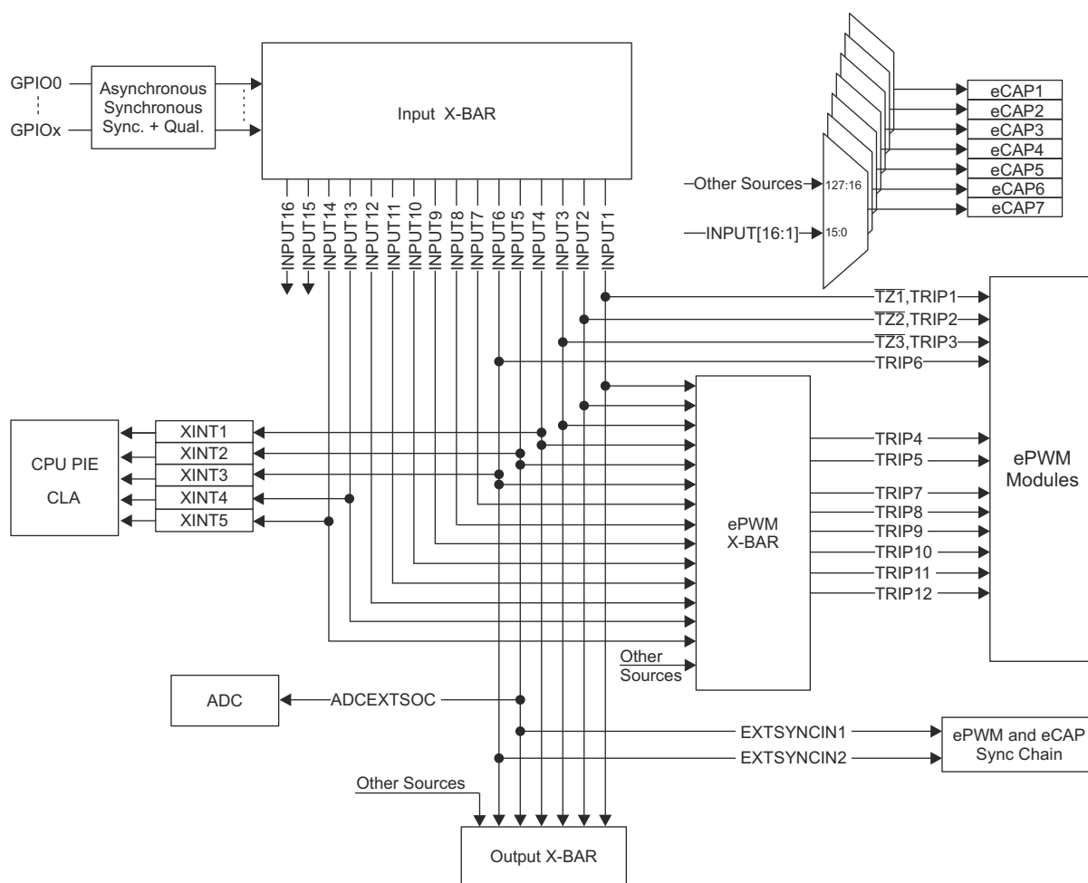
图 6-5. 输入 X-BAR
