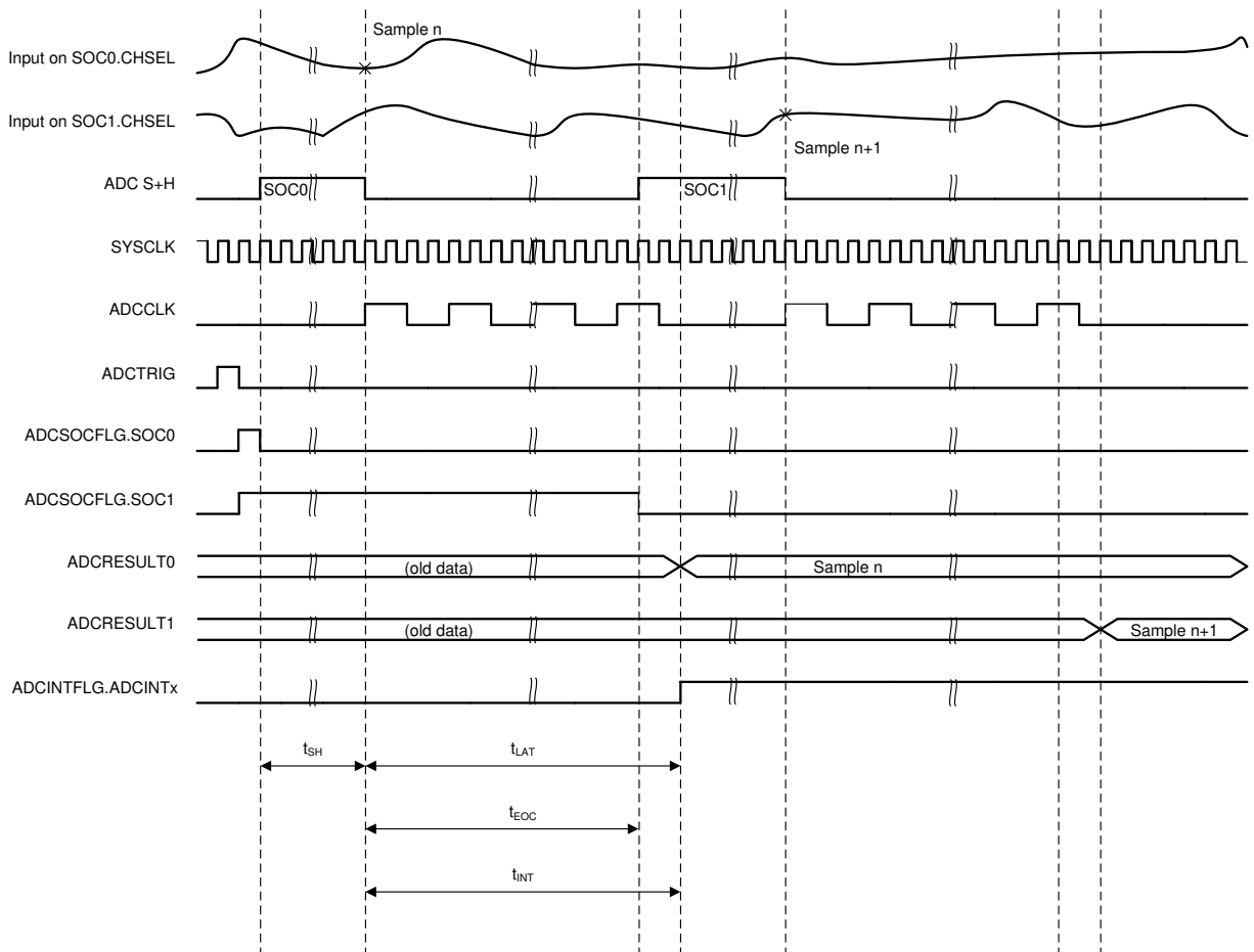
图 7-44. ADC 时序
