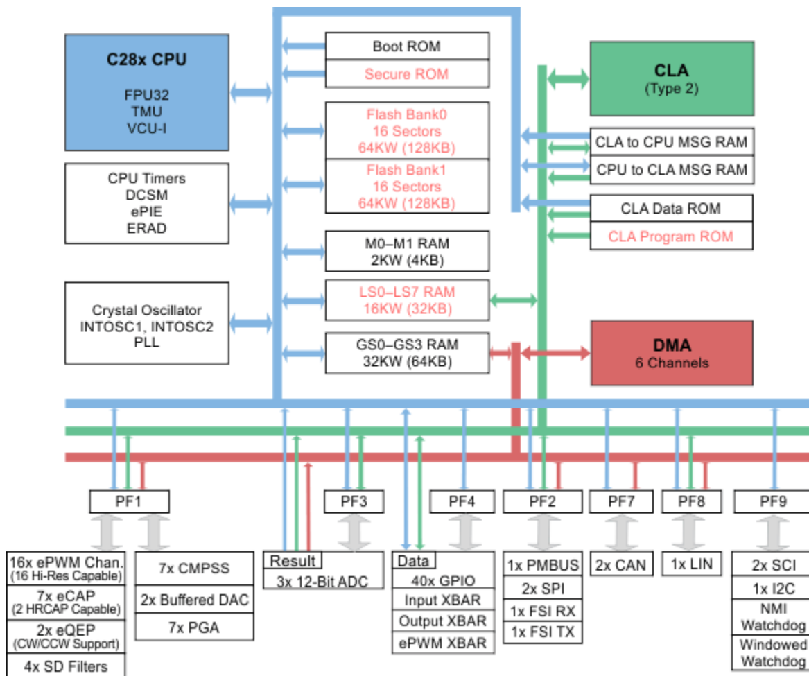
图 3-1. 功能方框图
