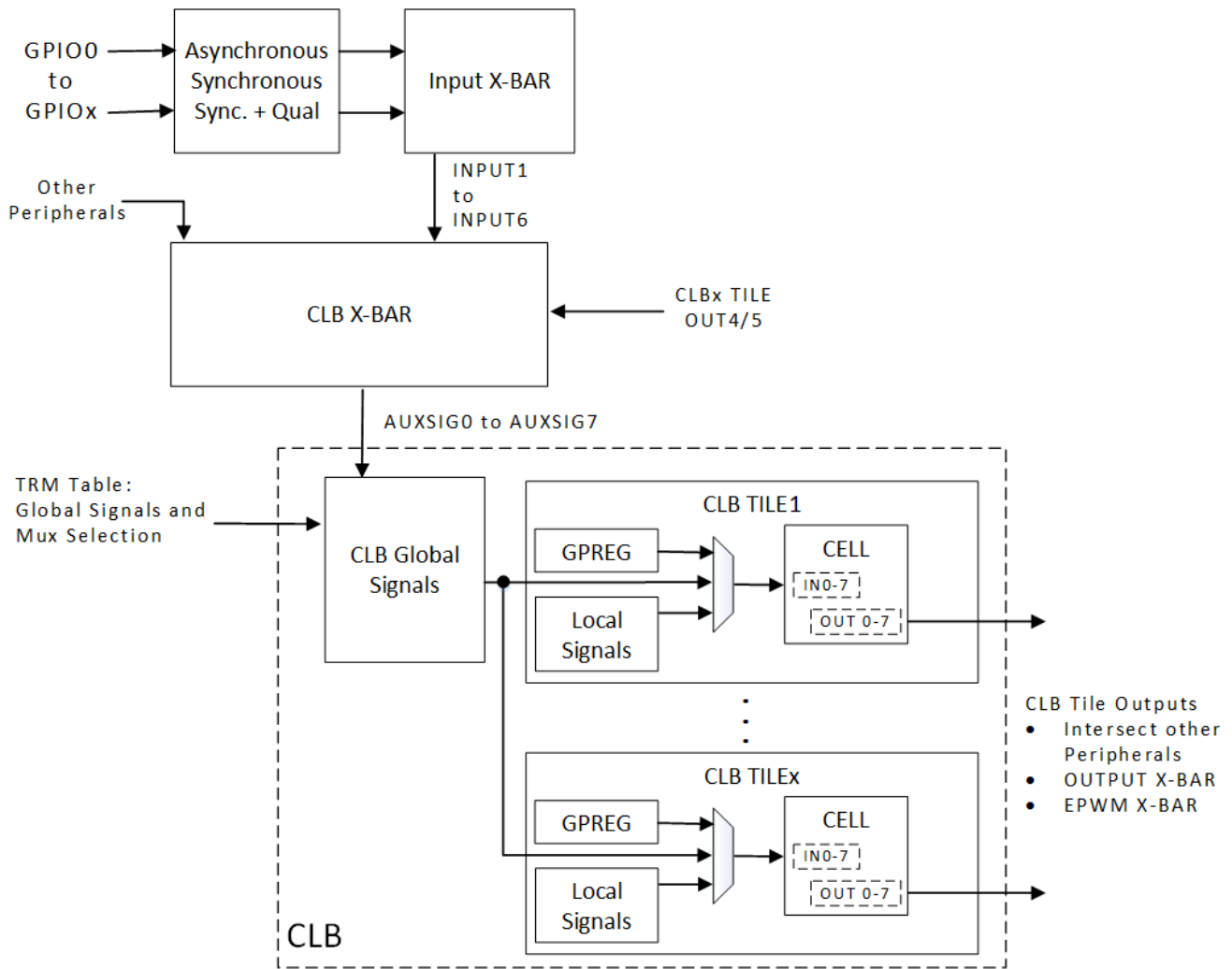
图 8-5. CLB 概述
