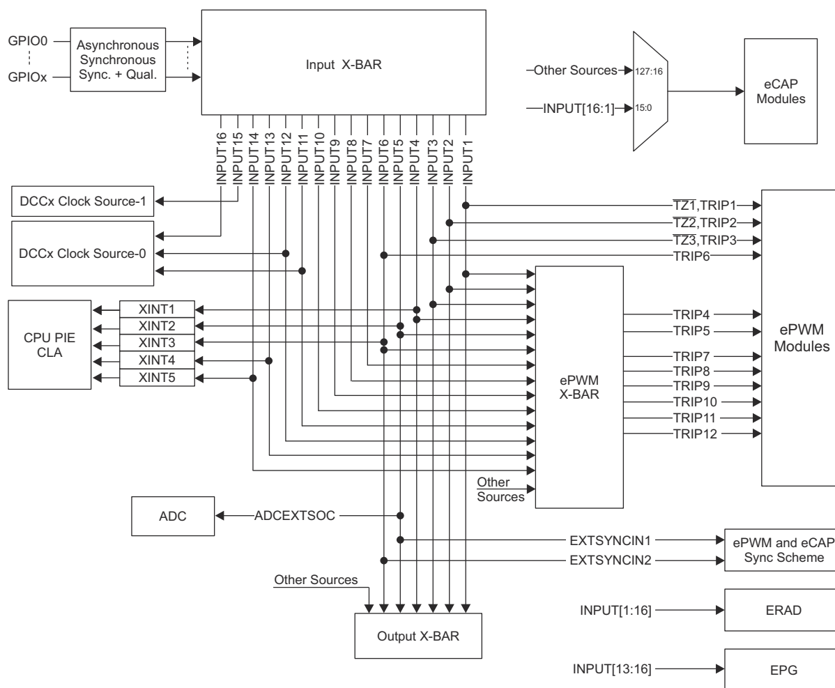
图 5-6. 输入 X-BAR
