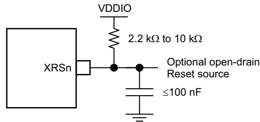
图 6-11. 复位电路
