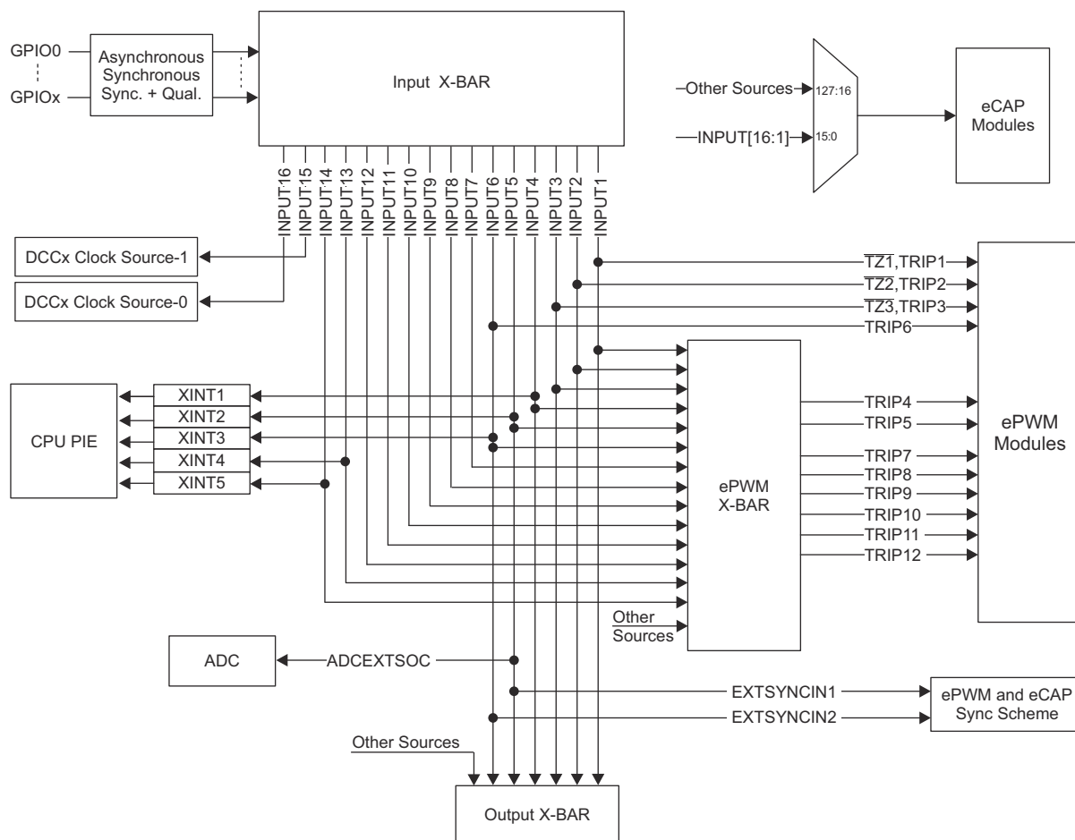
图 5-4. 输入 X-BAR
