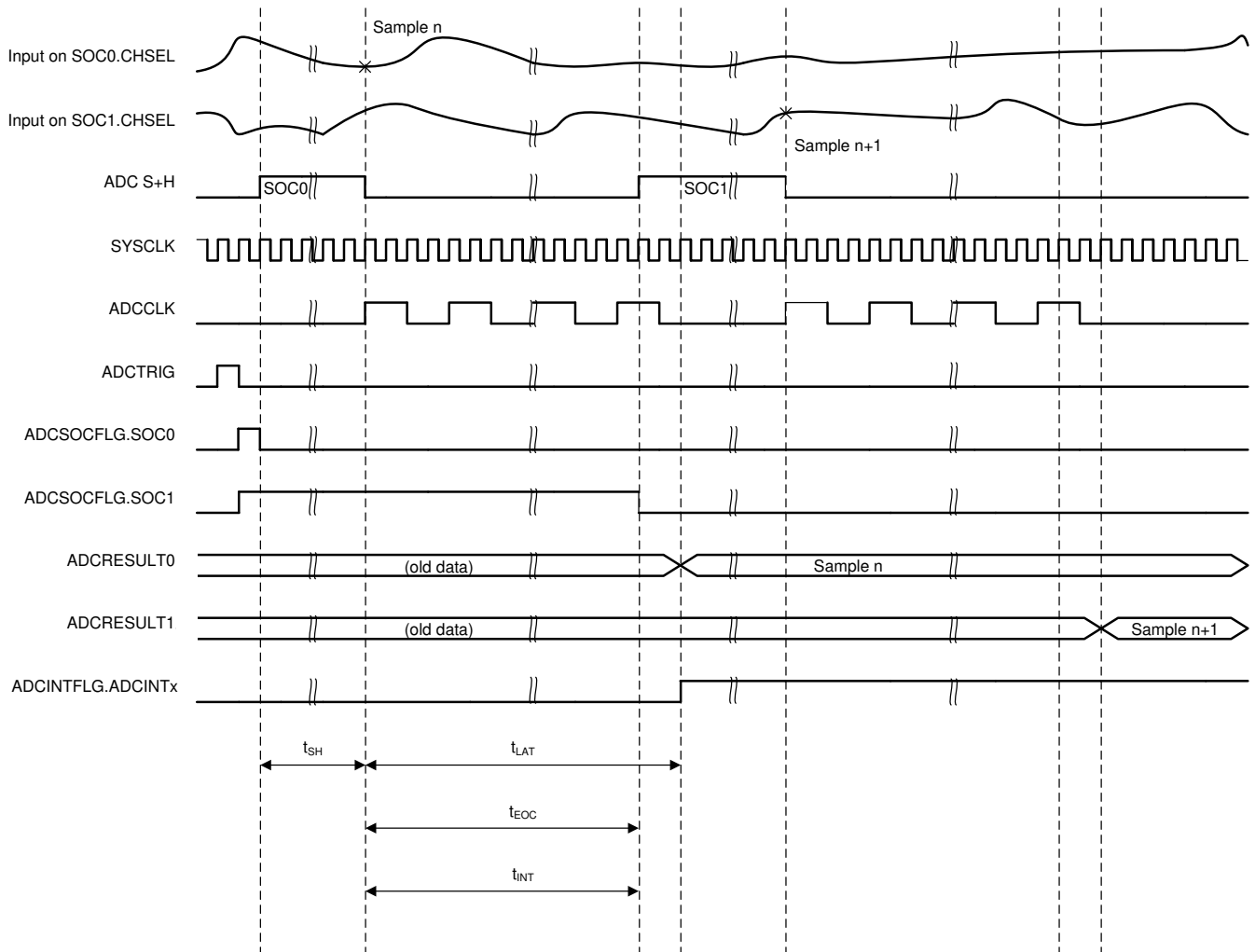
图 6-43. ADC 时序
