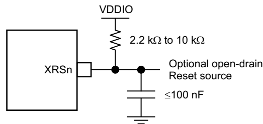
图 6-10. 复位电路
