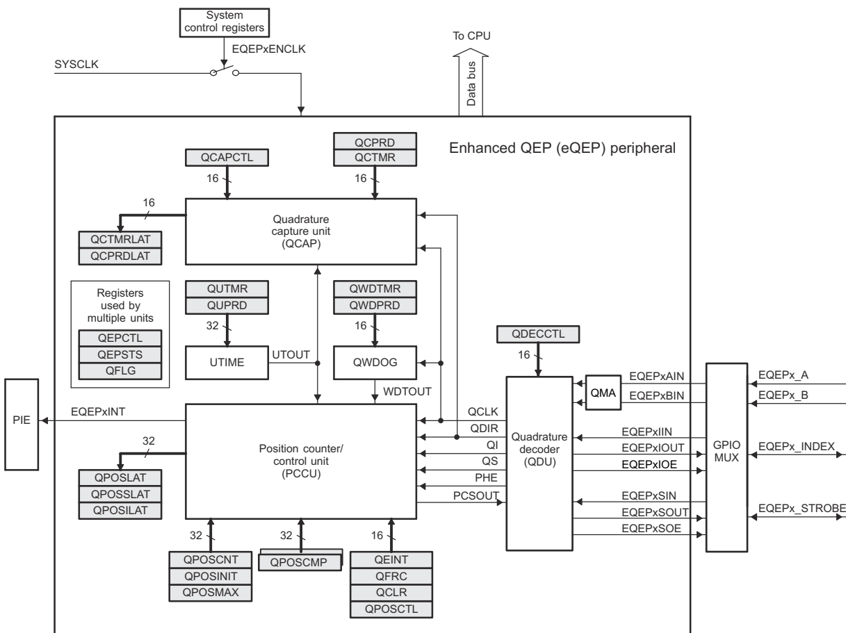
图 6-59. eQEP 方框图
