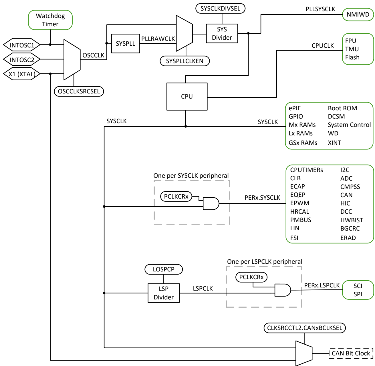
图 6-13. 计时系统
