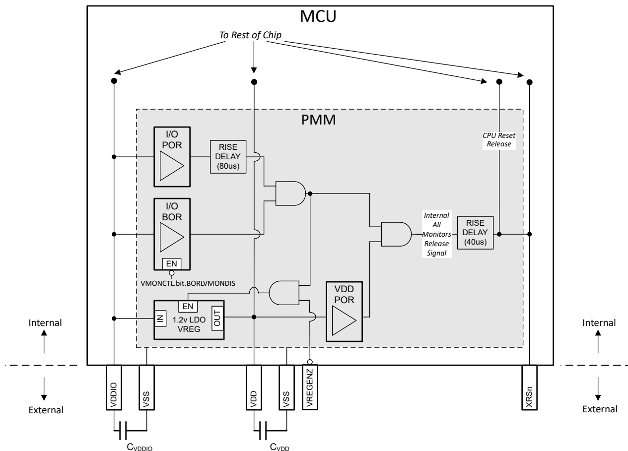
图 6-4. PMM 方框图
