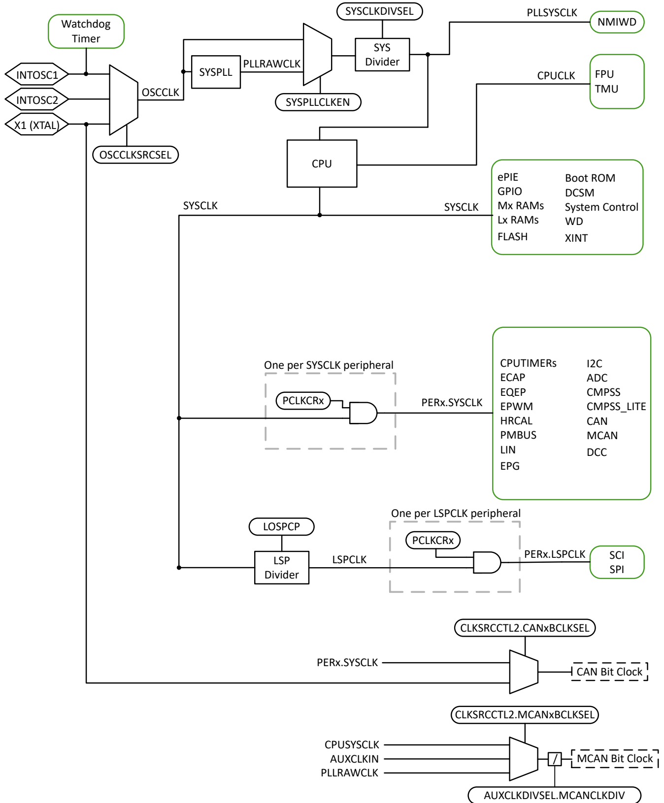
图 6-11. 计时系统
