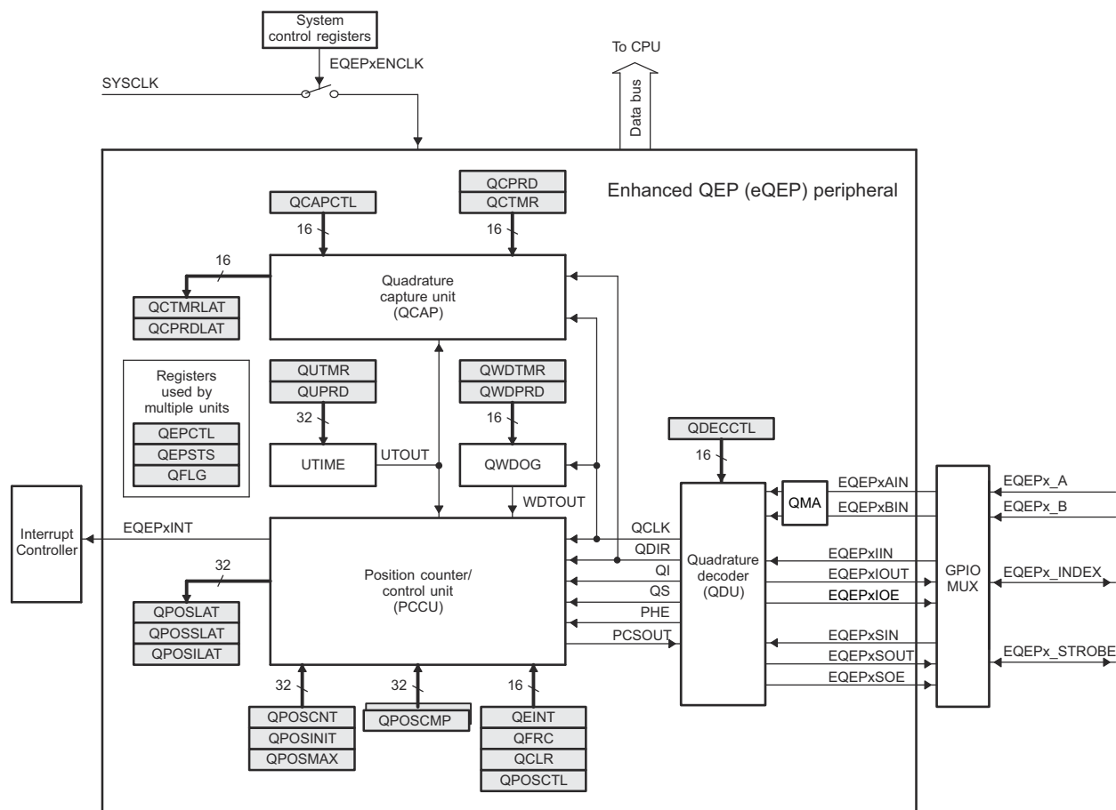
图 6-62. eQEP 方框图
