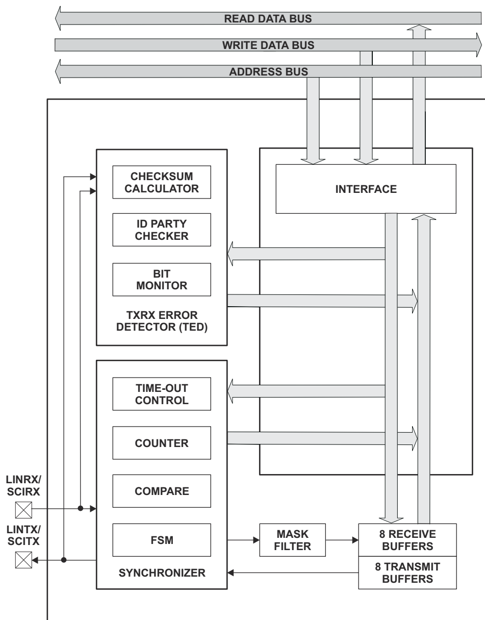
图 6-74. LIN 方框图
