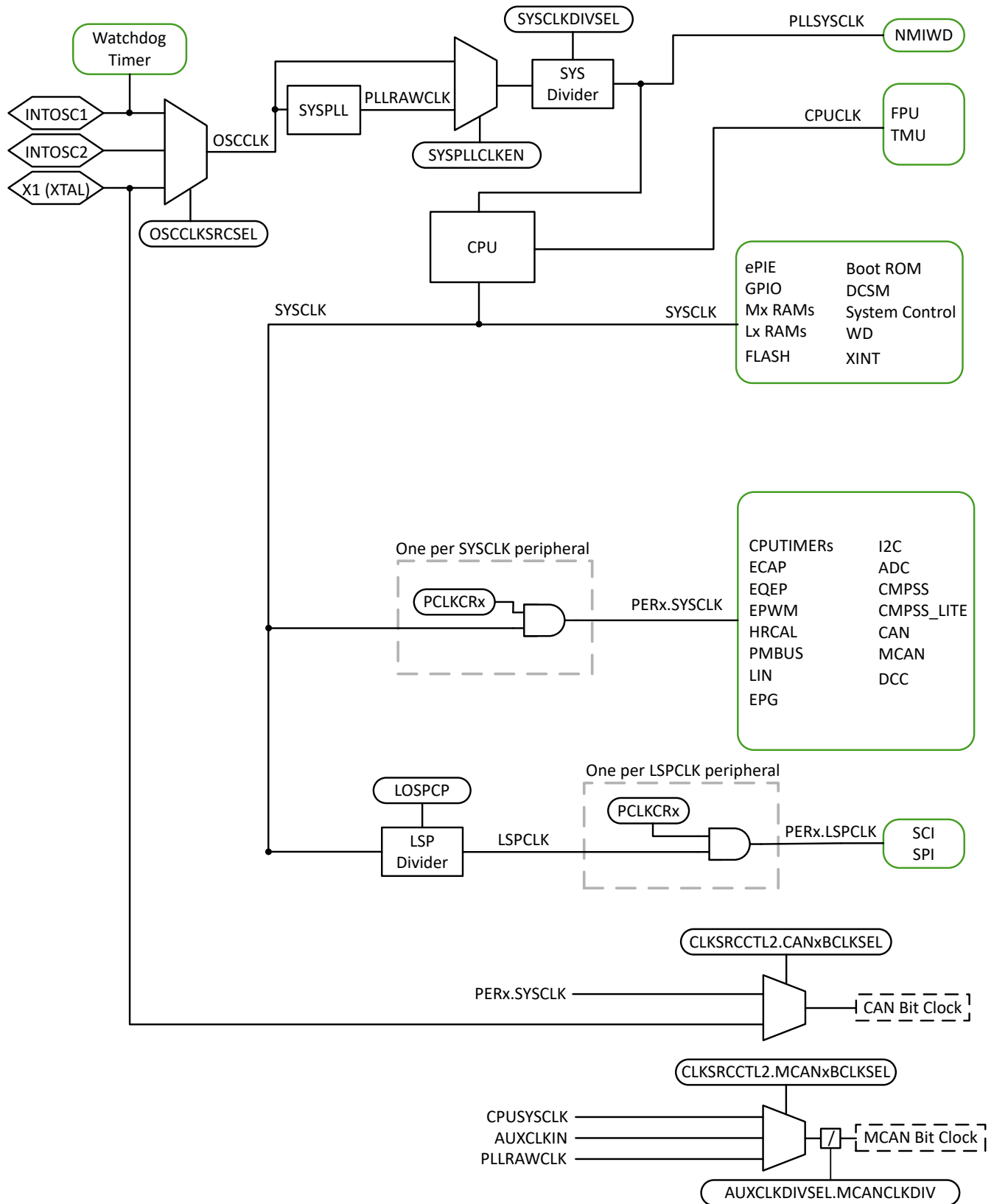
图 6-11. 计时系统
