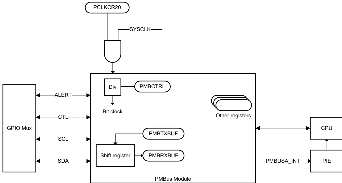
图 6-67. PMBus 方框图
