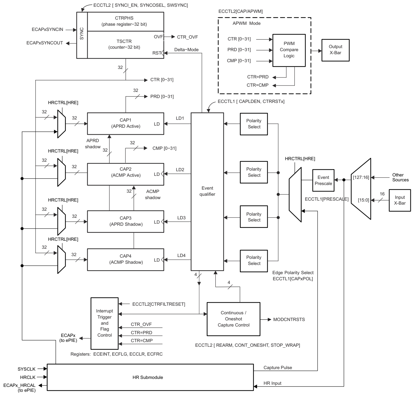
图 6-60. eCAP 方框图
