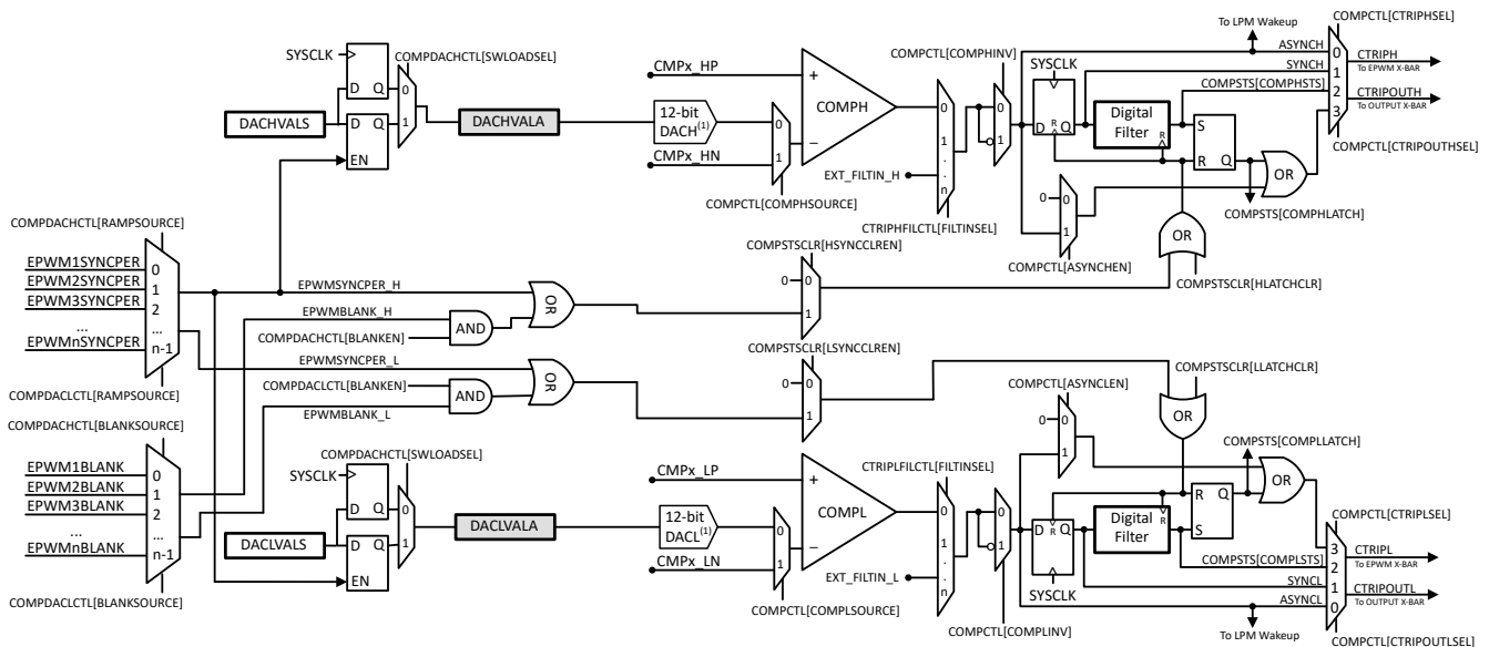
图 6-47. CMPSS_LITE 模块方框图
