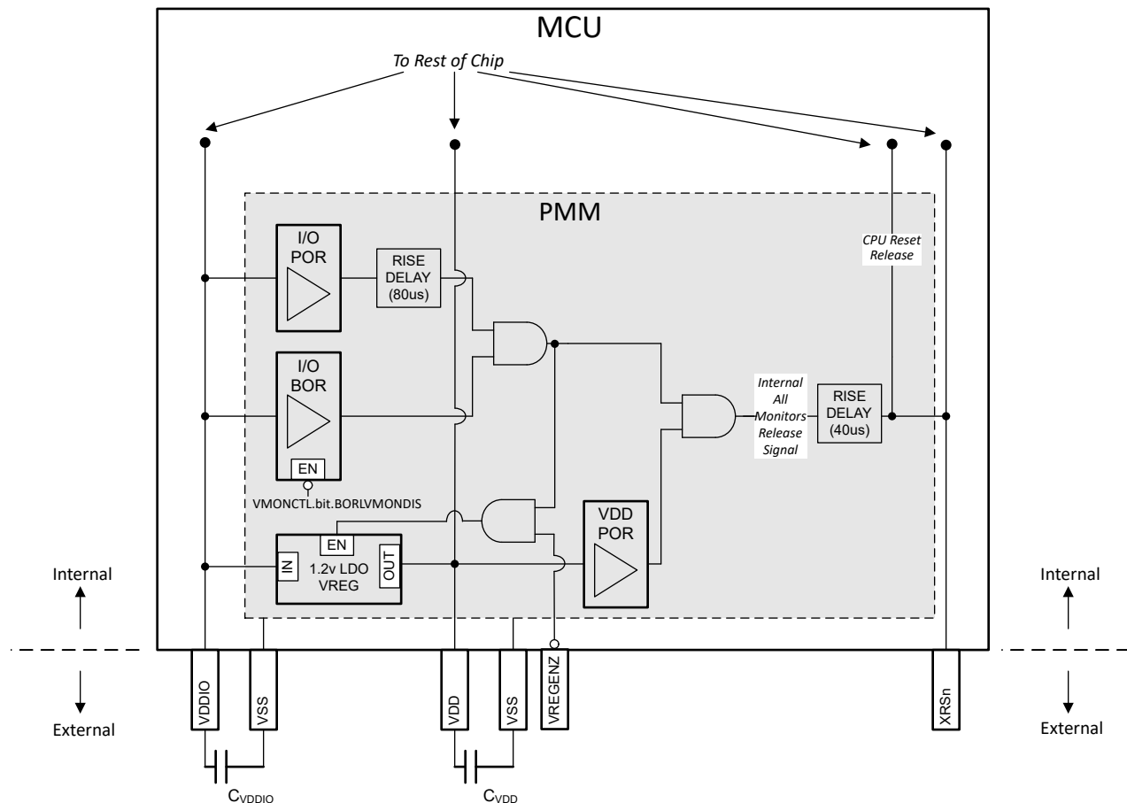
图 6-4. PMM 方框图
