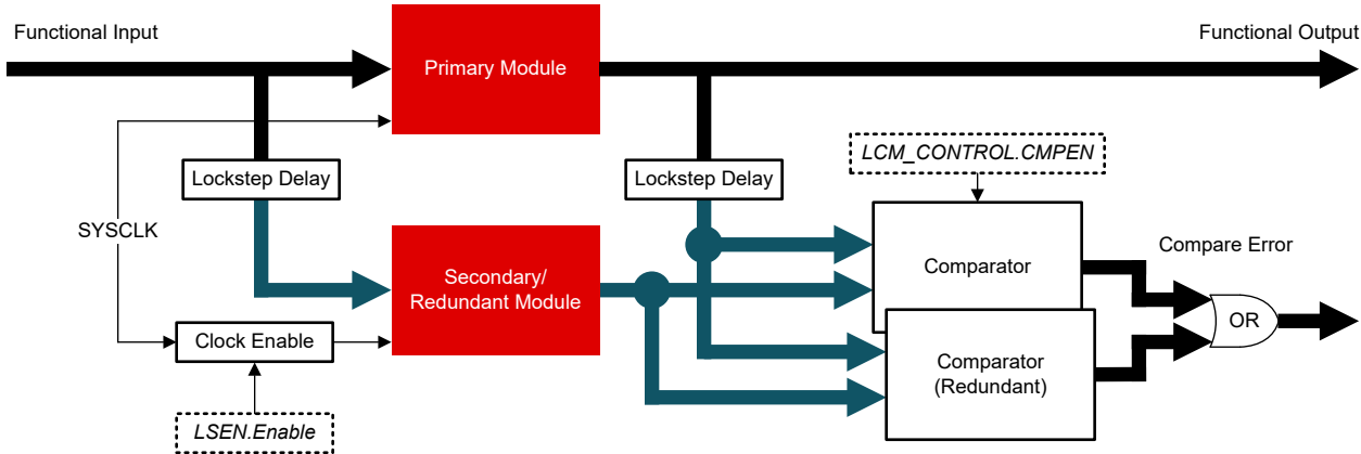
图 7-2. LCM 方框图
