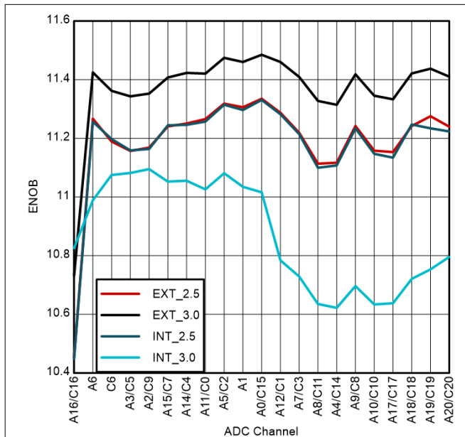
图 6-40. 80 引脚 PN LQFP 和 64 引脚 PM LQFP 的每通道 ENOB
