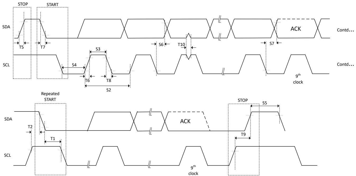
图 6-66. I2C 时序图
