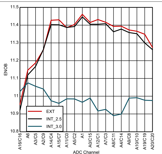
图 6-41. 48 引脚 PHP HTQFP 的每通道 ENOB
