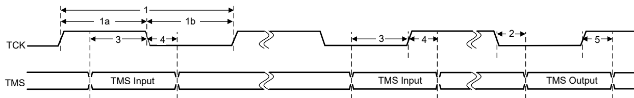
图 6-27. cJTAG 时序
