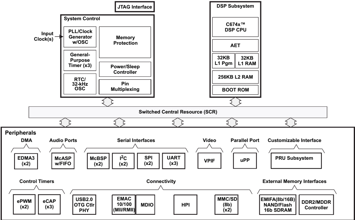
图 1-1. 功能方框图
