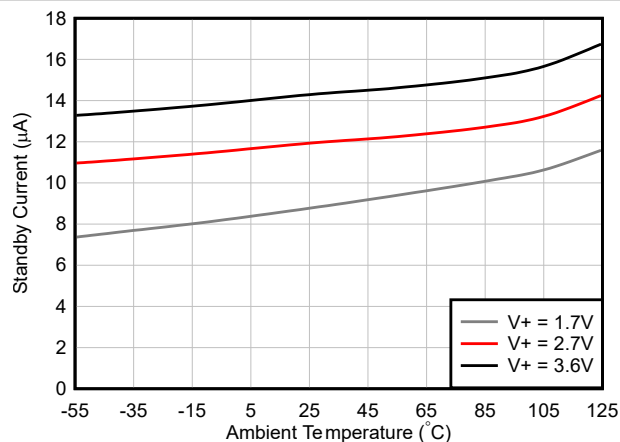
图 6-13. 待机电流与温度间的关系
