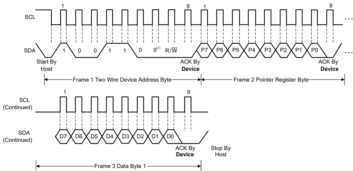
图 7-8. 针对写入字格式的两线制时序图
