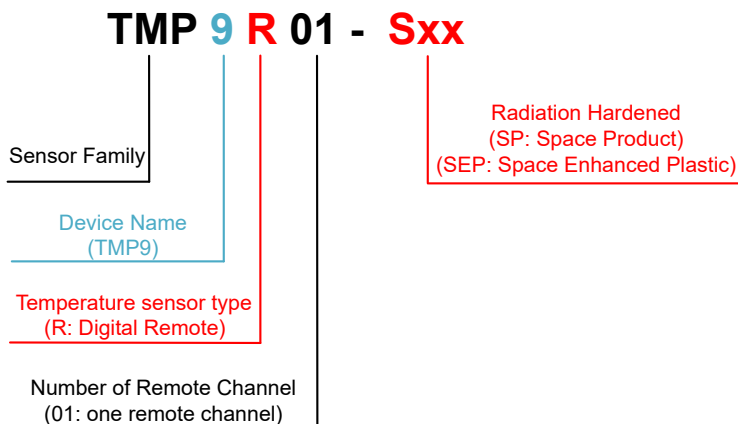
图 4-1. TMP9R01-SP 和 TMP9R01-SEP 器件命名规则
