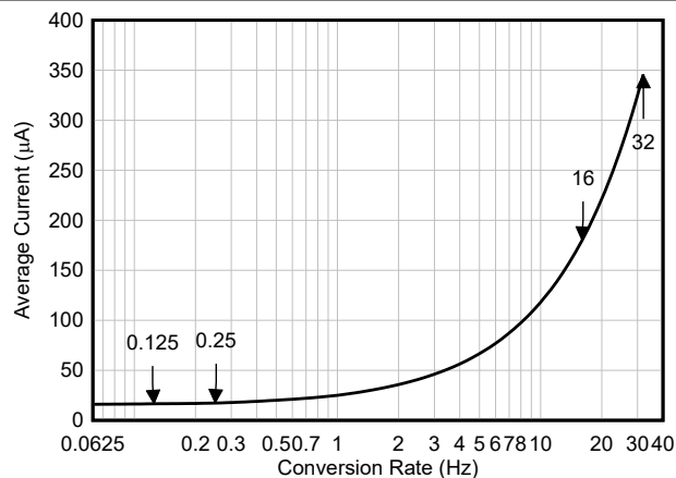
图 6-9. 平均电流与转换速率间的关系
