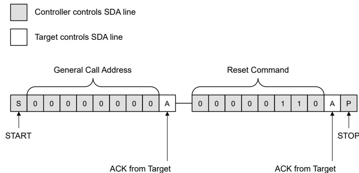
图 7-10. SMBus 通用广播复位时序图
