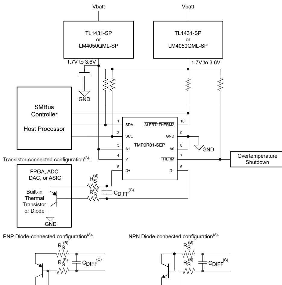
图 7-1. 基本连接
