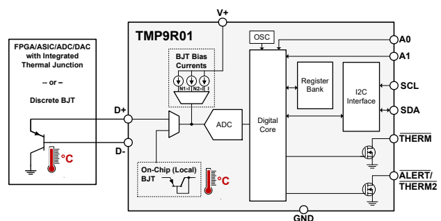
功能方框图
