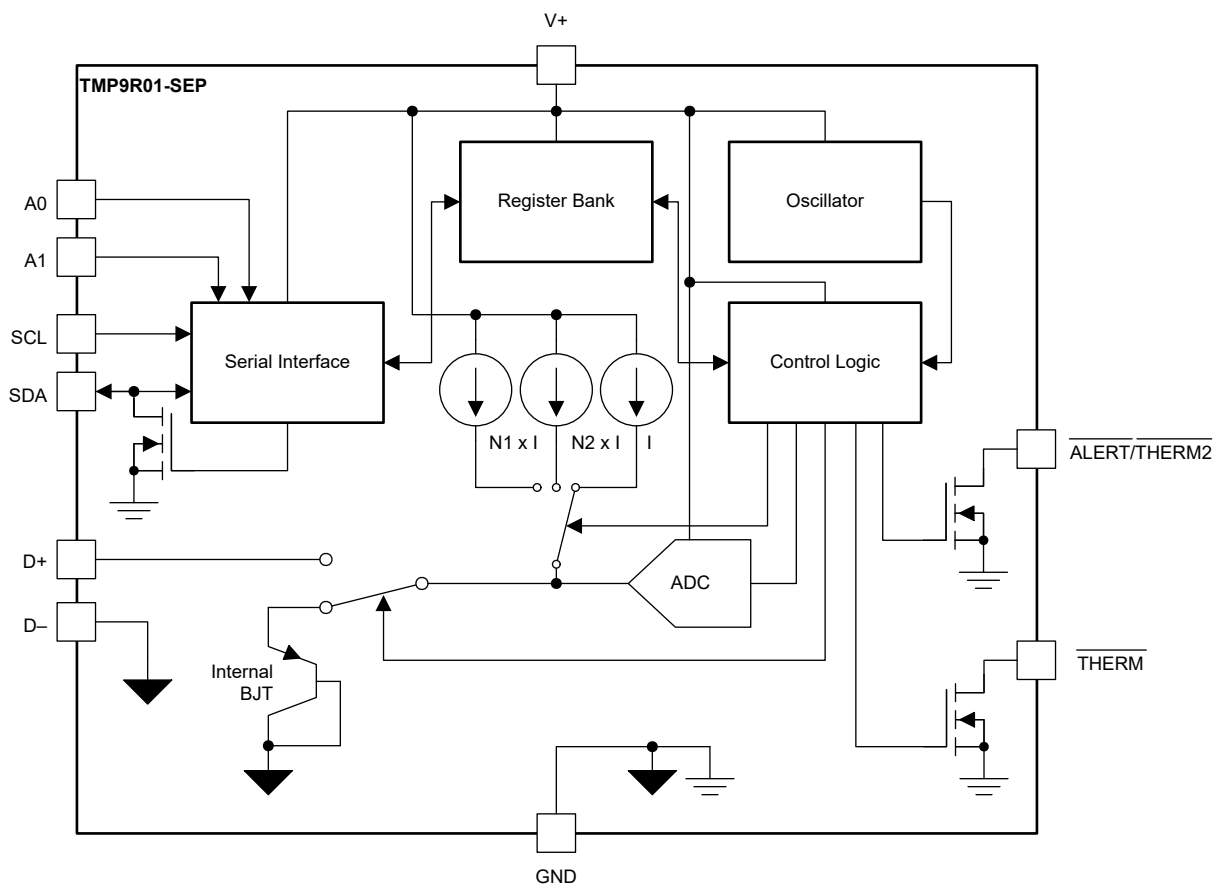
图 7-2. 功能方框图
