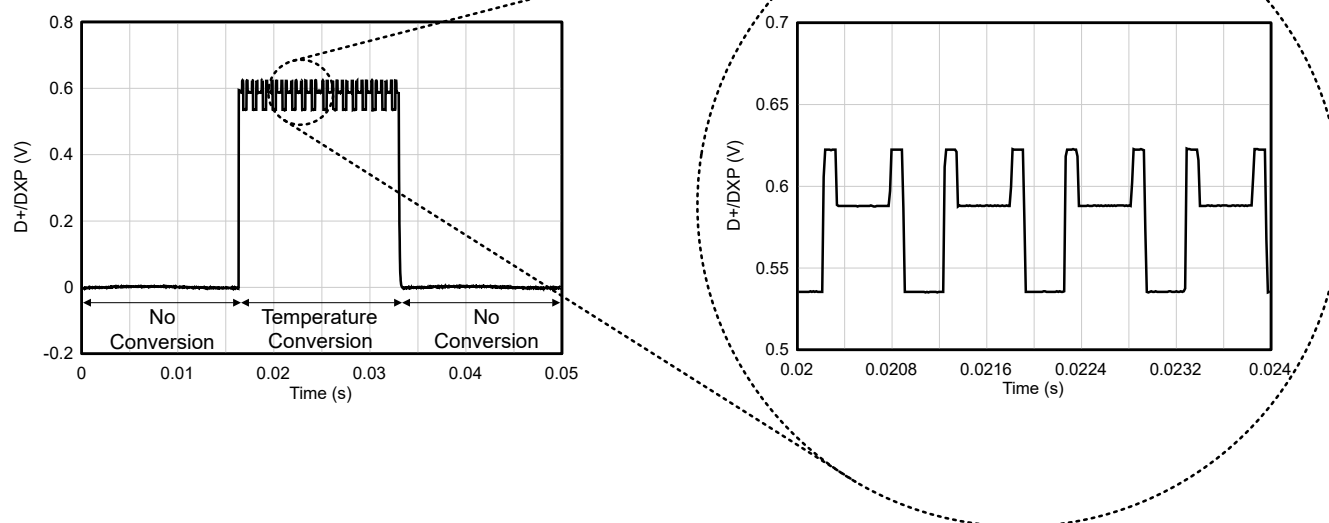
图 9-2. D+ 波形
