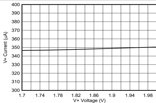
图 6-8. 静态电流与电源电压之间的关系 (默认转换率, 每秒 16 次转换)
