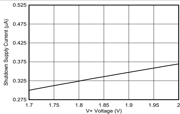
图 6-9. 关断静态电流与电源电压之间的关系
