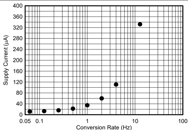
图 6-6. 静态电流与转换率之间的关系
