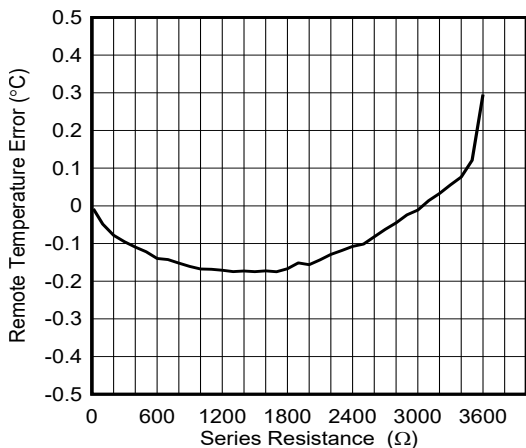
图 6-4. 远程温度误差与串联电阻之间的关系
