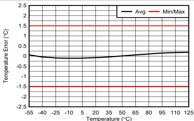
图 6-2. 本地温度误差与环境温度之间的关系
