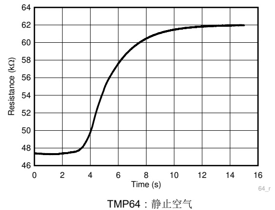
图 7-10. 热响应时间
