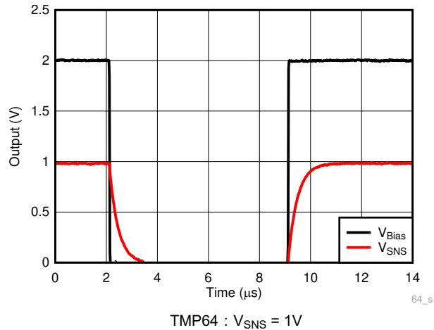
图 7-7. 阶跃响应
