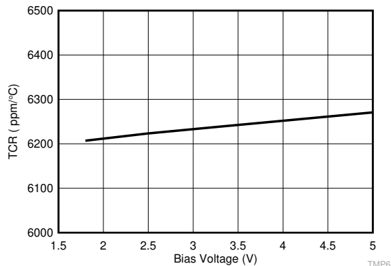
图 6-4. TCR 是检测电压 V_{\text{SNS}} 的函数
