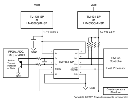
简化框图
