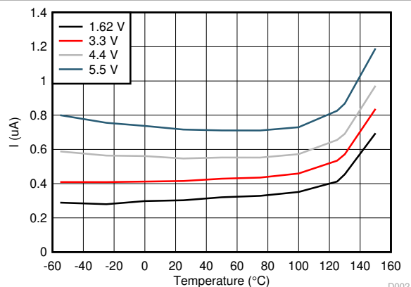
图 6-1. 平均电源电流与工作温度间的关系
