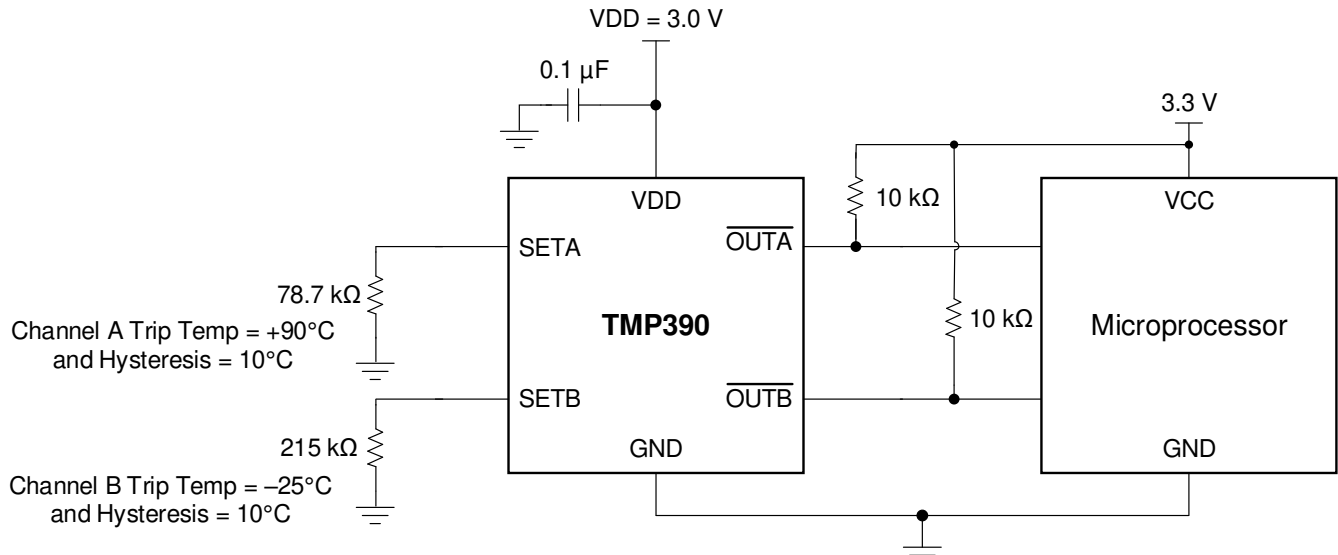
图 8-3. 阈值为 +90°C 和 -25°C 且迟滞为 10°C 的 TMP390 示例电路
