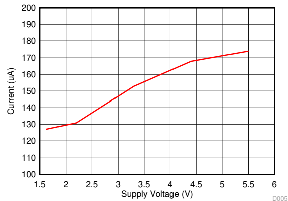
图 6-4. 转换电流与电源电压间的关系
