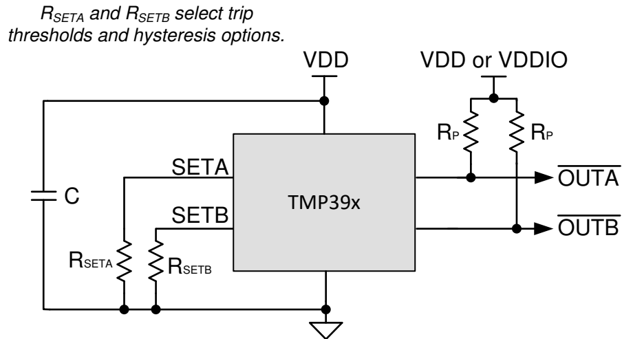
图 7-1. 简化原理图
