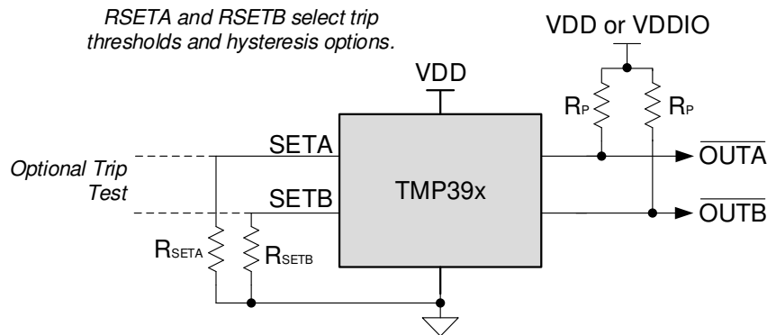
图 8-1. 简化原理图
