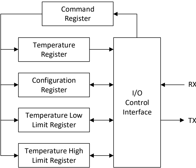
图 7-17. 内部寄存器结构
