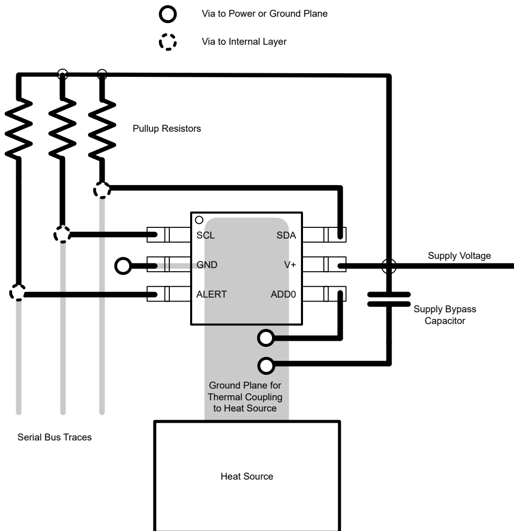
图 8-8. DRL 布局示例
