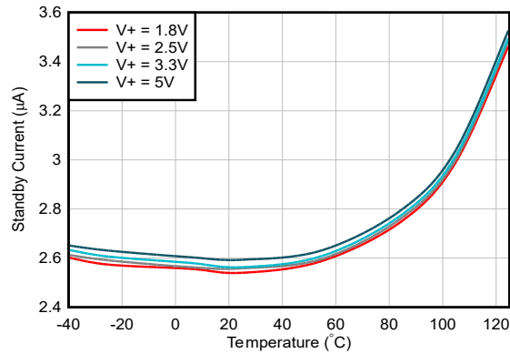
图 6-15. 待机电流与温度间的关系
