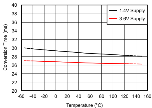
图 6-8. 转换时间与温度间的关系
