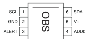
图 5-2. DRL 封装 6 引脚 SOT563 TMP112D-Q1 和 TMP112-Q1 (顶视图)
