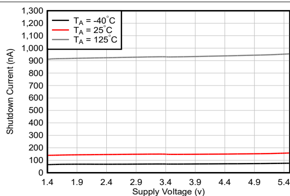
图 6-11. 关断电流与电源电压间的关系
