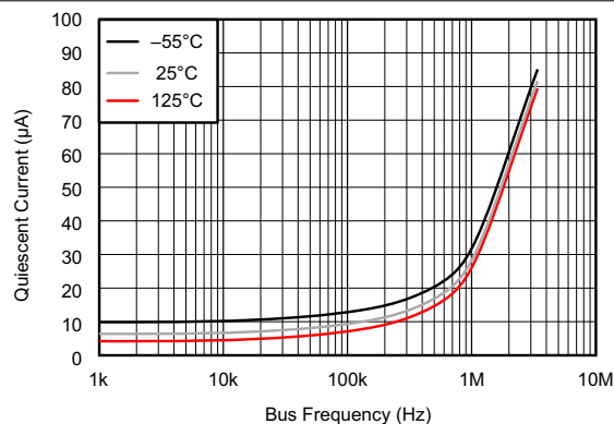
图 6-5. 平均静态电流与温度间的关系
