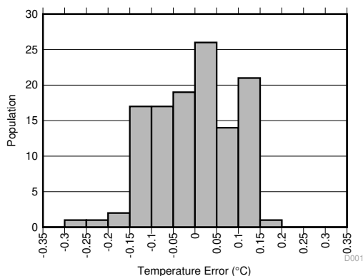
图 6-2. 25^\circ\text{C} 时的温度误差
