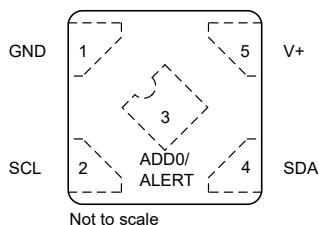
图 5-1. DPW 封装 5 引脚 X2SON TMP112D-Q1 (顶视图)
