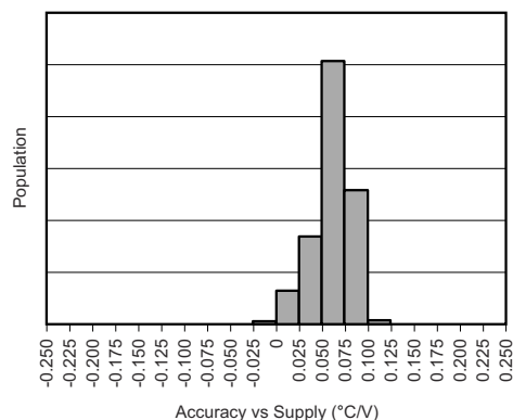
图 6-3. 精度与电源间的关系
