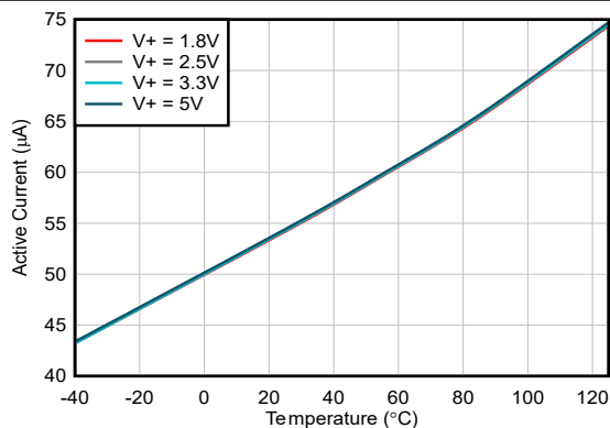
图 6-13. 有效转换电流与温度间的关系
