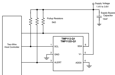
简化版原理图 (SOT563 封装)
