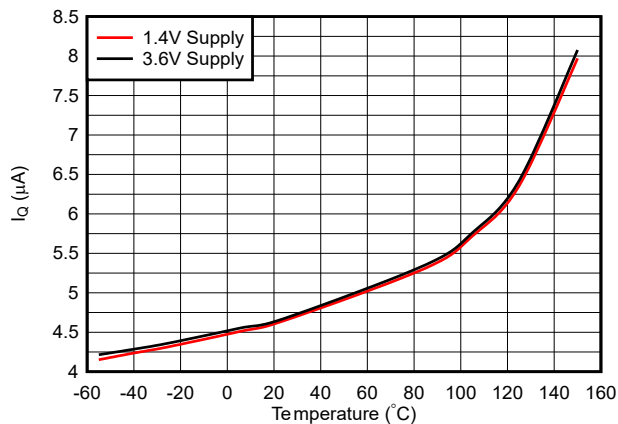
图 6-5. 平均静态电流与温度间的关系
