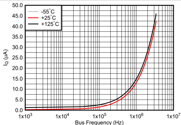
图 6-7. 静态电流与总线频率间的关系 (由 3.3\text{V} 电源供电时的温度)
