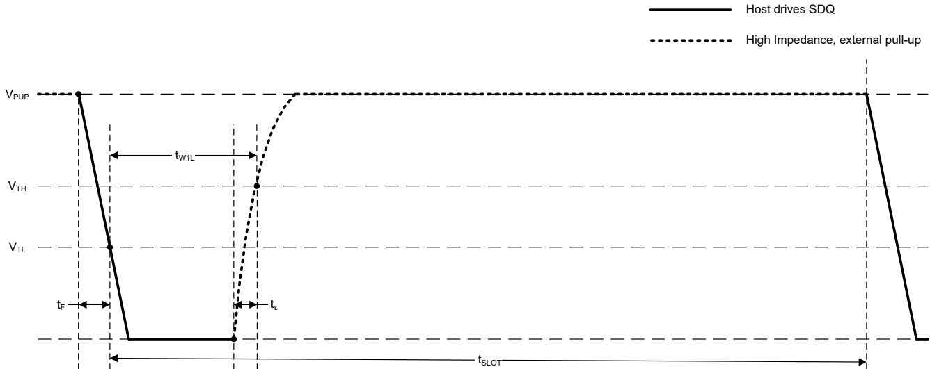
图 6-18. 写入“1”时序图
