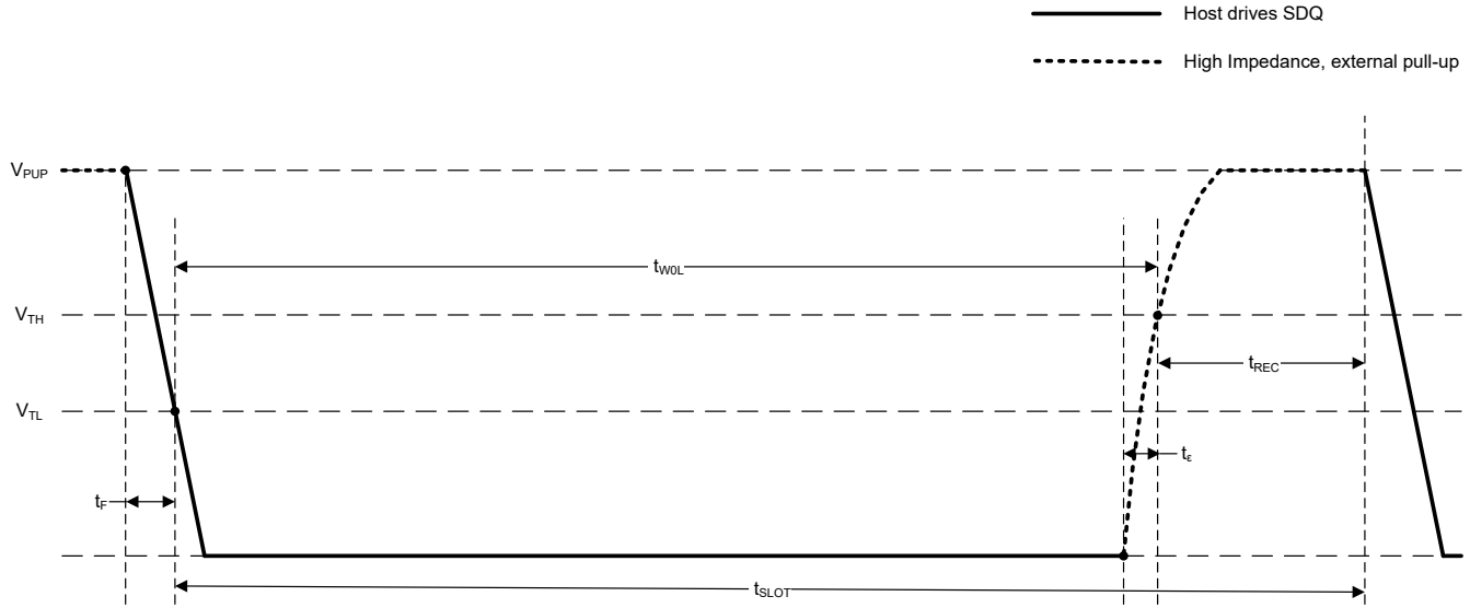
图 6-19. 写入“0”时序图
