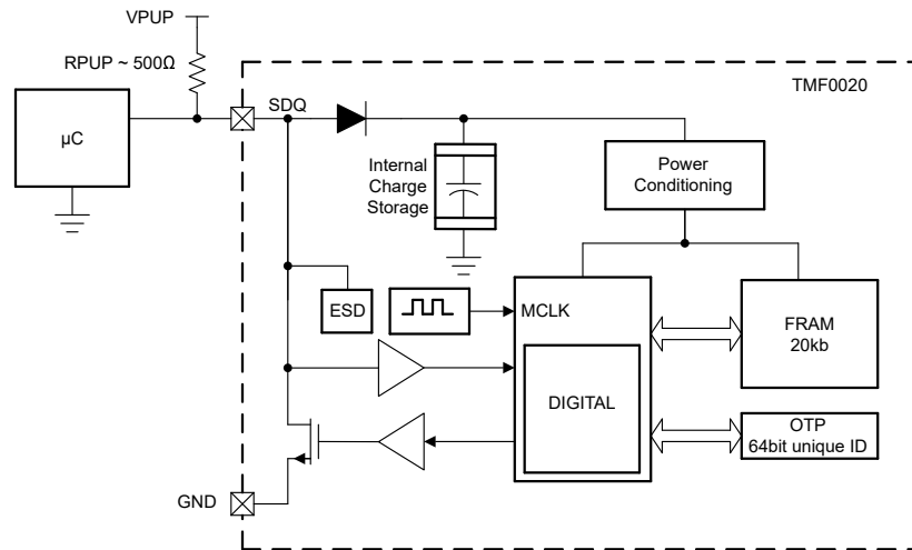
图 6-1. 功能方框图
