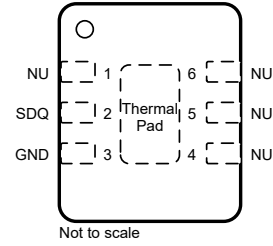
图 4-2. DRP 封装，6 引脚 VSON (俯视图)
