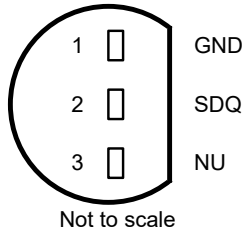
图 4-1. LP 封装、3 引脚 TO-92 (底视图)
