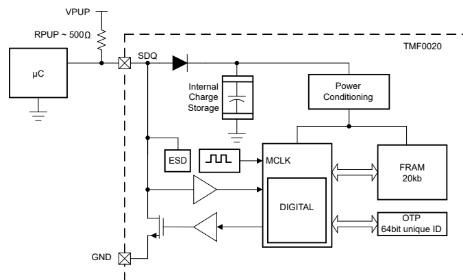
方框图
