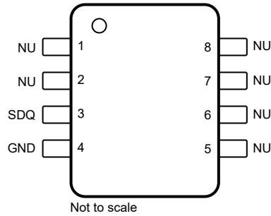
图 4-3. TMF0008 PS 封装, 8 引脚 SOIC (顶视图)
