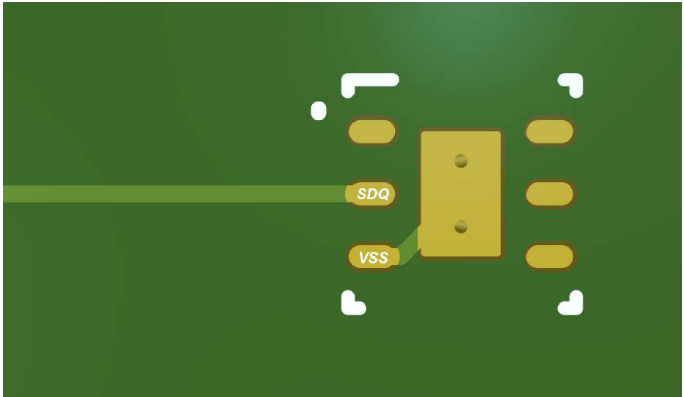
图 7-5. 电路板布局示例
