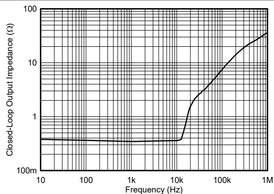
图 6-14. 输出阻抗与频率间的关系
