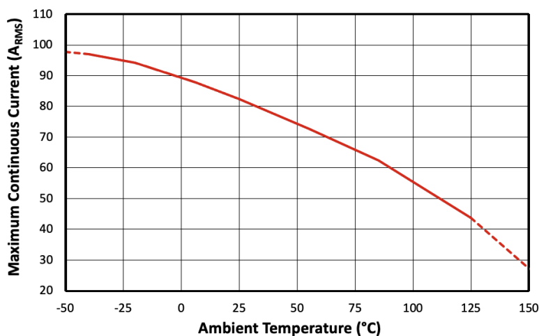
图 7-4. 最大连续 RMS 电流与环境温度间的关系
