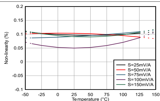
图 6-4. 非线性与温度间的关系
