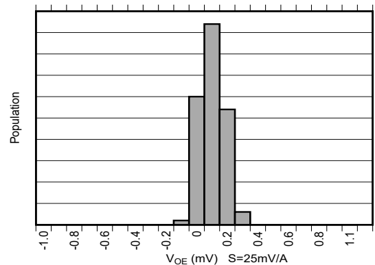
图 6-6. 失调误差产生分布图
