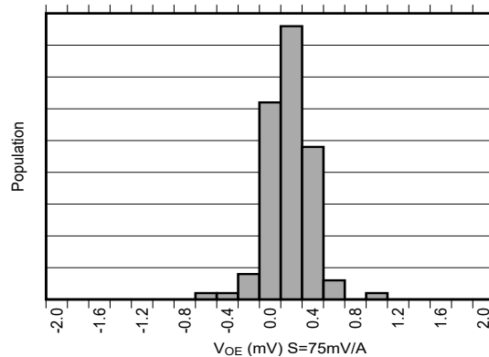
图 6-8. 失调误差产生分布图
