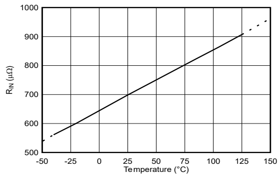
图 6-22. 输入导体电阻与温度间的关系
