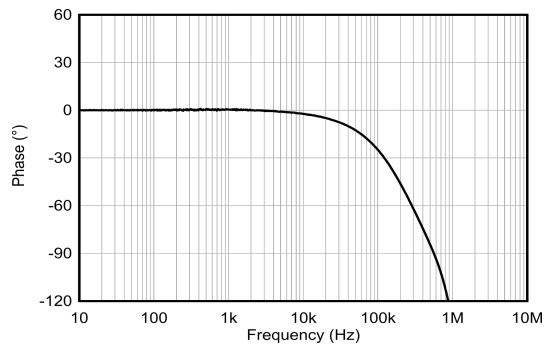
图 6-12. 相位与频率间的关系 (所有增益)
