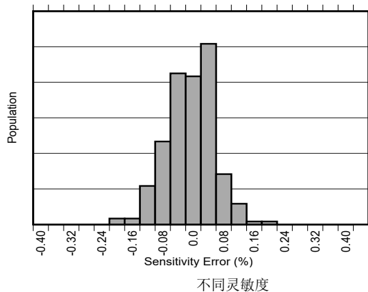
图 6-5. 灵敏度误差产生分布图
