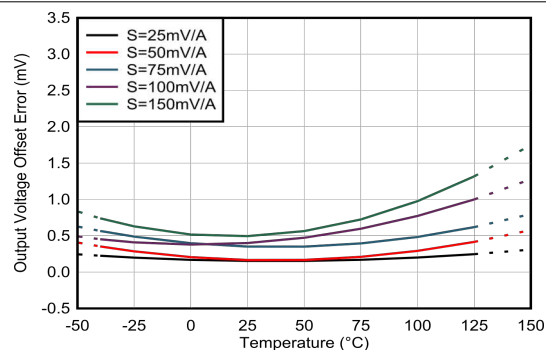
图 6-2. 失调误差与温度间的关系
