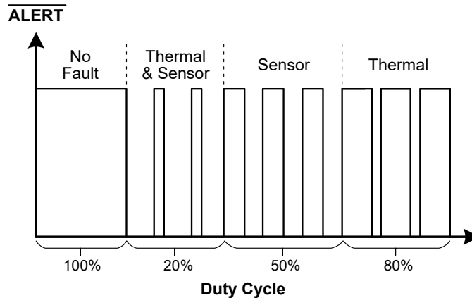
图 8-10. 传感器诊断波形
