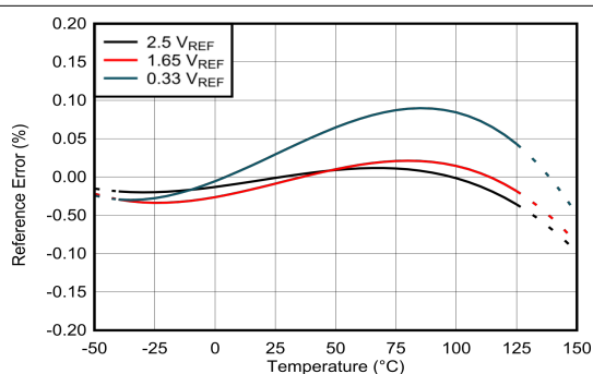
图 6-3. 基准误差与温度间的关系
