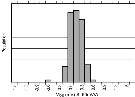
图 6-7. 失调误差产生分布图
