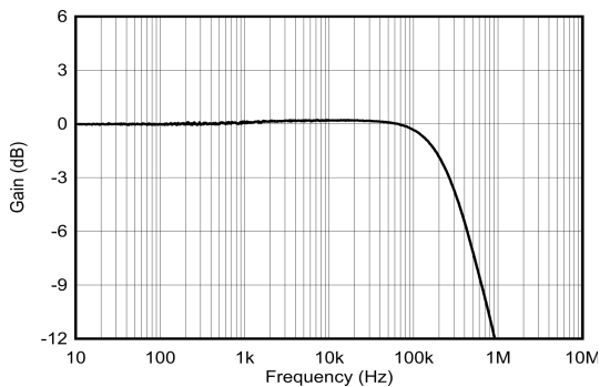
图 6-11. 灵敏度与频率间的关系 (所有增益都归一化为 1Hz)
