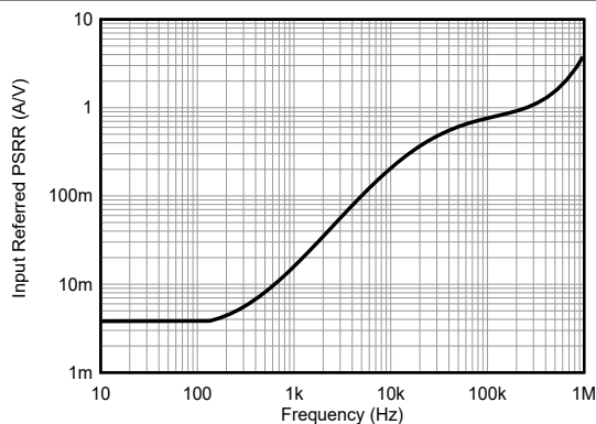
图 6-13. PSRR 与频率间的关系
