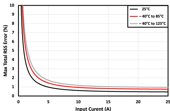
图 9-1. RSS 误差与输入电流间的关系
