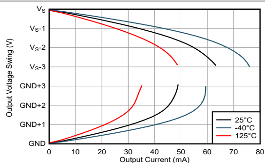
图 6-20. 输出摆幅与输出电流间的关系
