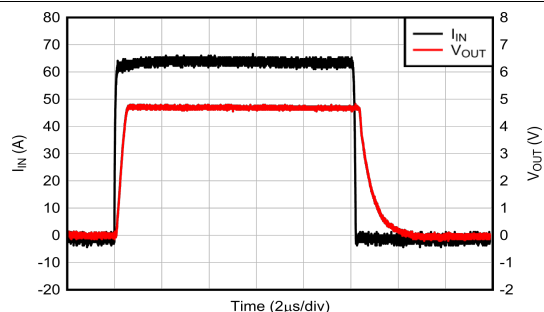
图 6-18. 电流过载响应
