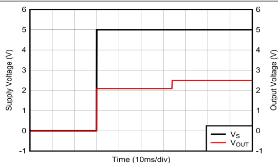
图 6-19. 启动瞬态响应
