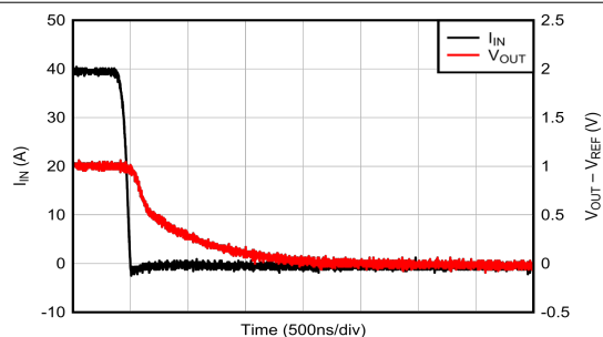
图 6-16. 电压输出阶跃响应 (下降)
