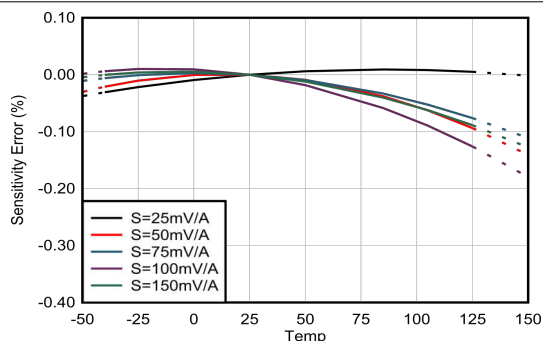
图 6-1. 灵敏度误差与温度间的关系
