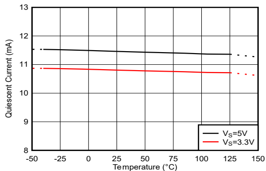
图 6-21. 静态电流与温度间的关系
