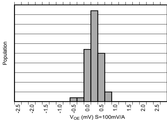
图 6-9. 失调误差产生分布图
