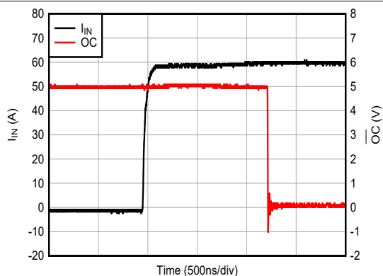
图 6-17. 带掩码的过流输出响应
