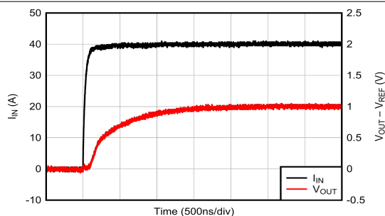
图 6-15. 电压输出阶跃响应 (上升)
