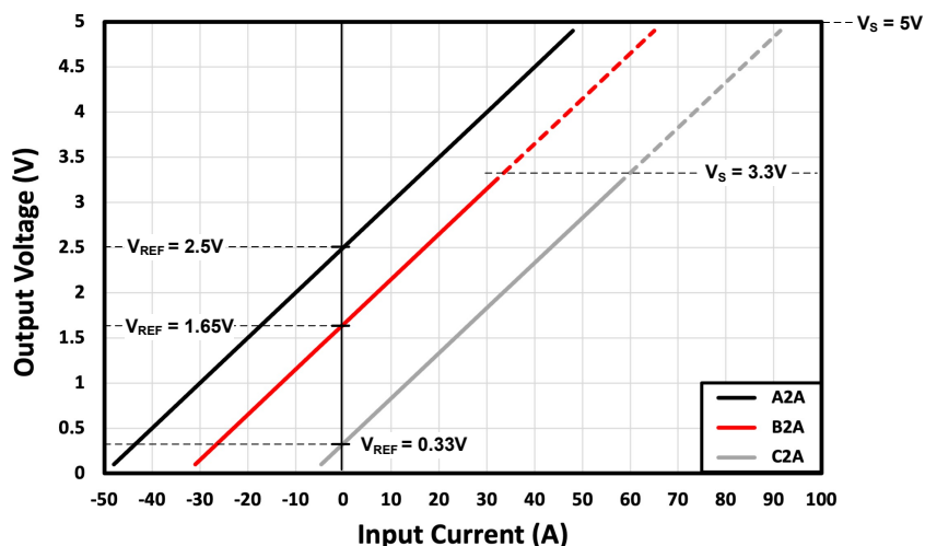
图 8-5. TMCS1123x2A 的输出电压与输入电流之间的关系
