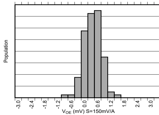
图 6-10. 失调误差产生分布图
