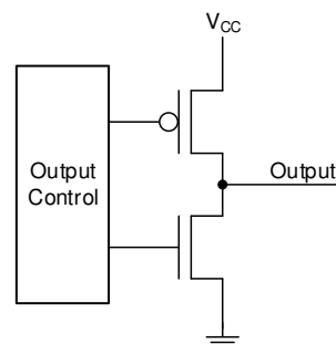
图 7-7. 推挽式 (CMOS) 输出 (简化版)
