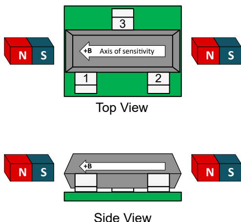
图 7-2. 正磁通密度
