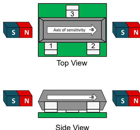
图 7-3. 负磁通密度
