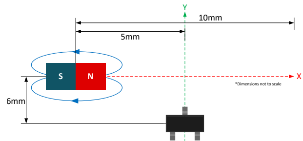
图 8-3. 顶视图
