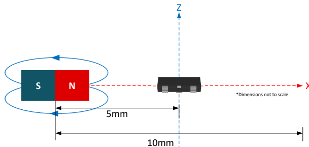
图 8-2. 侧视图
