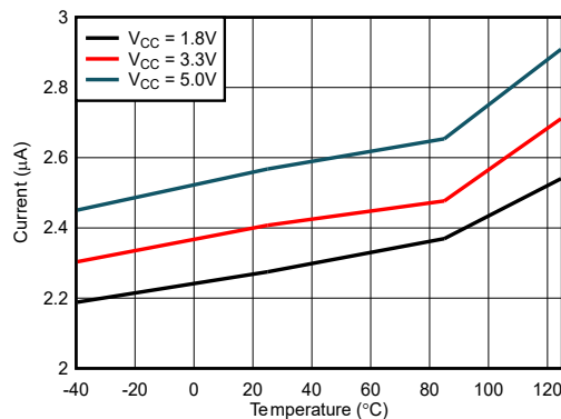
图 6-8. 20Hz I CAVG 与温度之间的关系
