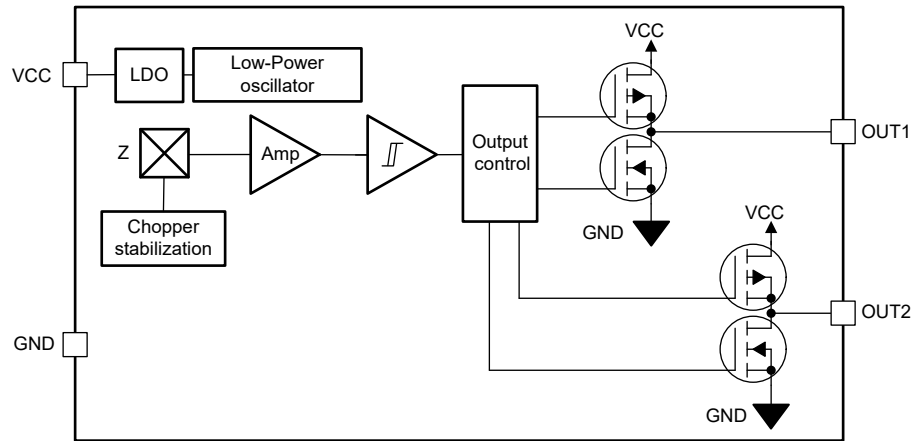
图 7-1. 方框图
