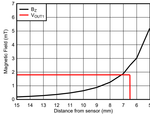
图 8-2. TMAG5230D5D 对 B_{EXT} 的响应
