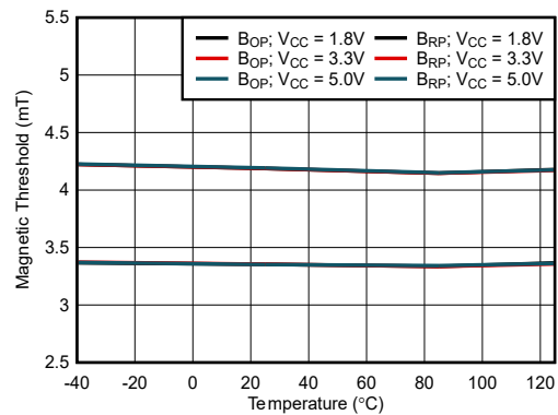
图 6-4. 4.1mT B_{OP} : 阈值与温度间的关系
