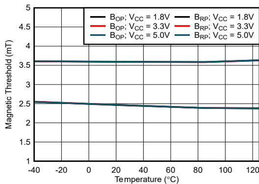
图 6-3. 3.5mT B_{OP} : 阈值与温度间的关系
