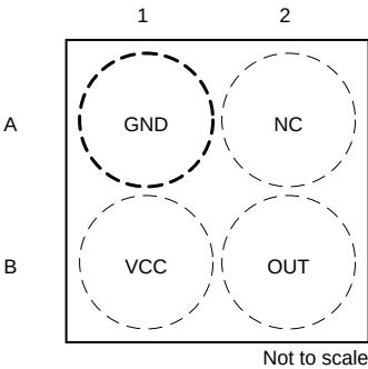
图 5-1. YBK 和 YBH 封装 4 引脚 DSBGA (全极) 顶视图
