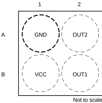
图 5-2. YBK 和 YBH 封装 4 引脚 DSBGA (双路单极) 顶视图
