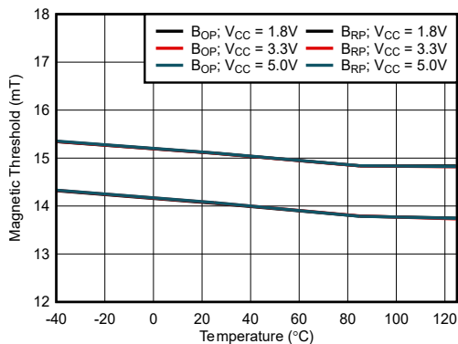
图 6-7. 15mT B OP 、14.1mT B RP ：阈值与温度间的关系
