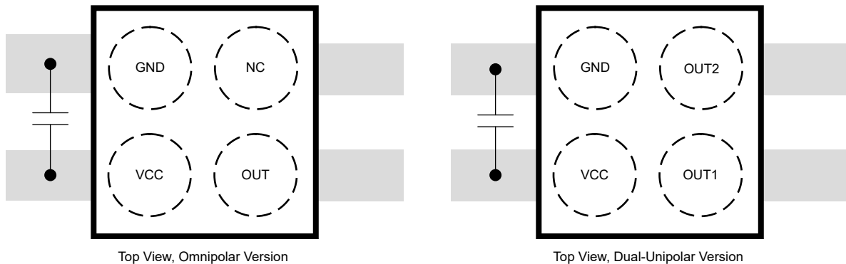
图 8-3. DSBGA 布局示例
