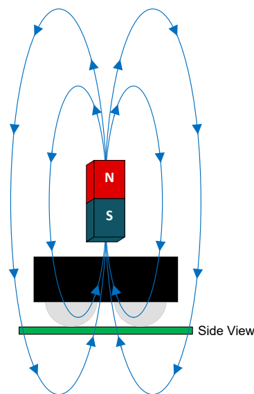
图 7-4. 正磁通密度：磁体对齐
