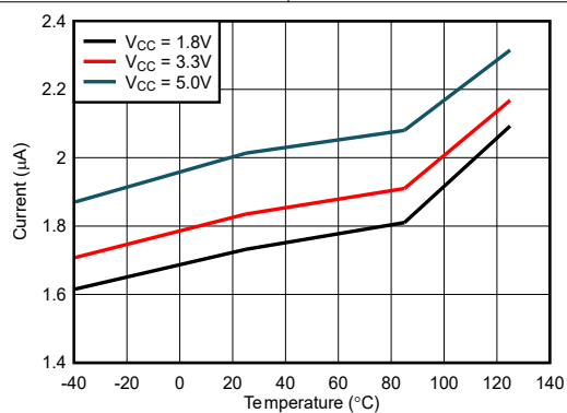
图 6-8. 20Hz I CAVG 与温度之间的关系
