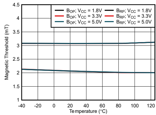
图 6-2. 3mT B_{OP} 、2.1mT B_{RP} : 阈值与温度间的关系
