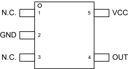
图 5-3. DBV 封装 5 引脚顶视图
