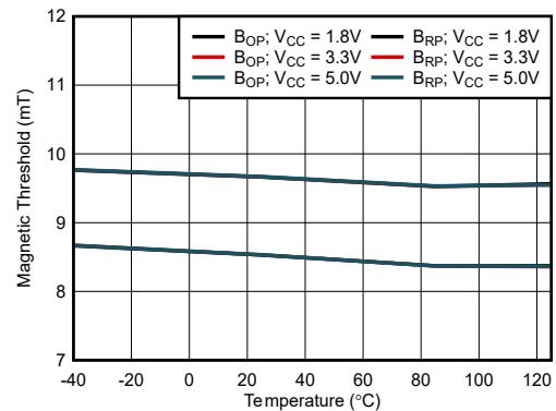
图 6-6. 9.5mT B_{OP} : 阈值与温度间的关系
