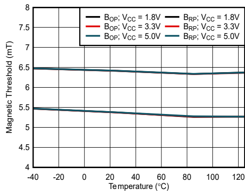
图 6-5. 6.3mT B_{OP} : 阈值与温度间的关系
