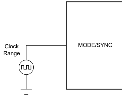
图 6-3. 允许使用 MODE/SYNC 引脚实现同步的典型实现方案
