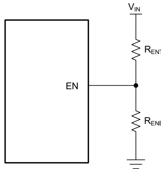
图 6-2. 使用 EN 引脚时的 V_{IN} UVLO
