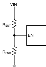
图 7-2. 外部 UVLO 应用的设置
