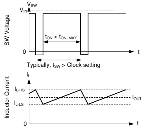
图 6-8. 电流限值波形
