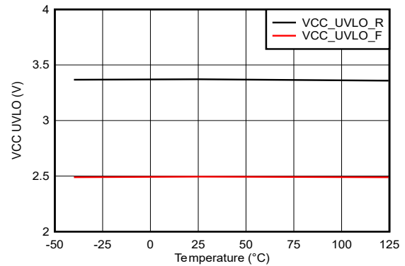
图 5-4. V CC UVLO
