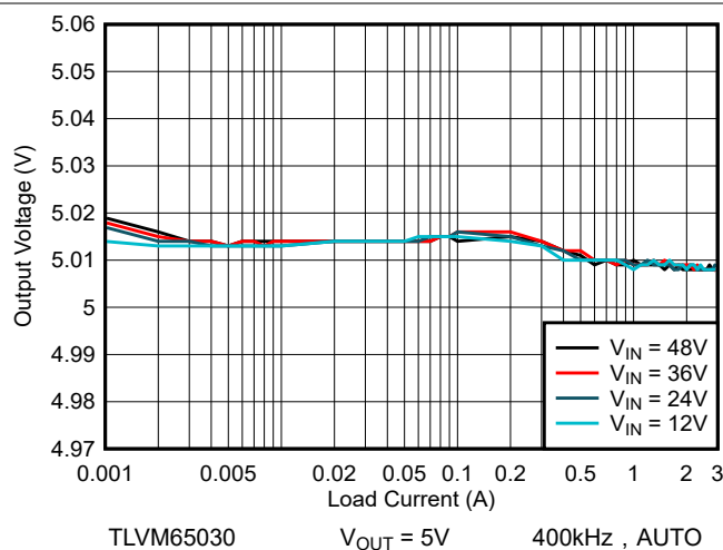
图 7-5. 线性 and 负载调整率
