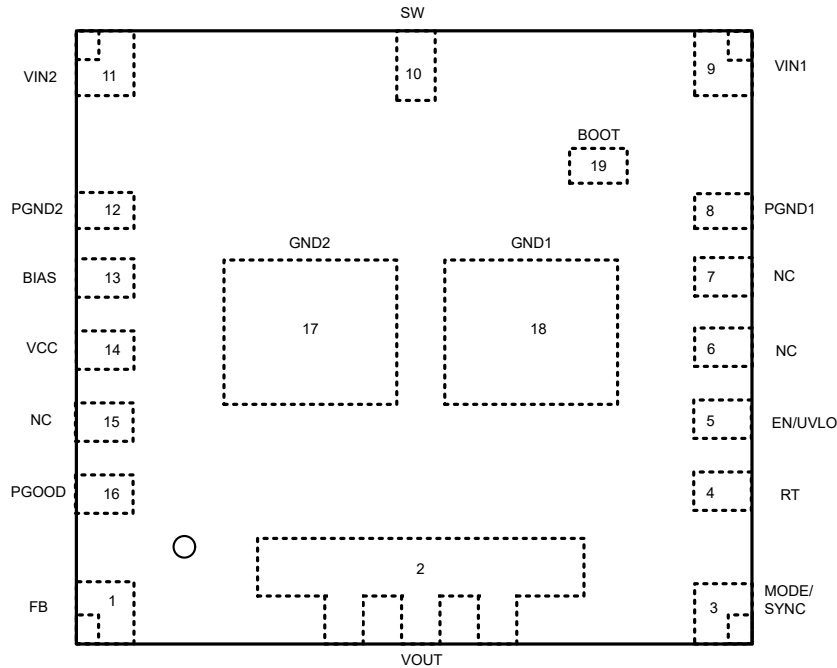
图 4-1. 19 引脚 VCG、QFN-FCMOD 封装 ( 顶视图 )
