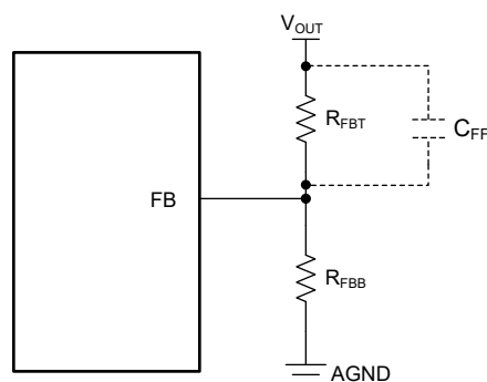
图 6-1. 设置可调版本的输出电压
