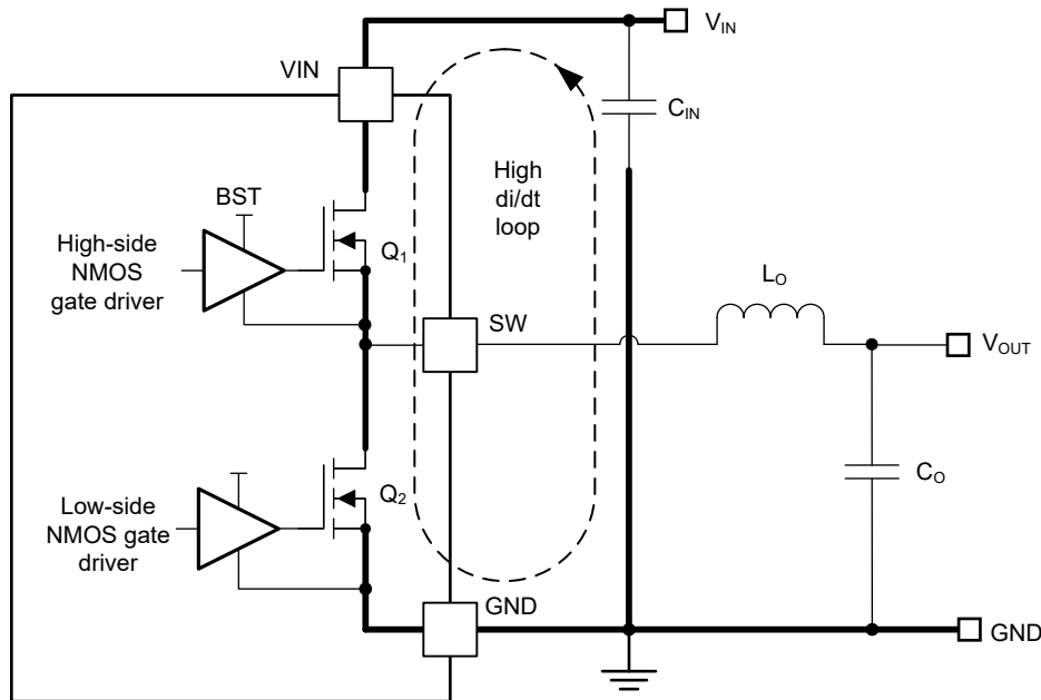
图 7-18. 具有快速边沿的电流环路
