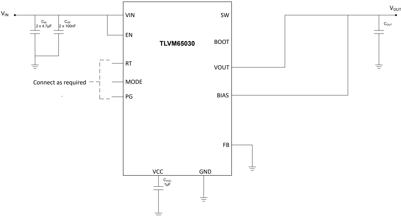
图 7-1. 采用 TLVM65030 的固定输出电压模式示例应用电路
