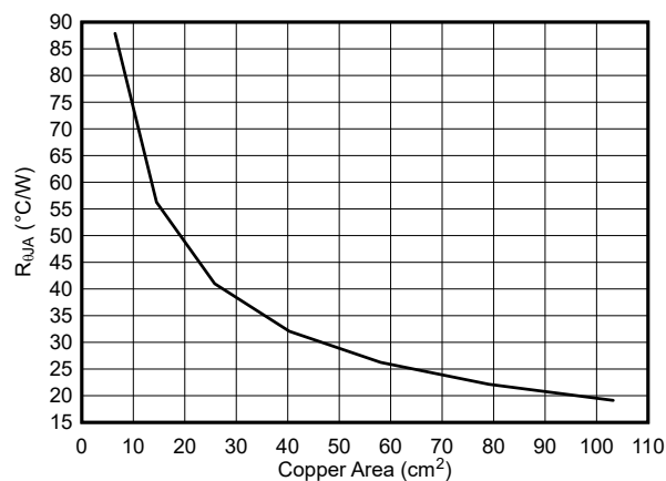
图 7-3. 热阻与铜面积之间的关系
