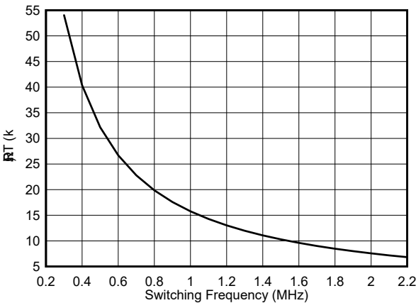
图 6-6. 开关频率与 RT 间的关系
