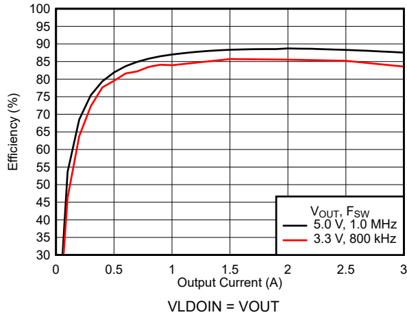
图 6-18. 效率
