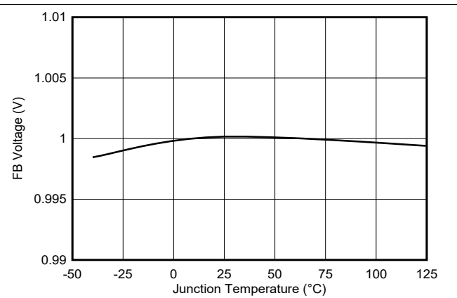
图 6-2. 反馈电压
