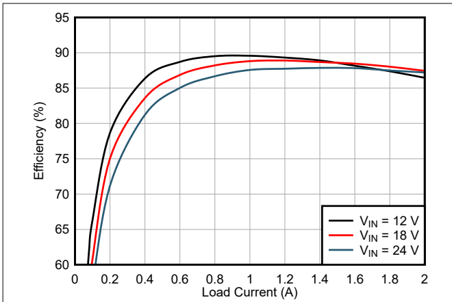
图 8-13. 效率曲线
