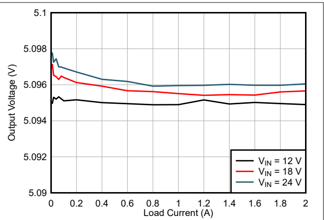
图 8-14. 负载调整率
