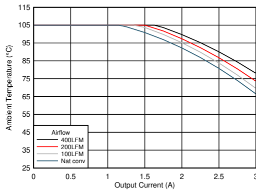
图 6-22. 安全工作区 V_{OUT} = 5.0V, F_{sw} = 1MHz
