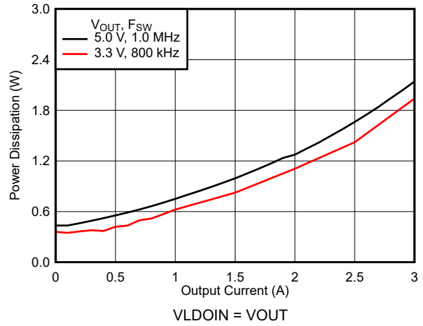
图 6-19. 功率耗散
