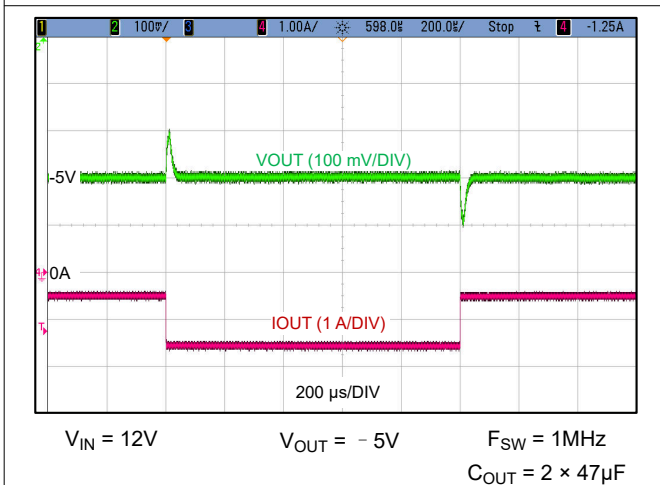
图 8-15. 负载瞬态 ( -0.5A 至 -1.5A , 1A/ \mu s )
