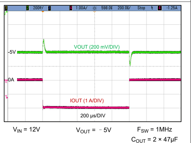
图 8-16. 负载瞬态 ( 0A 至 -2A , 1A/ \mu s )
