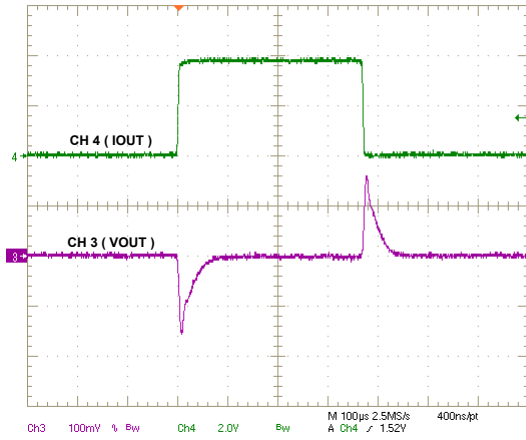
图 9-8. 瞬态负载，在 1\text{ A}/\mu s 下为 0A 至 4A
