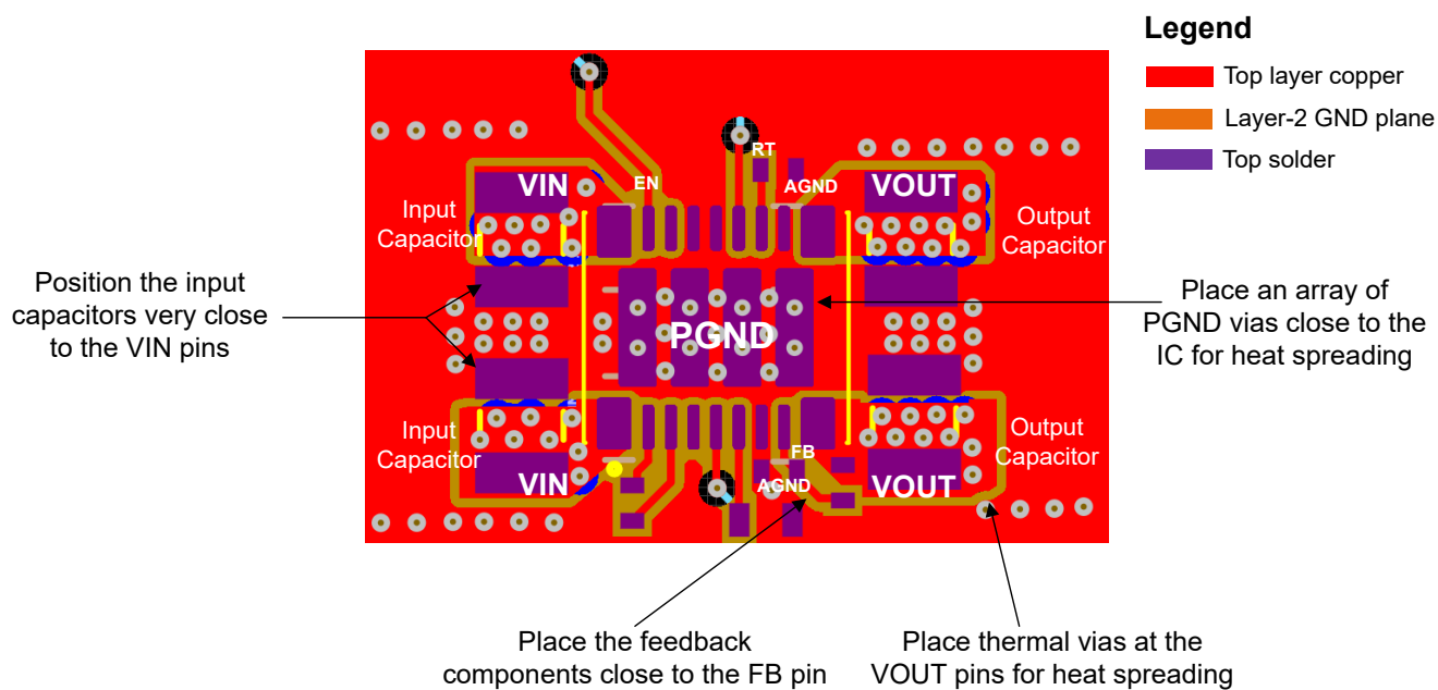
图 9-13. 典型顶层设计
