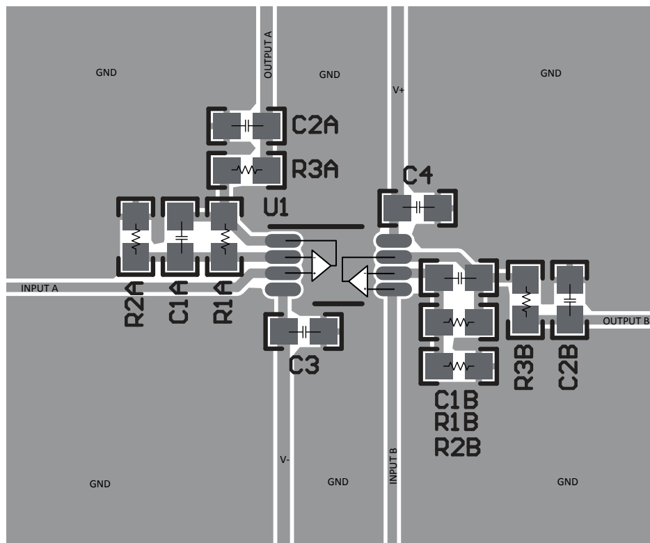
图 10-4. VSSOP-8 (DGK) 封装的示例布局
