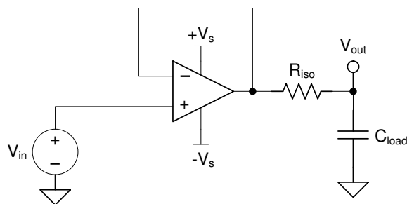
图 7-8. 使用 TLV9301 扩展容性负载驱动
