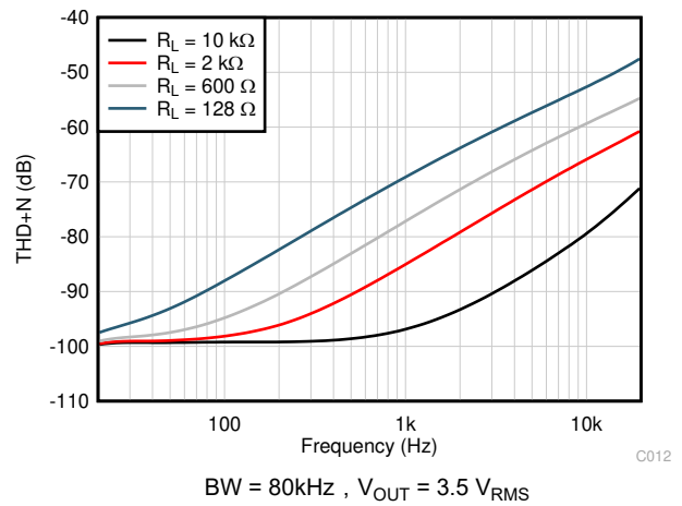
图 6-20. THD+N 比与频率间的关系
