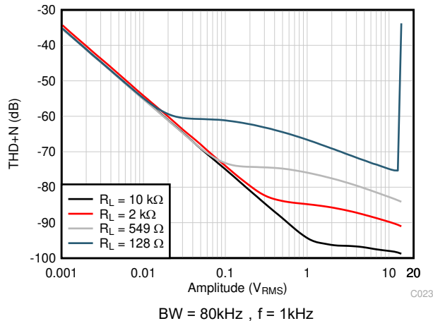
图 6-21. THD+N 与输出幅度间的关系
