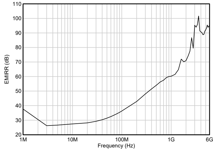
图 6-4. EMIRR 测试
