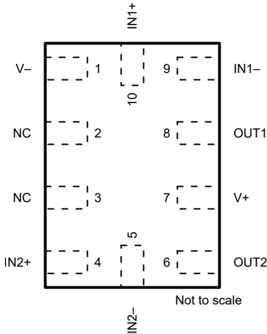
图 4-5. TLV9142 RUG 封装， 10 引脚 X2QFN (顶视图)
