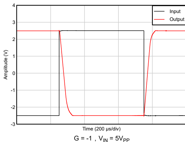
图 5-43. 大信号阶跃响应
