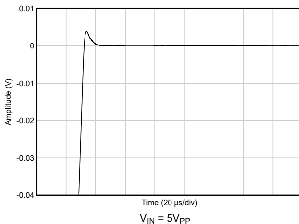
图 5-44. 稳定时间 (正)
