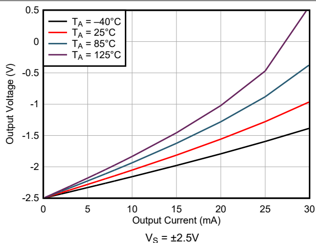
图 5-26. 输出电压摆幅与输出电流 (灌电流) 间的关系
