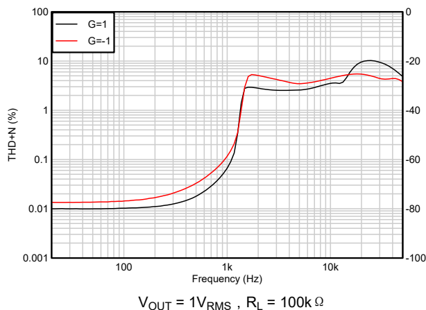
图 5-9. THD+N 与频率间的关系
