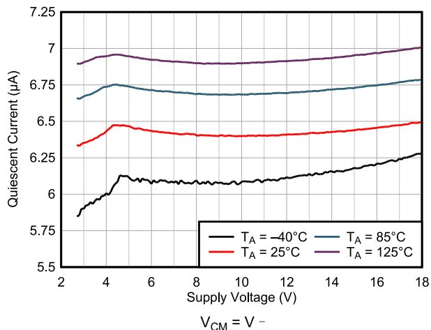
图 5-30. 静态电流与电源电压间的关系
