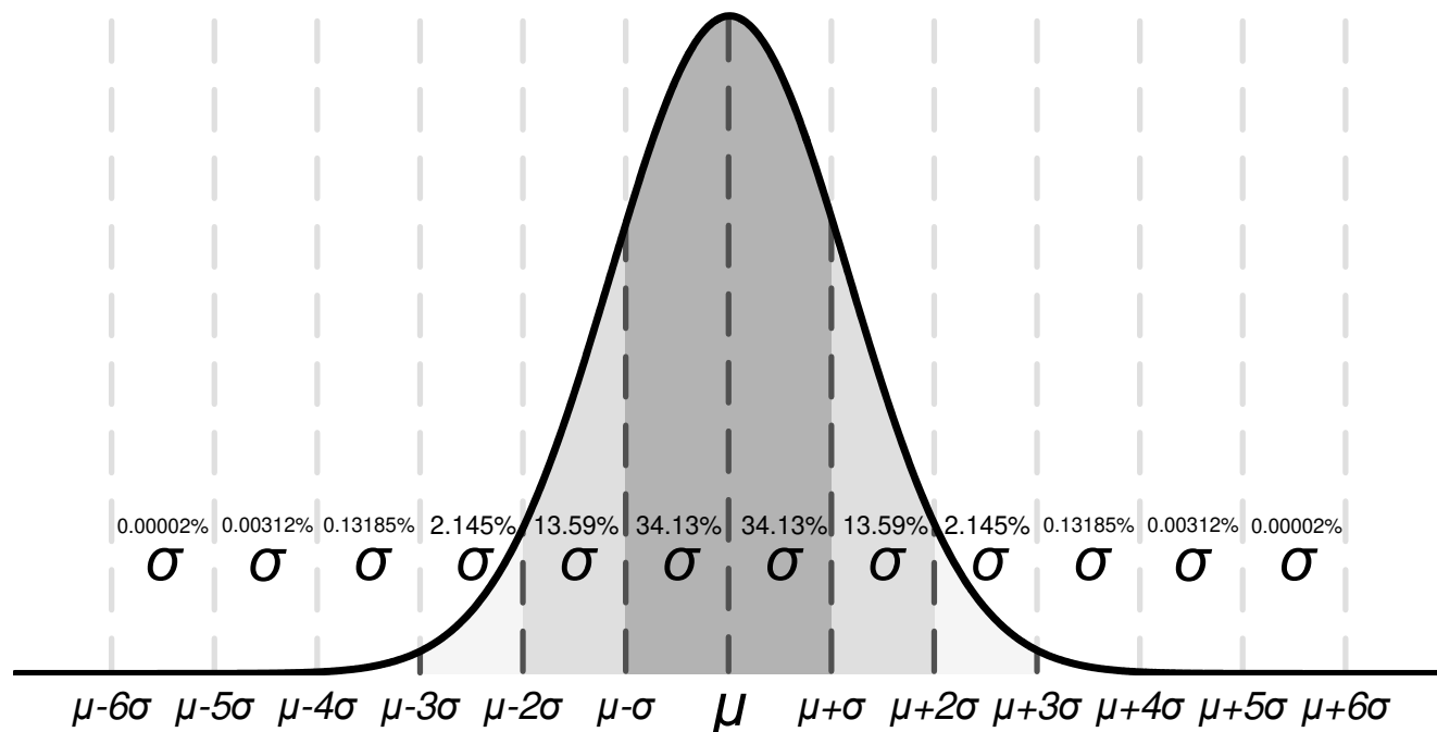
图 6-7. 高斯分布
