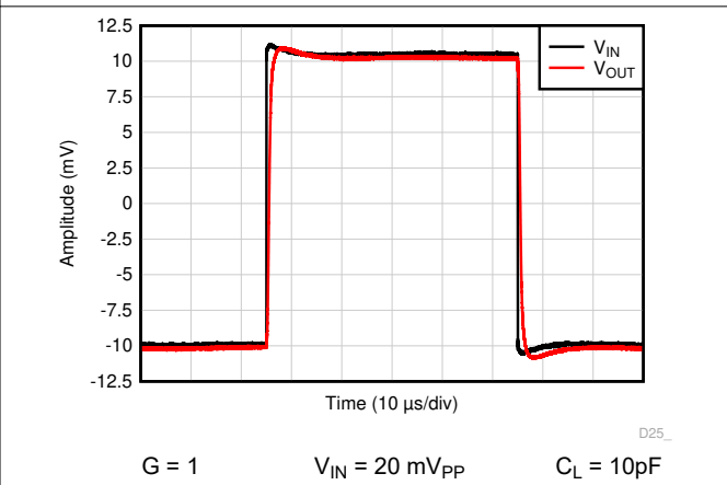
图 6-34. 小信号阶跃响应
