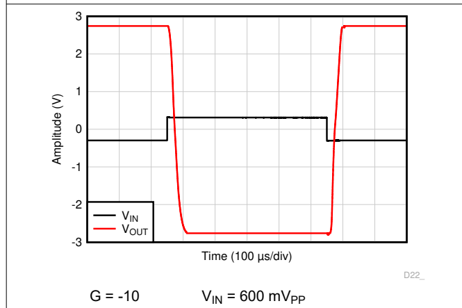
图 6-33. 过载恢复
