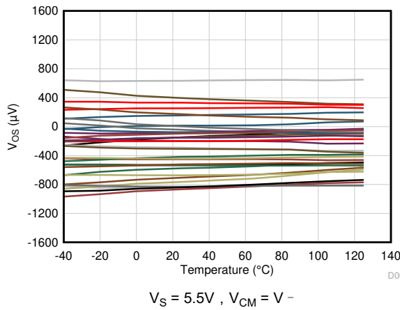
图 6-3. 输入失调电压与温度间的关系
