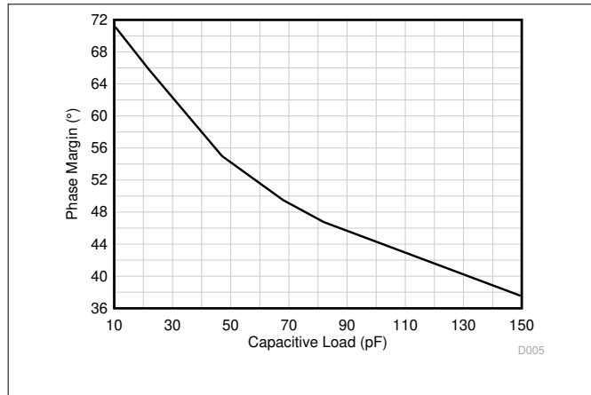
图 6-31. 相位裕度与容性负载间的关系
