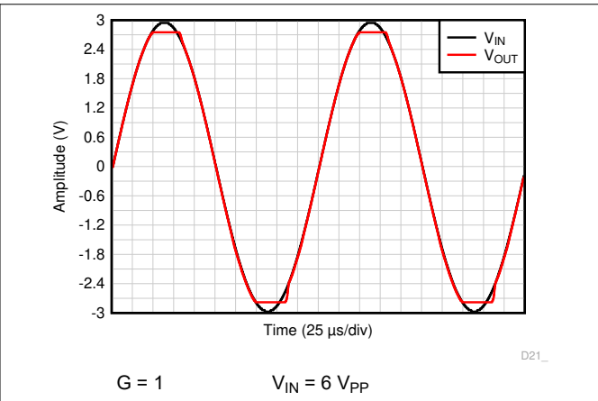
图 6-32. 无相位反转
