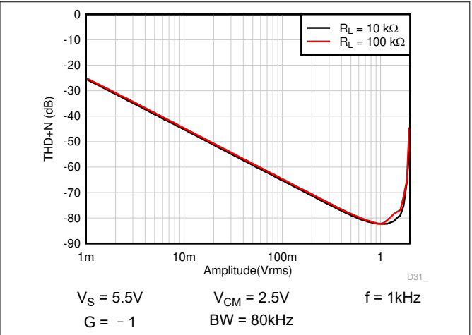
图 6-26. THD + N 与幅度间的关系
