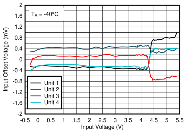
图 5-28. -40^\circ\text{C} 时失调电压与输入电压间的关系, 5V
