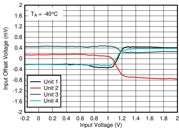
图 5-27. -40^\circ\text{C} 时失调电压与输入电压间的关系, 1.8V
