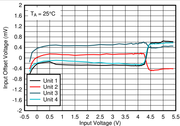
图 5-26. 25^\circ\text{C} 时失调电压与输入电压间的关系, 5V
