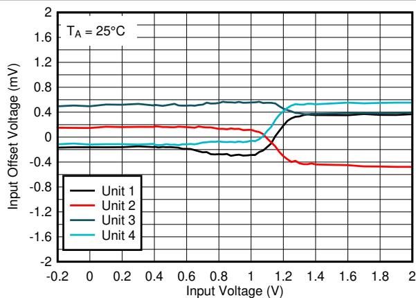
图 5-25. 25^\circ\text{C} 时失调电压与输入电压间的关系, 1.8V
