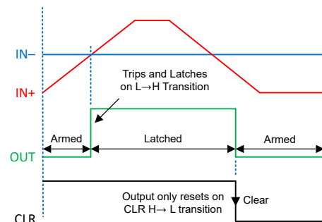
TLV903xL 推挽门锁响应
