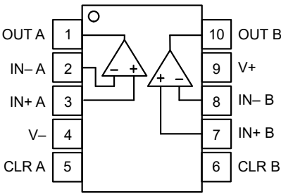
DGS 封装 10 引脚 VSSOP 俯视图
