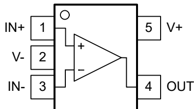
图 4-1. TLV9020-Q1、TLV9030-Q1 DCK 和 DBV 封装 标准“东南”引脚排列 5 引脚 SC-70 和 SOT-23 顶视图
