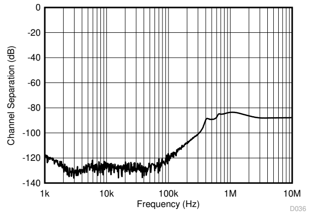
图 6-36. 通道隔离
