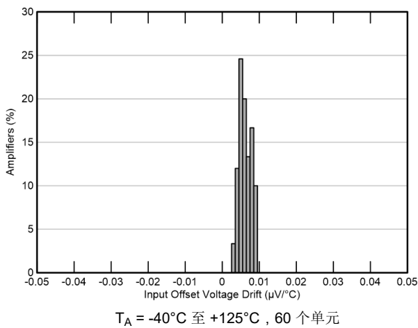
图 5-3. 偏移电压漂移
