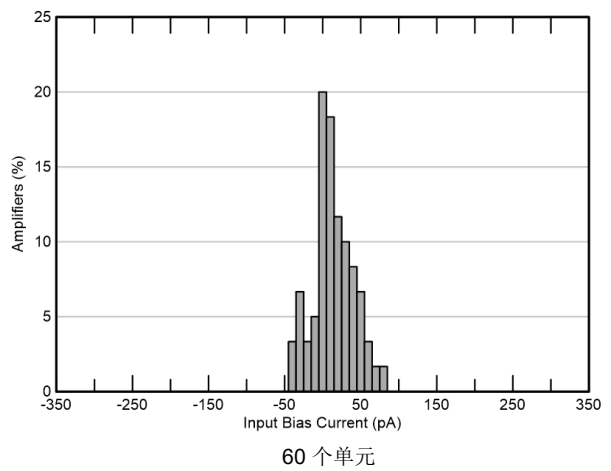
图 5-4. 输入偏置电流分布， I_{BN}
