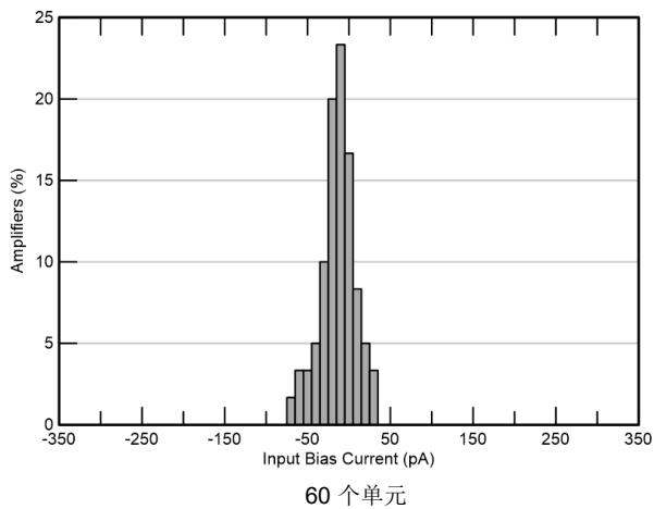
图 5-5. 输入偏置电流分布， I_{BP}
