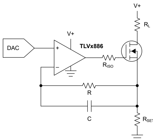
图 7-7. 可编程精密电流源
