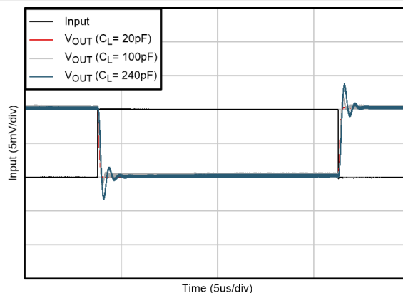
图 5-32. 负过载恢复
