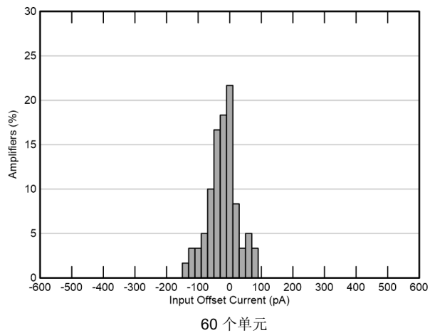
图 5-6. 输入偏移电流分配
