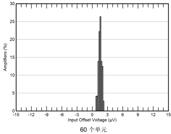
图 5-1. 失调电压分布图
