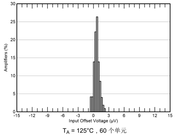
图 5-2. 失调电压分布图
