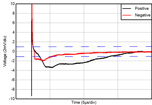
图 5-38. 趋稳时间
