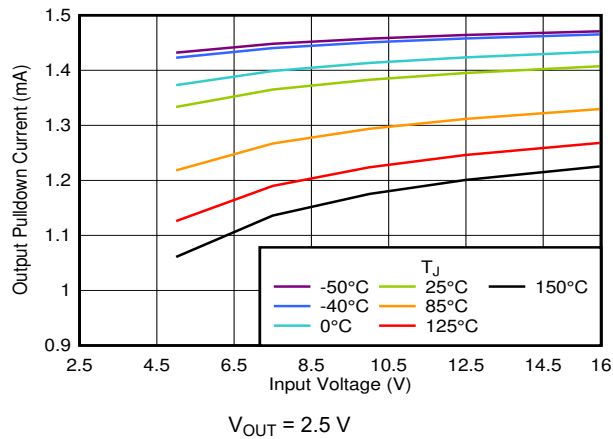
图 6-31. I_{PULLDOWN} vs V_{IN}
