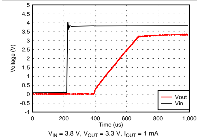
图 23. V_{IN} Power-Up
