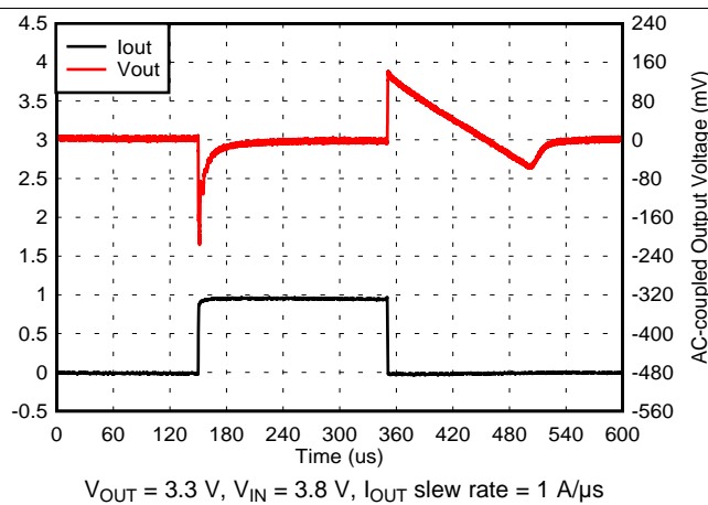
图 22. 1-mA to 1-A Load Transient (3.3 V)
