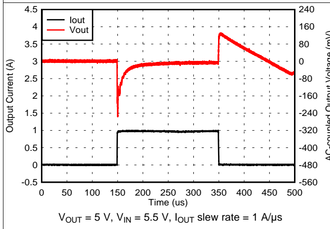
图 21. 1-mA to 1-A Load Transient (5 V)
