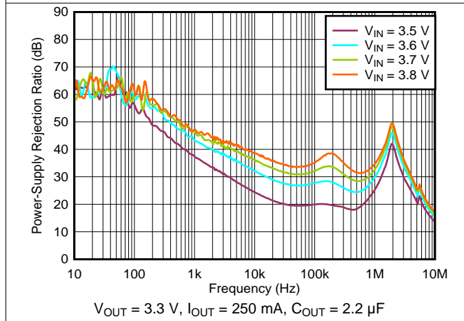
图 27. PSRR vs Frequency and V_{IN}
