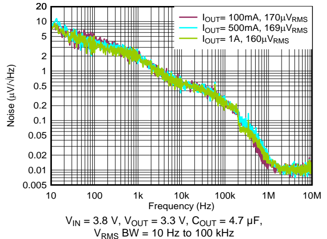
图 34. Output Spectral Noise Density
