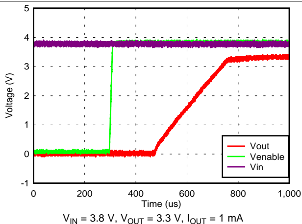
图 24. Startup With EN
