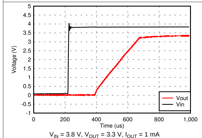
图 23. V_{IN} Power-Up
