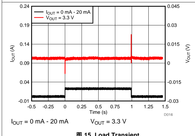
图 15. Load Transient
