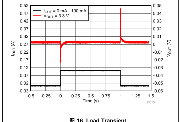
图 16. Load Transient
