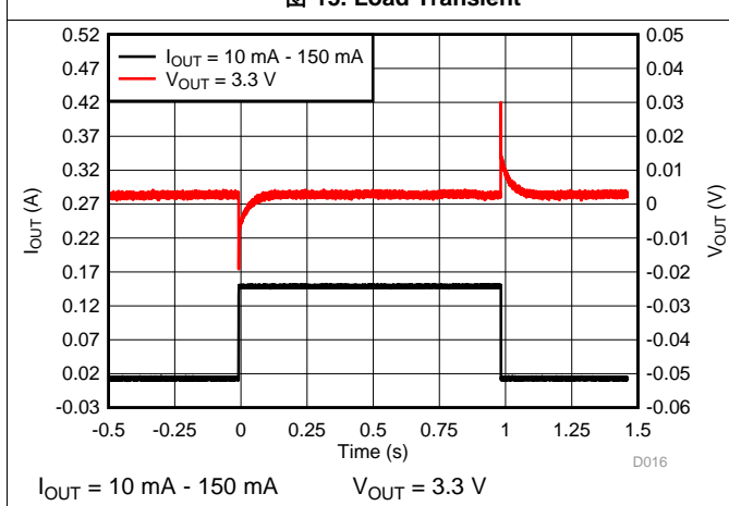
图 17. Load Transient
