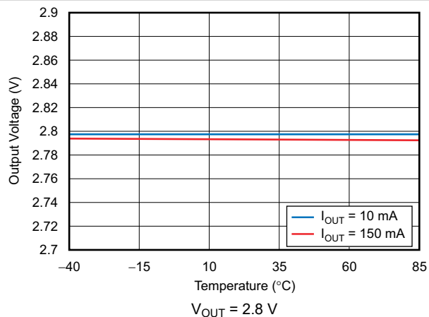
图 6-11. Output Voltage vs Temperature
