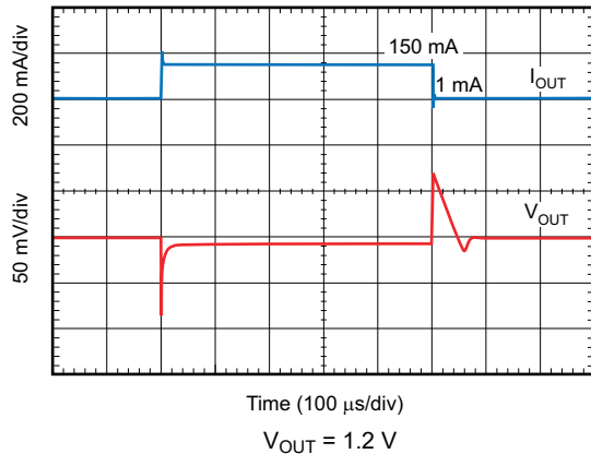
图 8-4. Load Transient Response
