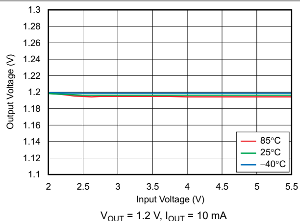
图 6-4. Line Regulation
