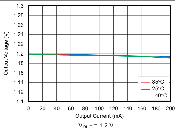
图 6-1. Load Regulation
