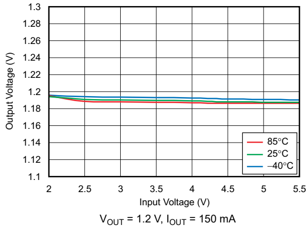
图 6-7. Line Regulation
