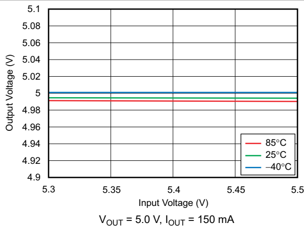
图 6-9. Line Regulation
