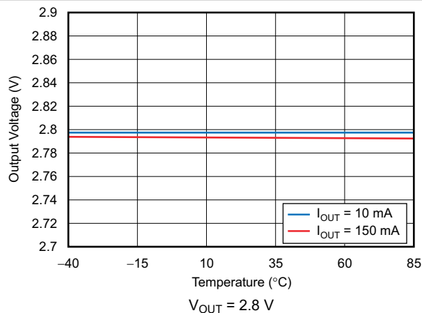
图 6-11. Output Voltage vs Temperature
