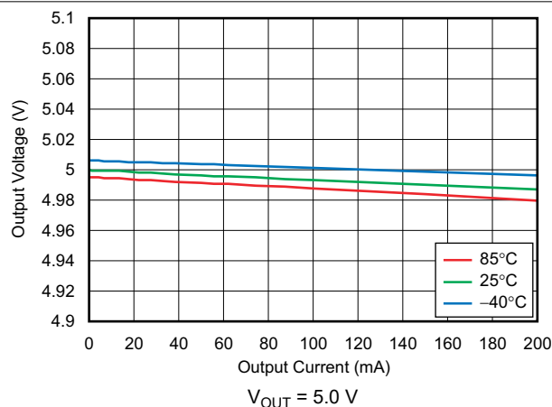
图 6-3. Load Regulation
