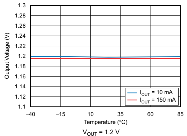
图 6-10. Output Voltage vs Temperature
