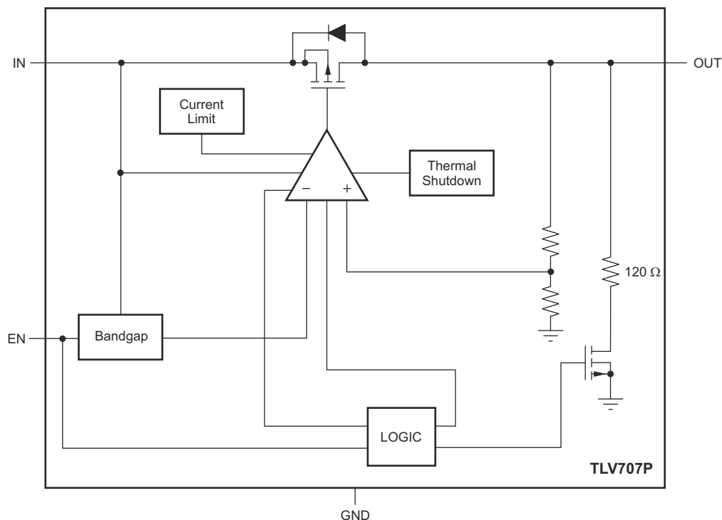
图 7-2. TLV707P Block Diagram
