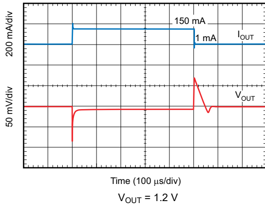
图 8-4. Load Transient Response
