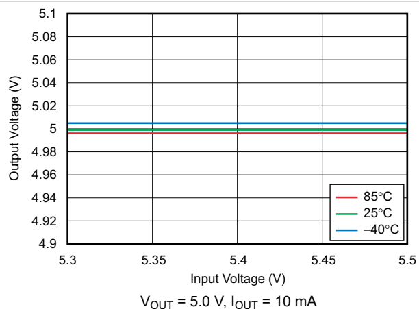
图 6-6. Line Regulation
