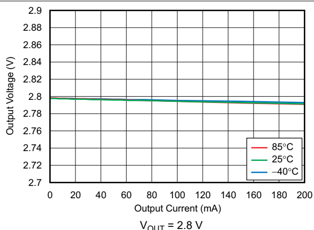
图 6-2. Load Regulation
