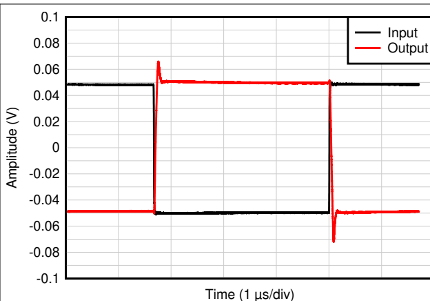
图 7-64. 小信号阶跃响应
