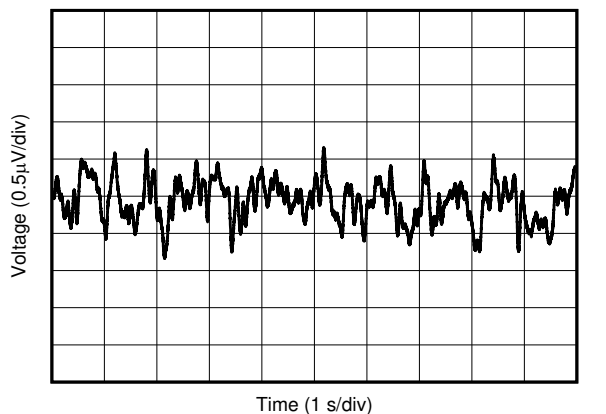
图 7-15. 0.1Hz 至 10Hz 闪烁噪声
