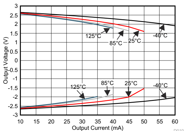
图 7-11. V_O 与 I_O 拉电流和灌电流间的关系
