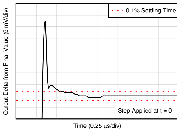
图 7-66. 大信号阶跃响应
