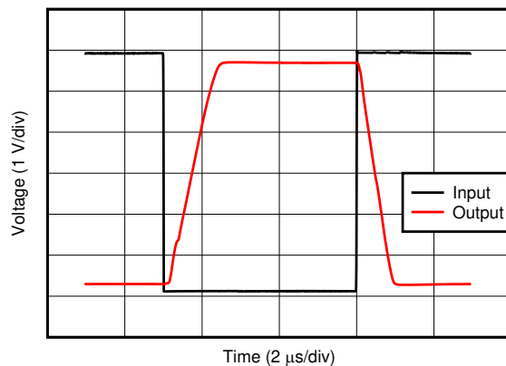
图 7-30. 过载恢复
