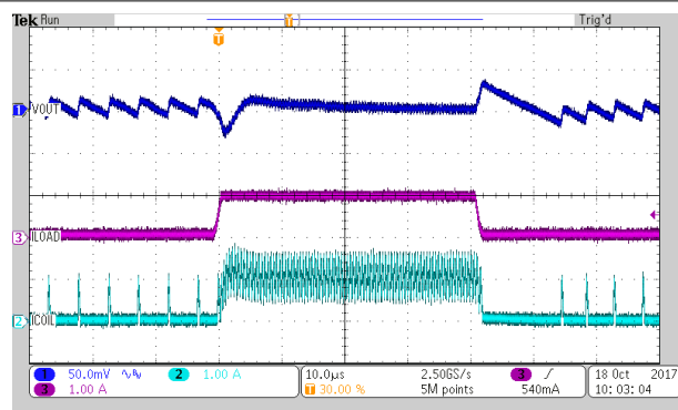
图 8-24. Load Transient
