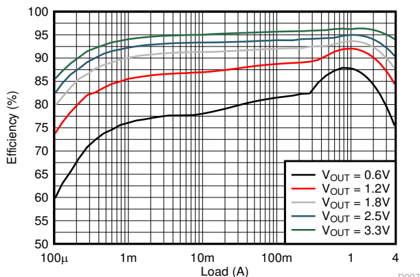
V_{IN} = 5V 时的效率
