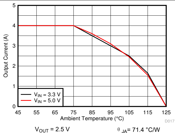
图 8-16. Thermal Derating
