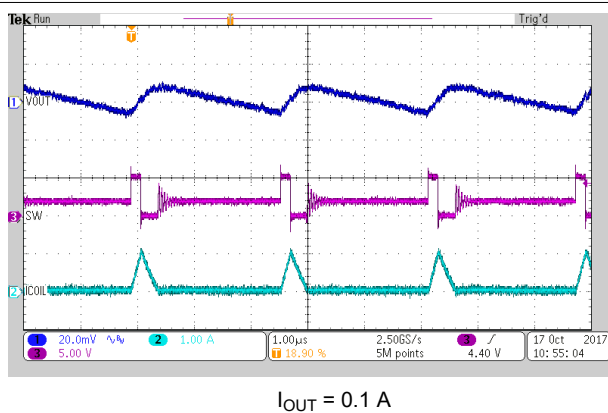
图 8-19. PSM Operation
