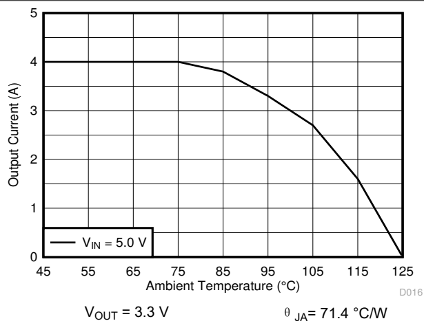
图 8-17. Thermal Derating
