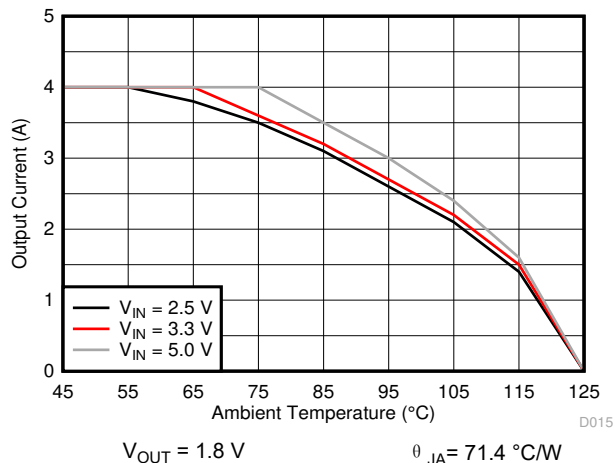
图 8-15. Thermal Derating
