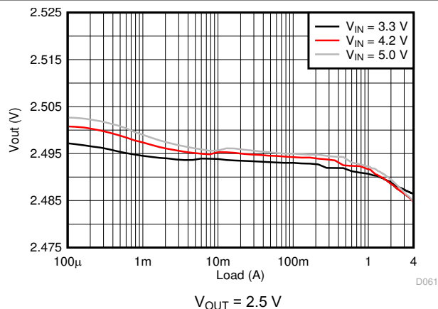
图 8-9. Load Regulation
