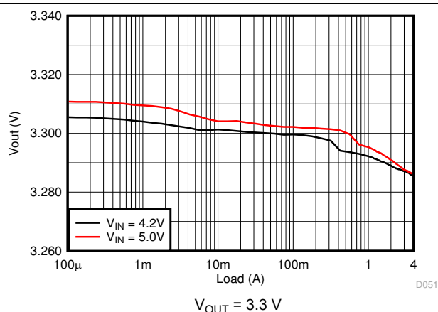
图 8-11. Load Regulation
