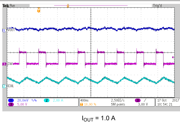
图 8-18. PWM Operation
