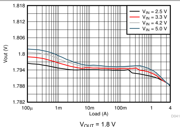
图 8-7. Load Regulation
