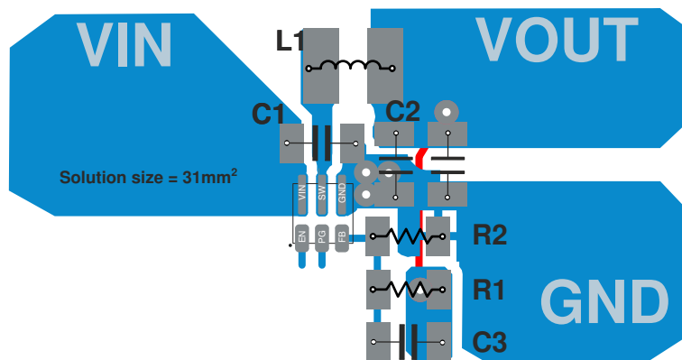
图 8-28. PCB Layout Recommendation
