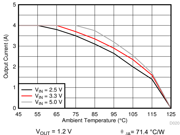
图 8-14. Thermal Derating
