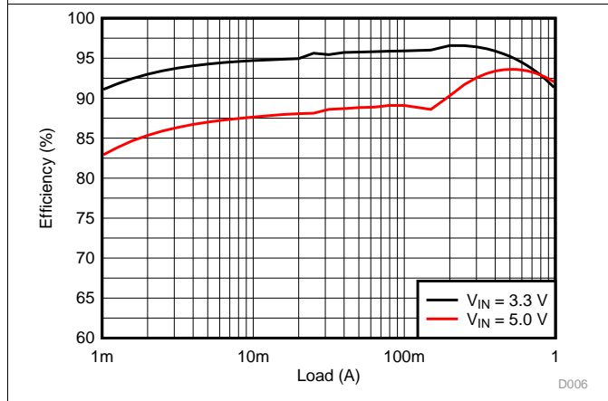
图 8. 2.5-V Output Efficiency
