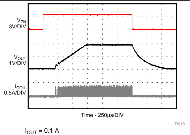
图 17. Startup with Load
