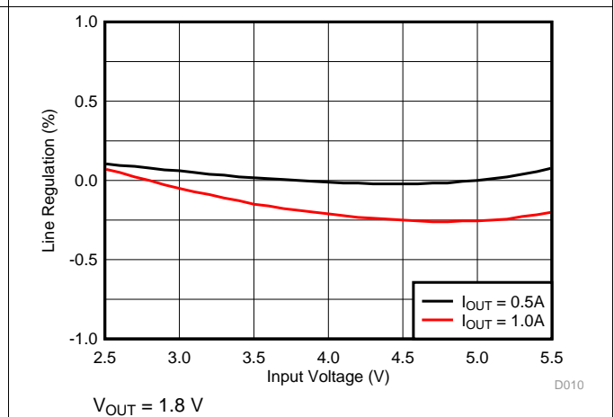
图 11. Line Regulation
