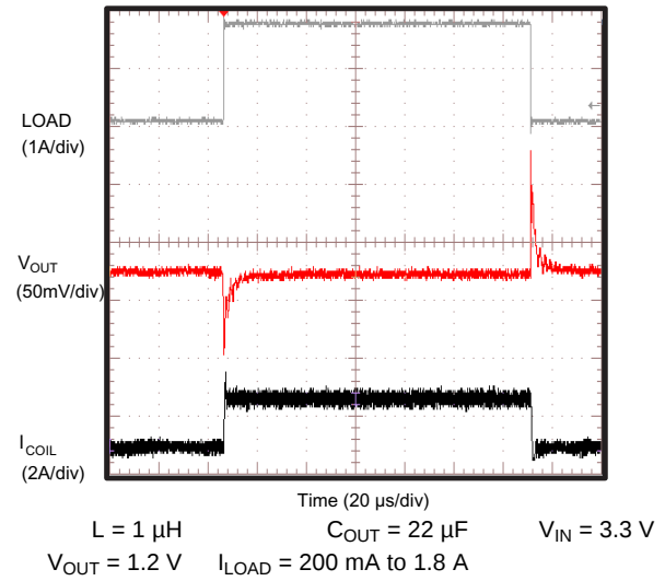
图 14. Load Transient
