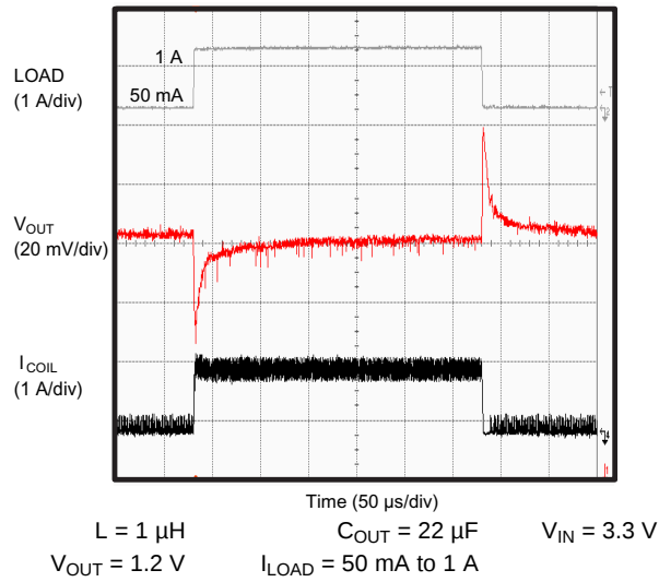
图 13. Load Transient
