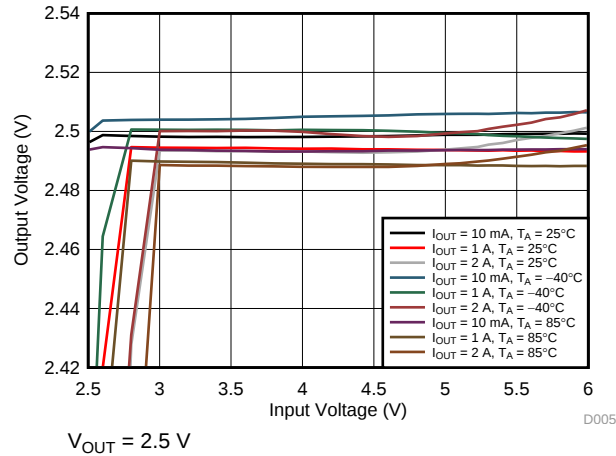
图 5. Output Voltage vs Input Voltage
