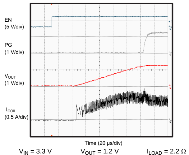
图 16. Startup
