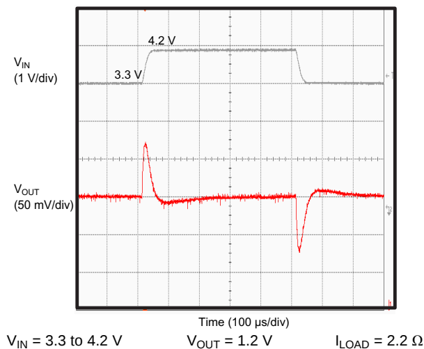
图 15. Line Transient
