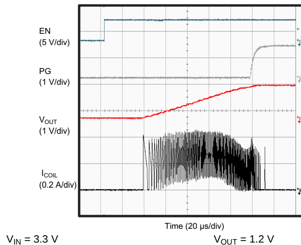
图 17. Startup (No Load)
