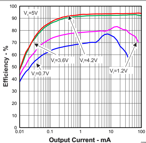
图 6-6. 效率与输入电压和输出电流的关系
