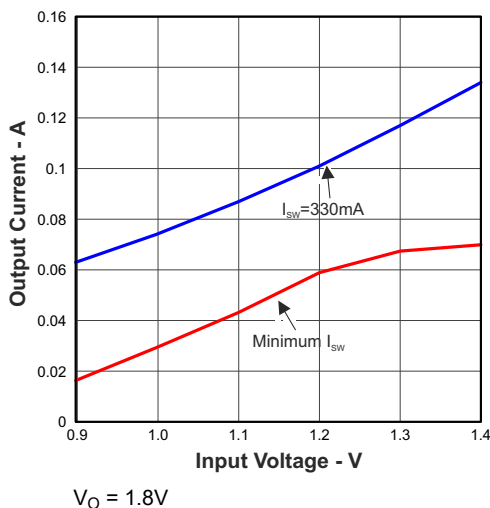
图 6-1. 最大输出电流与输入电压间的关系
