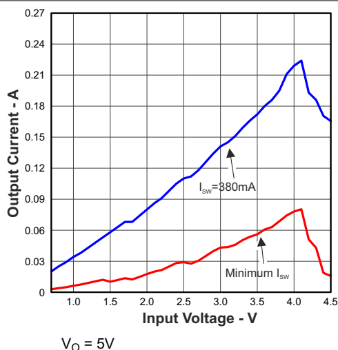
图 6-3. 最大输出电流与输入电压间的关系
