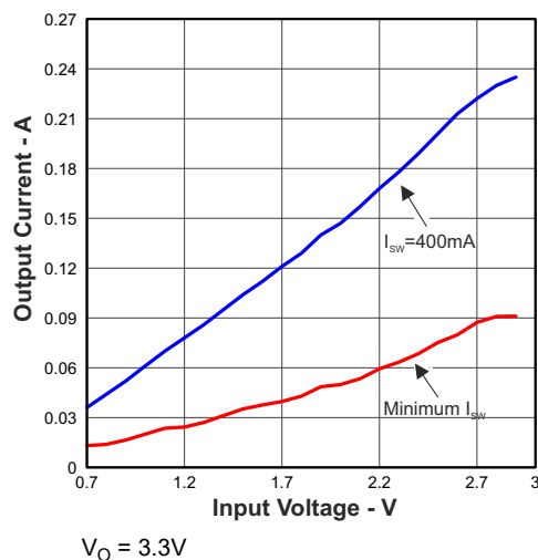
图 6-2. 最大输出电流与输入电压间的关系
