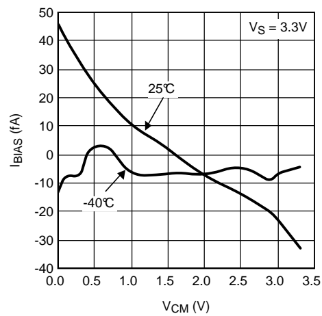
图 16. 输入偏置电流与共模电压间的关系
