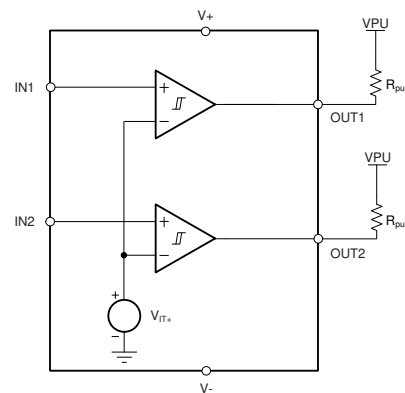
TLV4082-Q1 方框图
