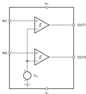
TLV4062-Q1 方框图
